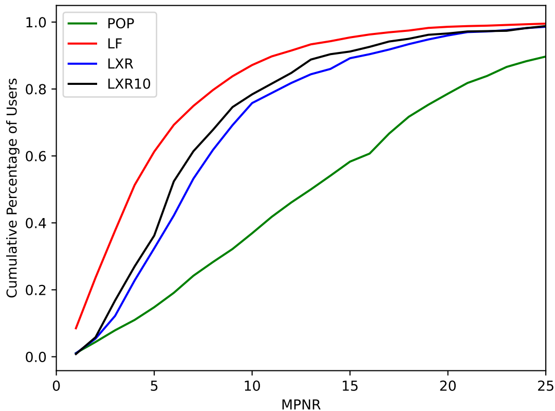
Recommender:VAE, Dataset:Pinterest
