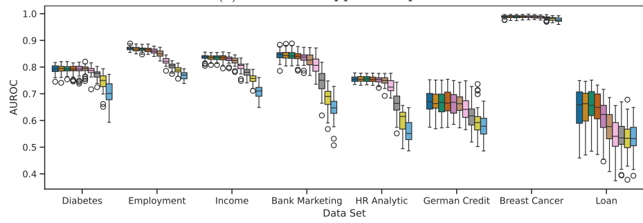
(b) AUROC
