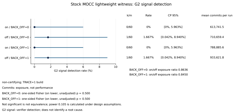
図 5 stock MOCC の軽量 witness 4 arm (各 60 走) の G2 signal 検出率 (点 = k/m , 横線 = Clopper-Pearson (CP) 両側 95% 区間) と, 走あたり commit 数の平均 (記述). witness on は BACK_OFF=0 / 1 とともに 0/60 (0%, CP [0%, 5.963%]), off は両方とも 1/60 (1.667%, CP [0.042%, 8.940%]). 片側 Fisher 検定 (on が低い方向, 未調整) は BACK_OFF=0 (主比較)・1 とともに p = 0.500 , on/off の曝露比は 0.8636 / 0.8450 である. 非有意は同等性を示さず, 0 件は不在を示さない. 検出力 0.105 は設計仮定 (独立 Bernoulli 試行, arm あたり 60 走, off の確率 0.0417, on の確率 0, \alpha 0.05 の片側 Fisher) の下の計算値で, 実測量ではない. TRACE=1 ビルドの commit 数は曝露量であって性能ではなく, 検出率は 3 秒の固定時間の走あたりの率で, 等しい commit 曝露での比較ではない. G2 signal は根因を同定せず, 実 anomaly と torn read も区別しない (on の signal が無く識別器は一度も発火していない). 非 certifying の観測であり, 個々の判定器の certified 表示や arm の属性は, この観測・MOCC・witness を認証しない. 分母は 4 ブロック \times 15 ラウンド \times 4 arm だけで, smoke 走は除く. CP 区間と Fisher の p は独立な Bernoulli 試行を仮定し, ノード内相関・回転順・時間変動をモデル化していない. 過去の観測の値とは合算も比較もしない. 条件: 48 スレッド, 10,000 レコード, Zipf 0.9, read 比率 50, rmw 0, max operations 10, 3 秒, TRACE=1 ビルド, 固定版 + X/P・軽量 witness の patch, Pegasus 計算ノード.
