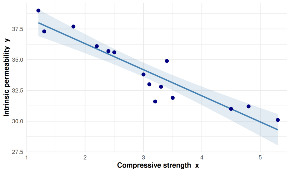
Figure 1: Ex 6-5 散佈圖與最小平方回歸線 (含 95% 平均反應信賴帶)。X 軸為 compressive strength x 、Y 軸為 intrinsic permeability y ；負斜率對應 \beta_1 = -2.123 。
