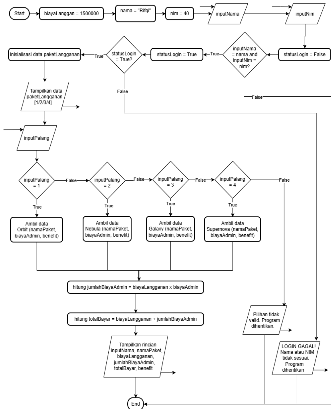
Gambar 1.1 Flowchart Program Paket Langganan ANGKASA pada Draw.io
