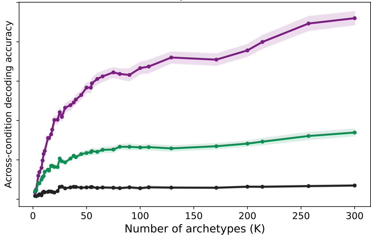
Temporal AA
