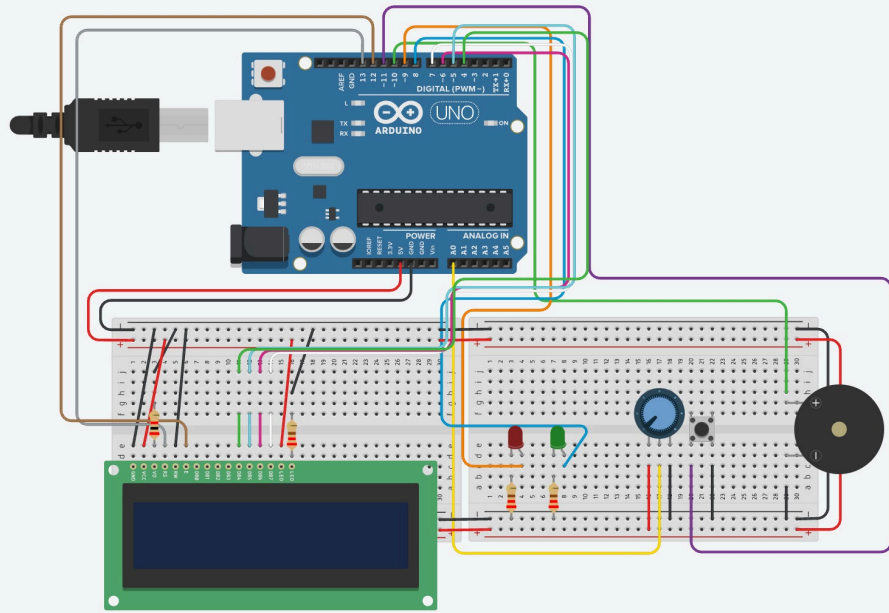
Captura del circuito armado en Tinkercad
