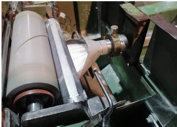
Anexo 09: Bandejas y Embudos de Máquina Integradas.
