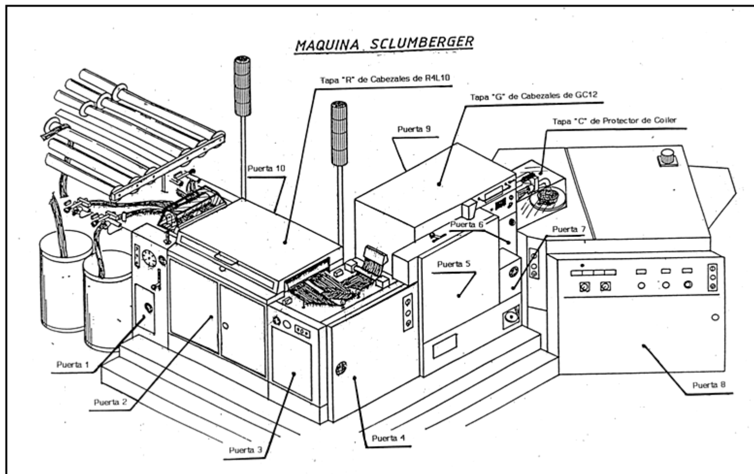
FIGURA 2 DESCRIPCIÓN DE PUERTAS – MAQUINA INTEGRADA (SCHLUMBERGER R4L10 / GC12 )
