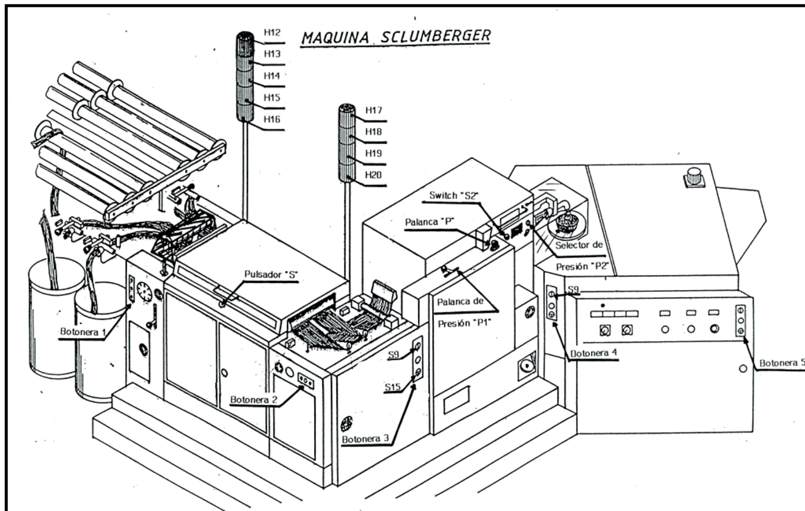
FIGURA 1 DESCRIPCION DE LUCES Y BOTONERAS – MAQUINA INTEGRADA (SCHLUMBERGER R4L10 / GC12)
