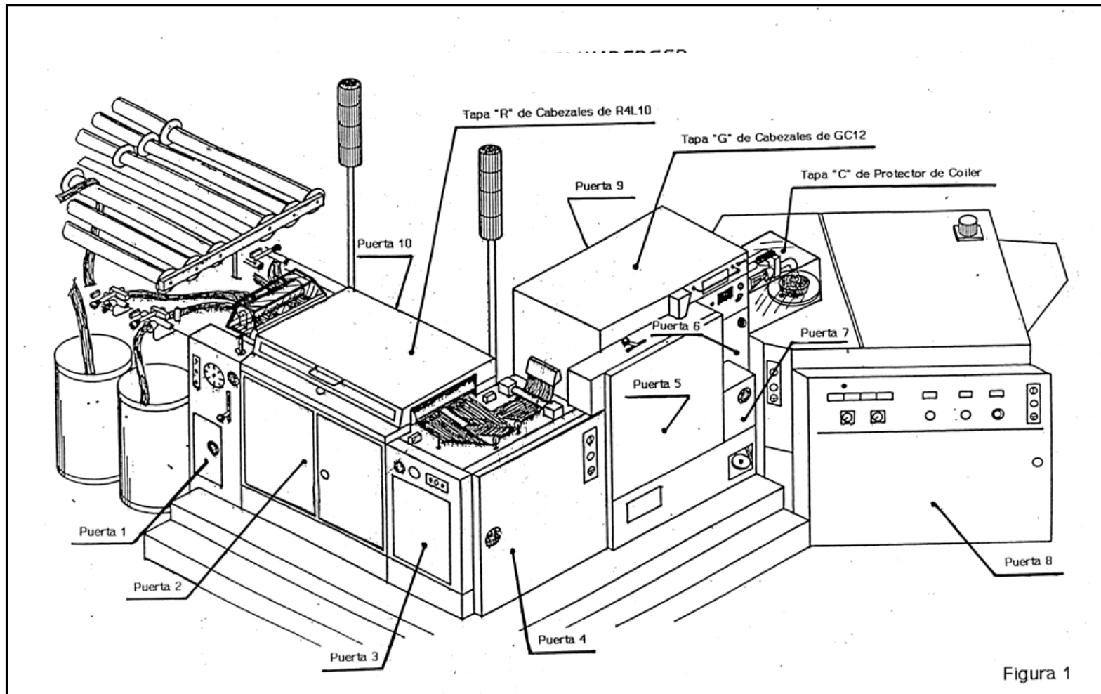
FIGURA 1: DESCRIPCIÓN DE PUERTAS - MÁQUINA INTEGRADA (SCHLUMBERGER)
