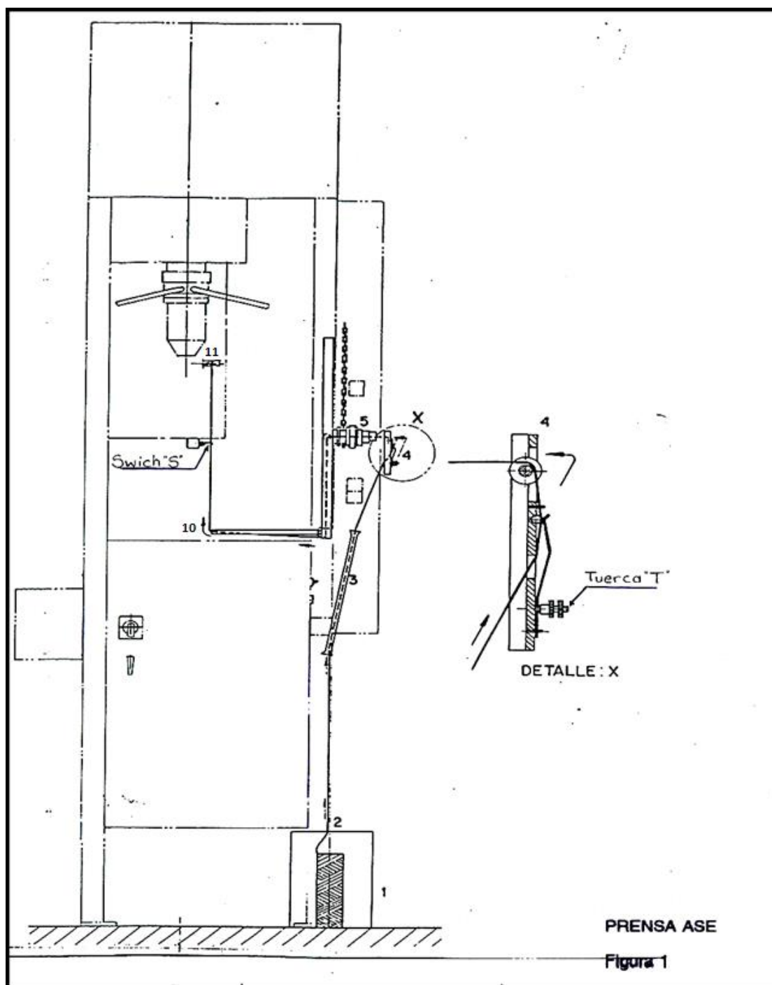
Figura 1. PRENSA ASE
