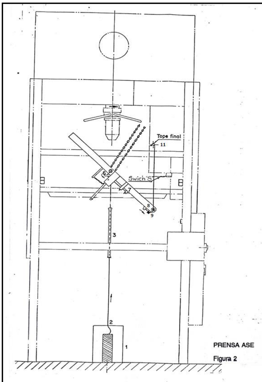
Figura 2. PRENSA ASE
