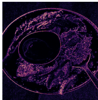
|\nabla^2 I_{clear}|
