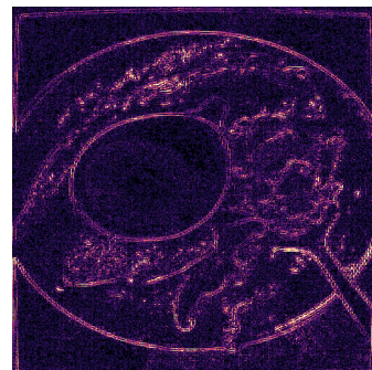
|\nabla^2 I_{fog}|
