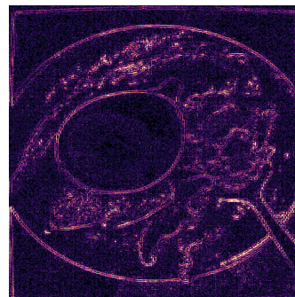
|\nabla^2 I_{fog}|
