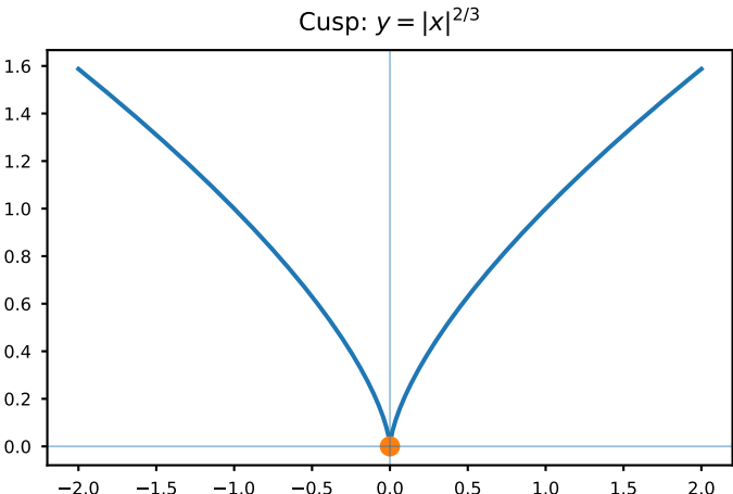
Fig. 7. Cusp
