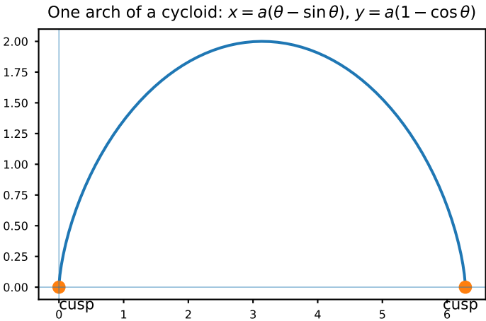
Fig. 31. Cycloid
