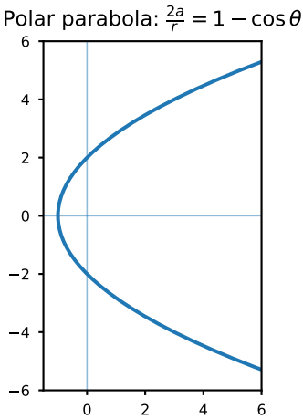
Fig. 27. Polar parabola
