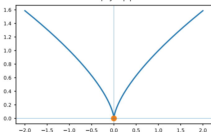
Fig. 7. Cusp
