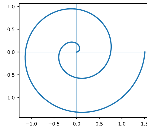
Fig. 24. Archimedean spiral
