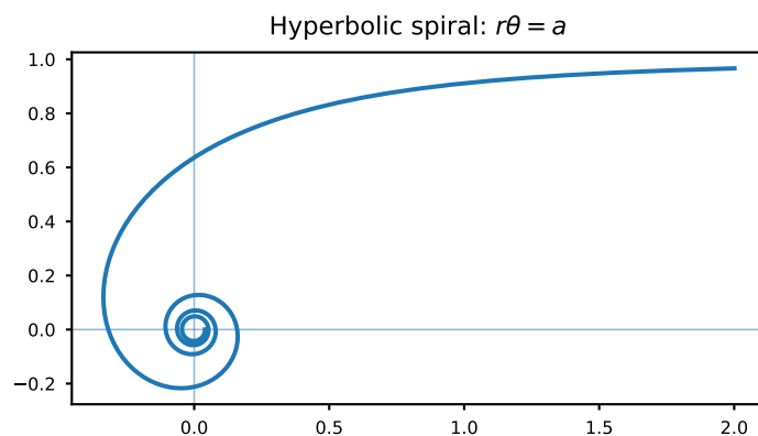
Fig. 26. Hyperbolic spiral
