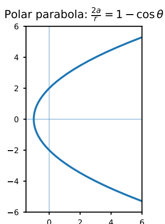
Fig. 27. Polar parabola
