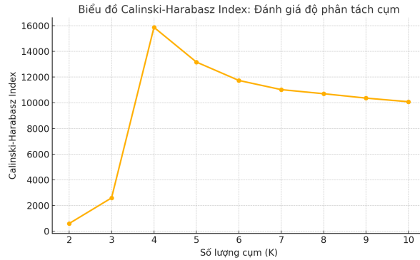
Hình 13: Calinski–Harabasz
