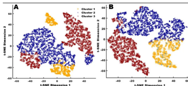
Hình 17: t-SNE
