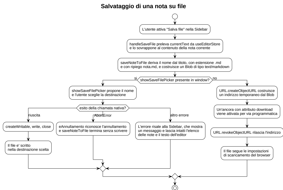
Figura 23: Diagramma UML 4.4.1-2 - Salvataggio di una nota su file
