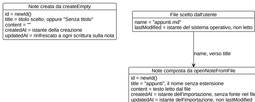
Figura 28: Diagramma UML 4.4.3 - Provenienza dei metadati per una nota creata nel prodotto e per una importata da file
