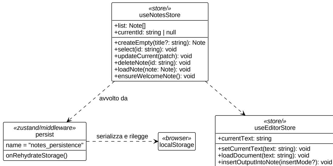
Figura 25: Diagramma UML 4.4.2-1 - La catena di persistenza dello store delle note
