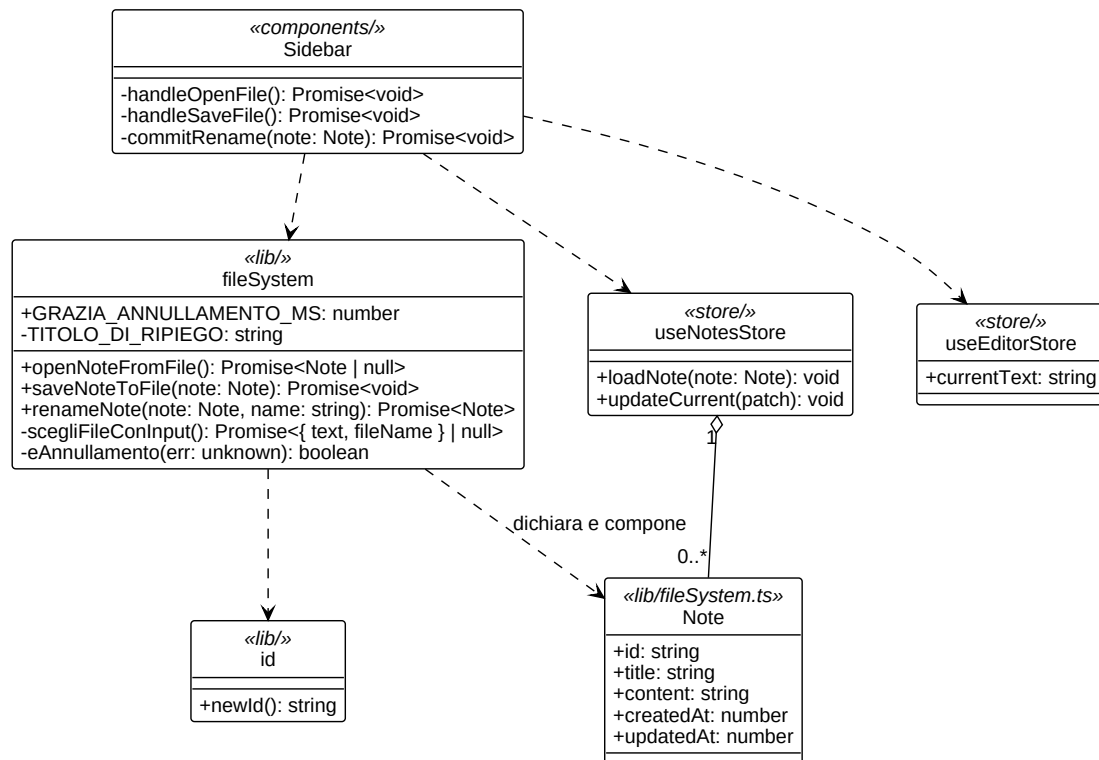
Figura 22: Diagramma UML 4.4.1-1 - Il modulo lib/fileSystem.ts e le sue dipendenze
