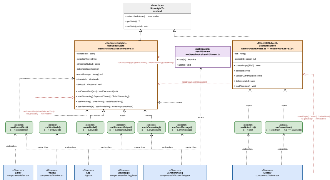
Figura 19: Diagramma soggetto-osservatori degli store e dei selettori
