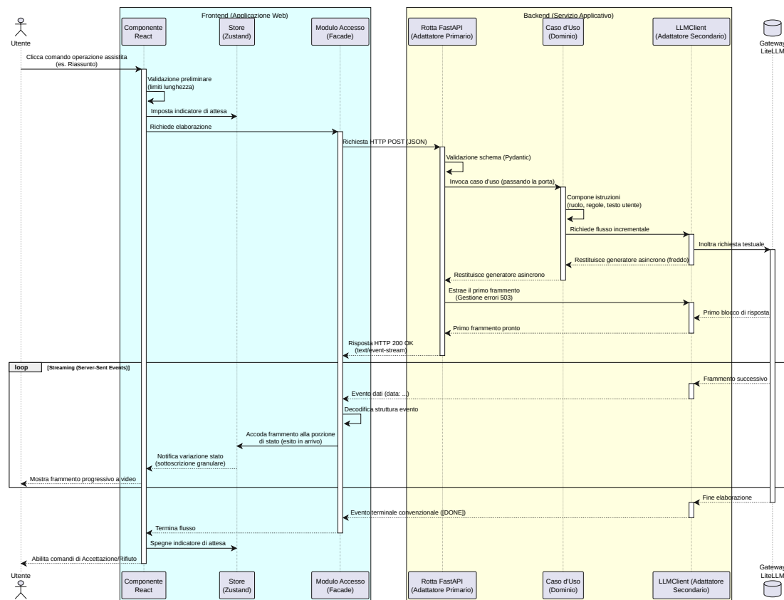
Figura 21: Diagramma di sequenza di un'operazione assistita con risposta in streaming
