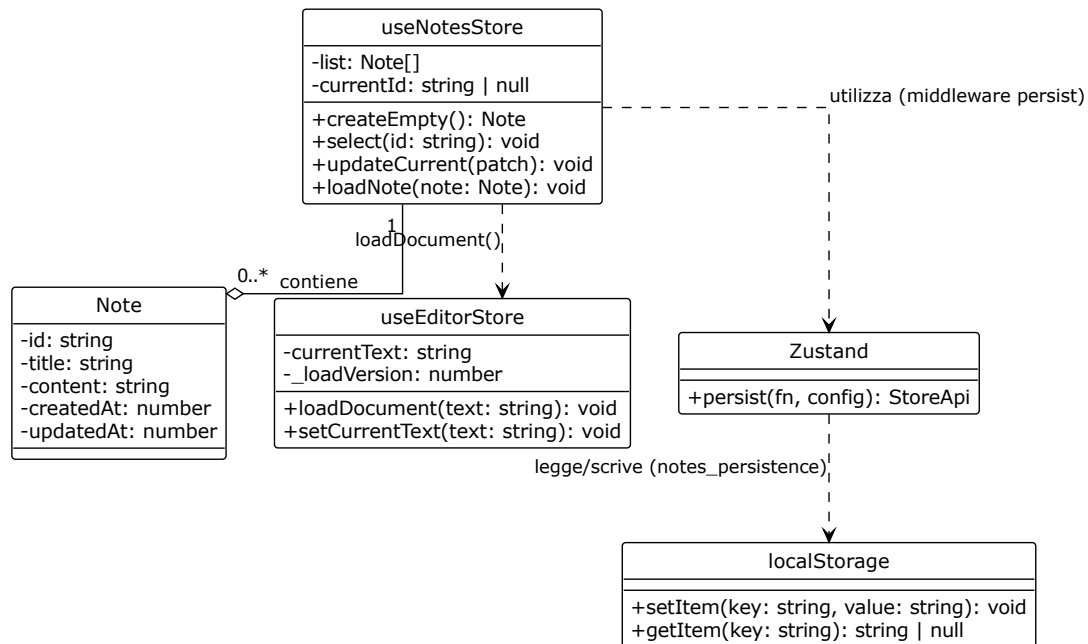
Figura 27: Diagramma UML 4.4.2-3 - continuità della sessione
