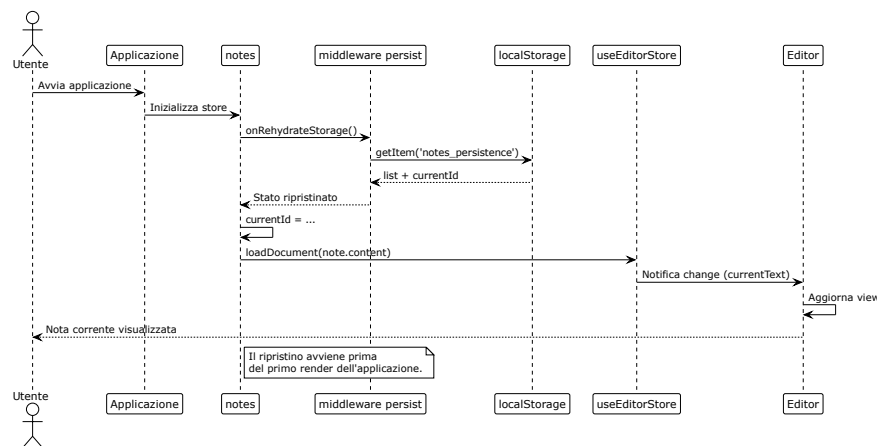
Figura 26: Diagramma UML 4.4.2-2 - lettura all'avvio
