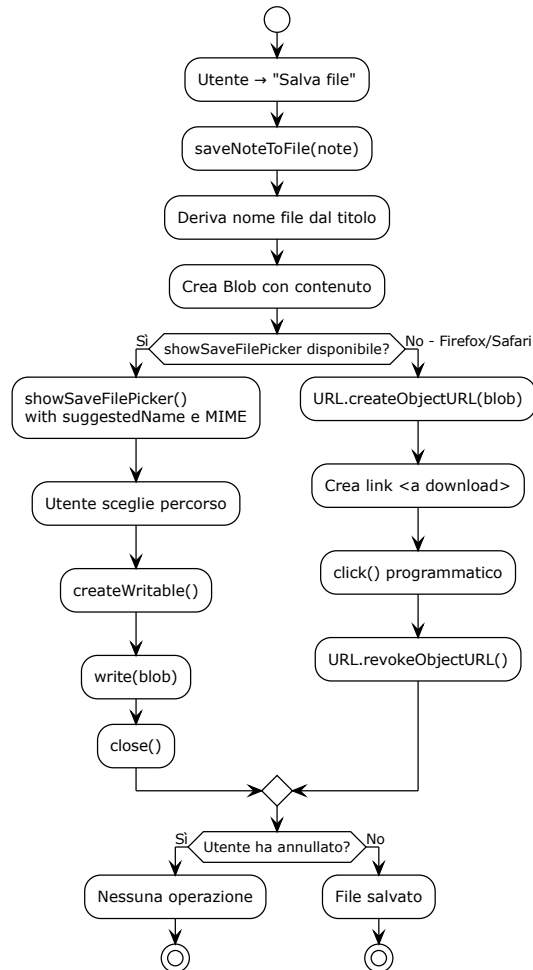
Figura 22: Diagramma UML 4.4.1-1 - fileSystem
