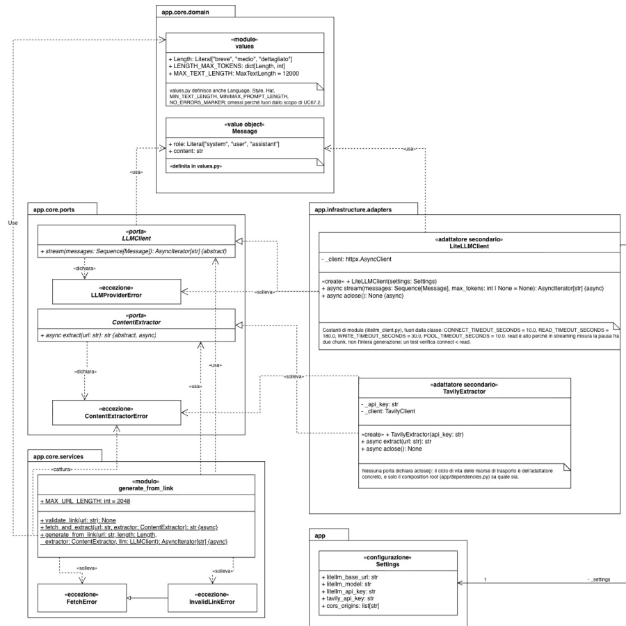
Figura 16: Architettura del servizio applicativo
