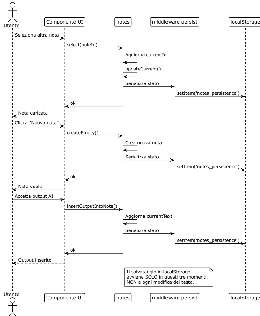
Figura 25: Diagramma UML 4.4.2-1 - salvataggio automatico in localStorage
