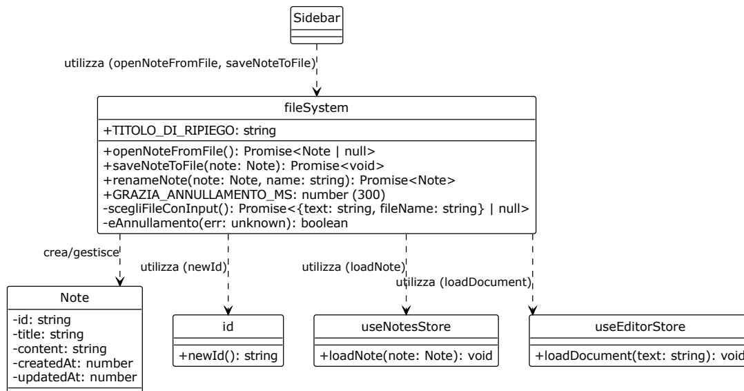
Figura 28: Diagramma UML 4.4.3 - nota creata nel prodotto vs nota importata da disco
