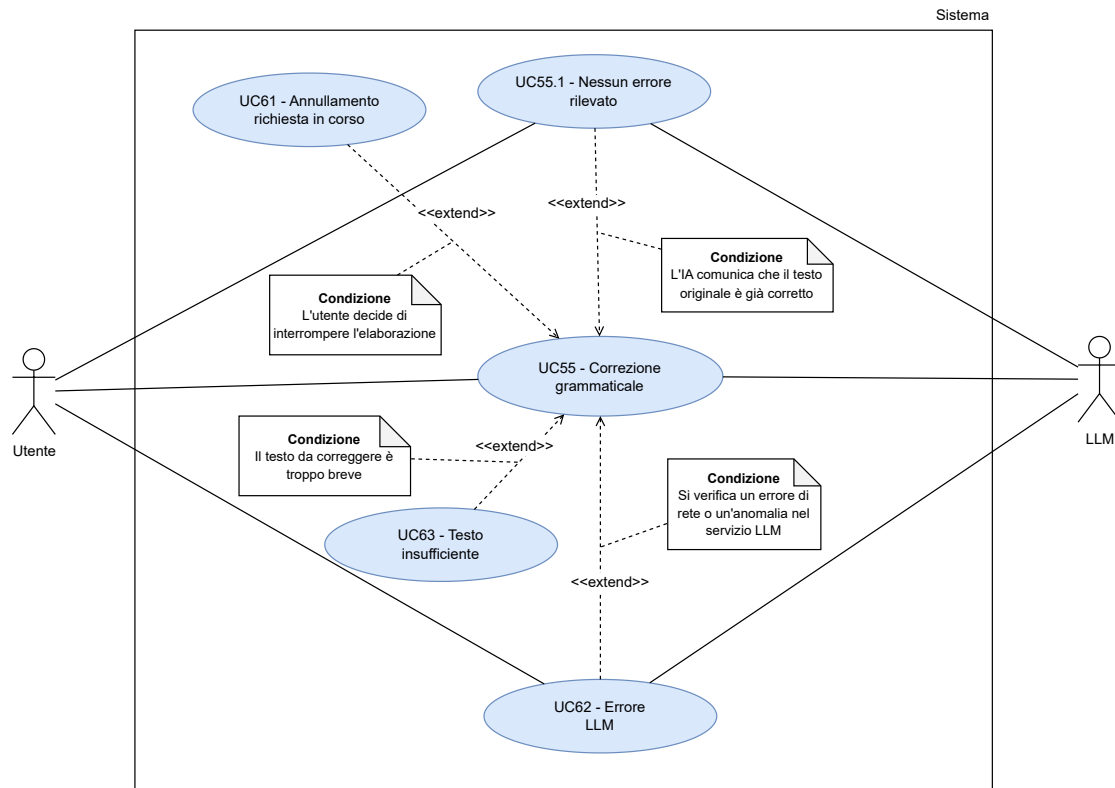
Figura 61: UC55 - Correzione Grammaticale
