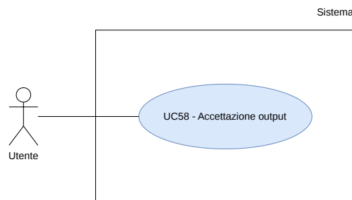
Figura 66: UC58 - Accettazione output
