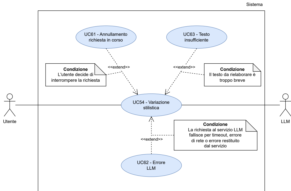
Figura 59: UC54 - Variazione Stilistica
