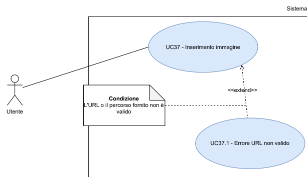
Figura 40: UC37 - Inserimento immagine
