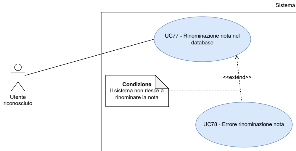
Figura 78: UC77 - Rinominazione nota nel database
