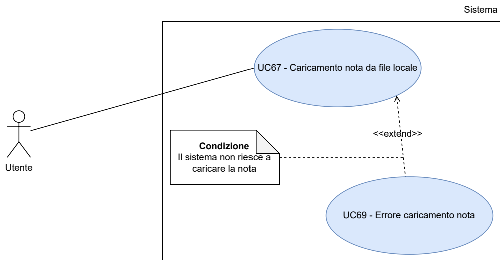
Figura 71: UC67 - Caricamento nota da file locale
