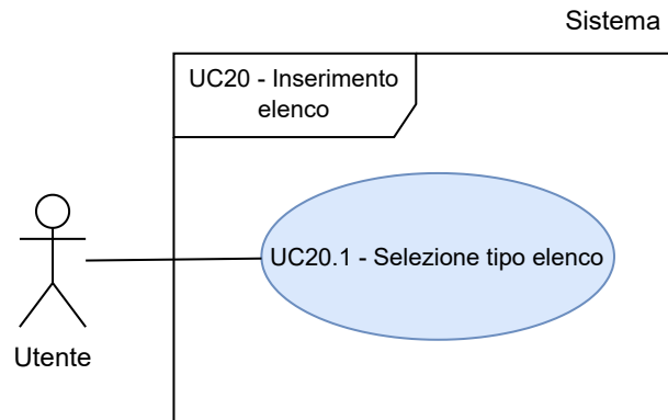
Figura 22: UC20.1 - Inclusione di UC20
