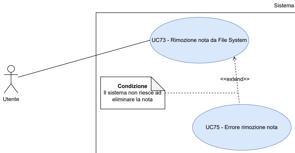
Figura 75: UC73 - Rimozione nota da File System
