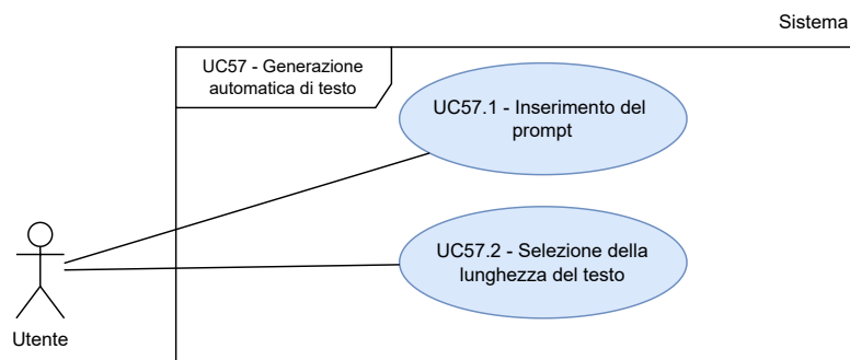
Figura 65: UC57.1, UC57.2 - Inclusioni di UC57
