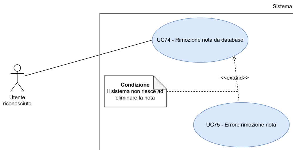
Figura 76: UC74 - Rimozione nota da database
