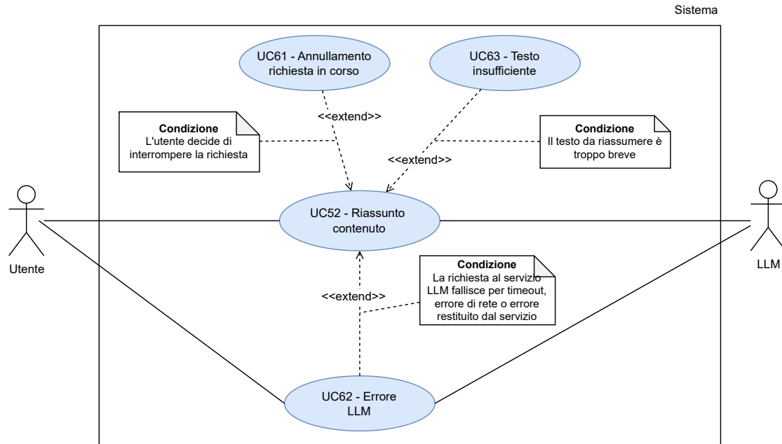
Figura 55: UC52 - Riassunto Contenuto
