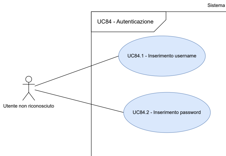
Figura 85: UC84.1, UC84.2 - Inclusioni di UC84
