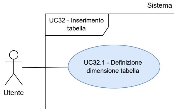
Figura 35: UC32.1 - Inclusione di UC32
