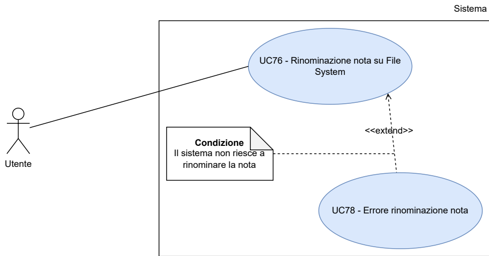
Figura 77: UC76 - Rinominazione nota su File System
