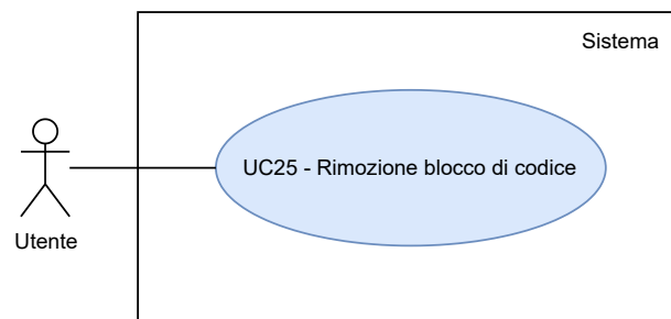
Figura 27: UC25 - Rimozione blocco di codice
