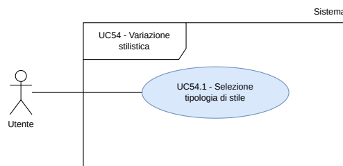
Figura 60: UC54.1 - Inclusione di UC54
