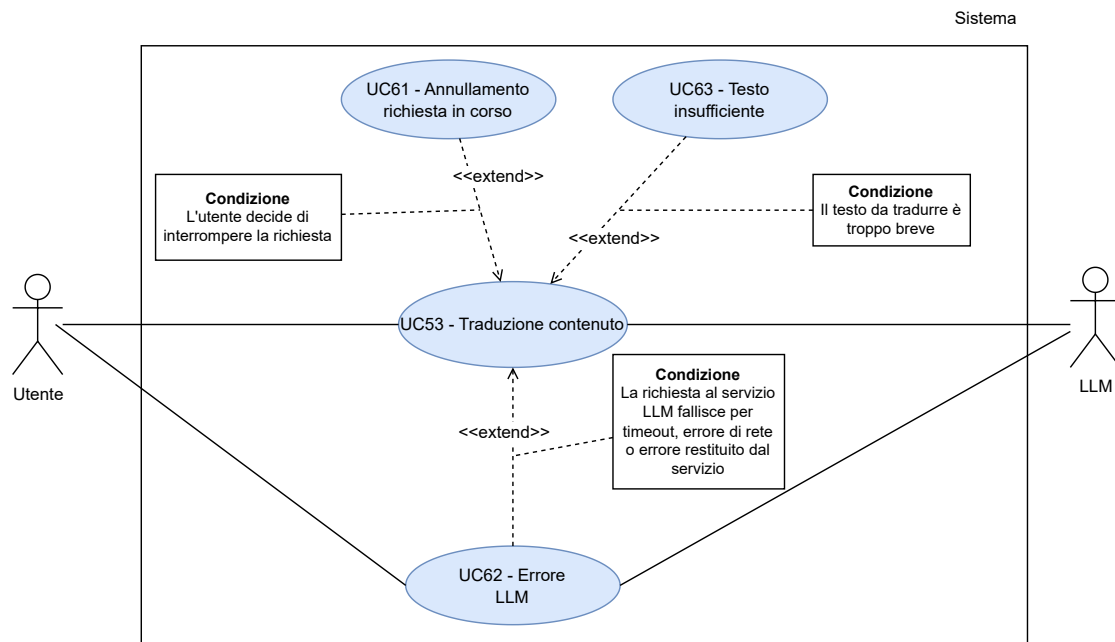
Figura 57: UC53 - Traduzione Contenuto
