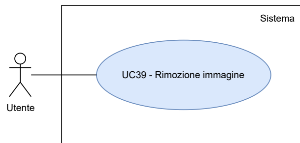
Figura 42: UC39 - Rimozione immagine
