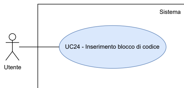
Figura 26: UC24 - Inserimento blocco di codice
