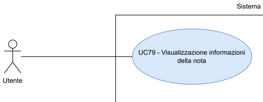
Figura 79: UC79 - Visualizzazione informazioni della nota
