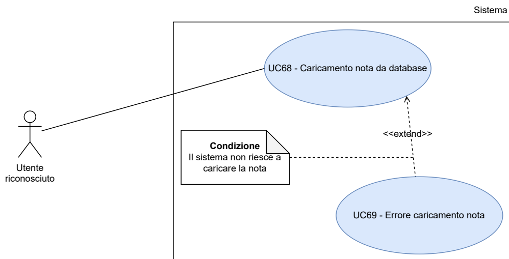
Figura 72: UC68 - Caricamento nota da database
