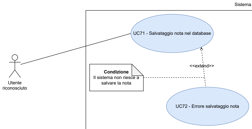
Figura 74: UC71 - Salvataggio nota nel database
