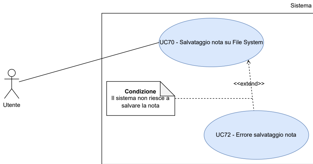
Figura 73: UC70 - Salvataggio nota su File System
