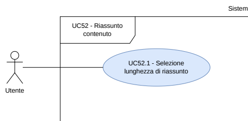
Figura 56: UC52.1 - Inclusione di UC52
