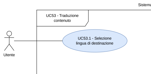
Figura 58: UC53.1 - Inclusione di UC53
