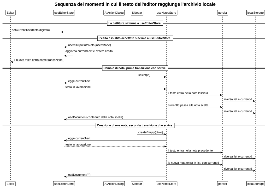
Figura 29: Diagramma UML 4.4.2-2 - Sequenza dei momenti in cui il testo dell'editor raggiunge l'archivio locale
