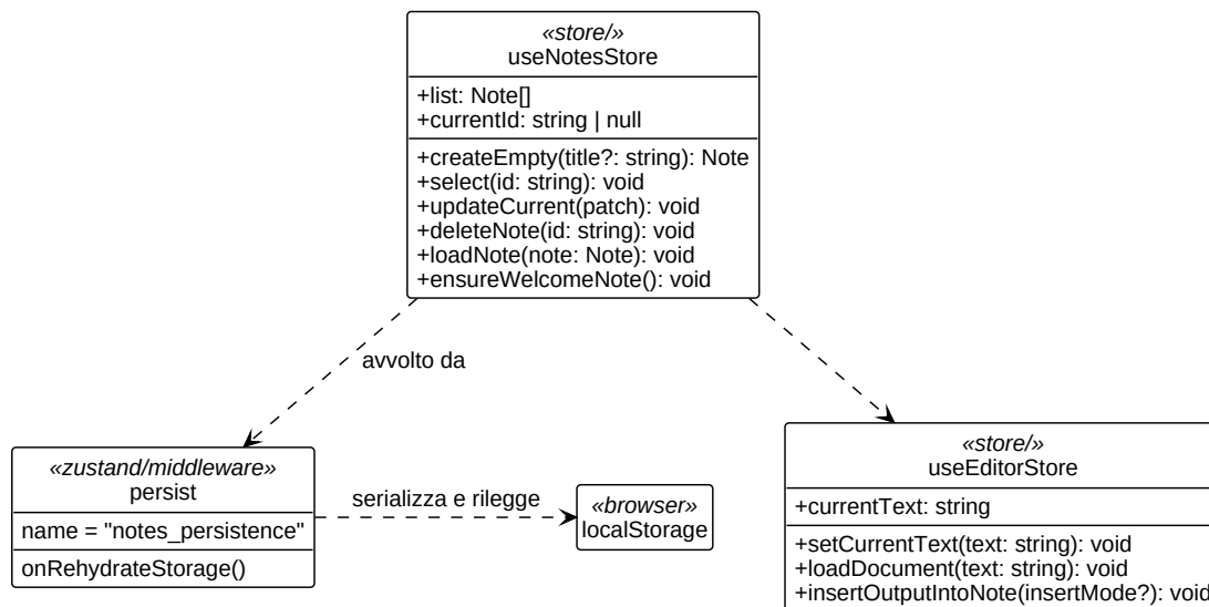
Figura 28: Diagramma UML 4.4.2-1 - La catena di persistenza dello store delle note
