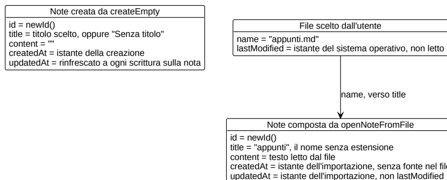
Figura 31: Diagramma UML 4.4.3 - Provenienza dei metadati per una nota creata nel prodotto e per una importata da file
