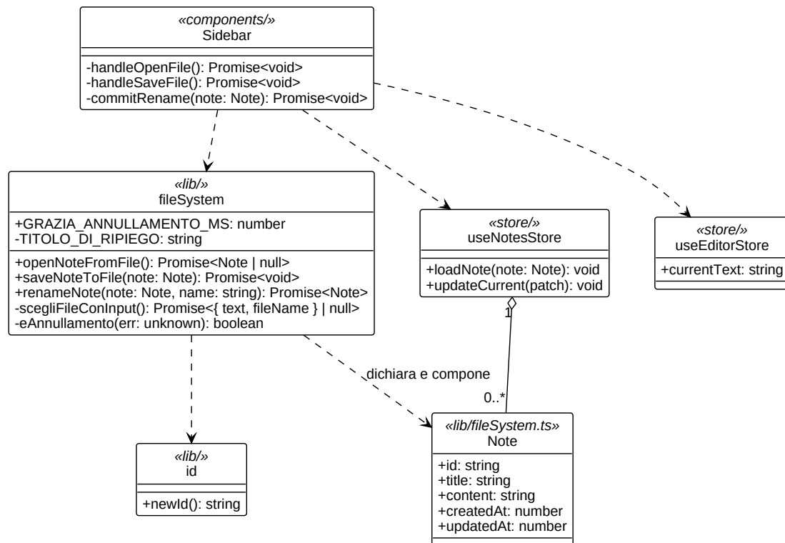
Figura 25: Diagramma UML 4.4.1-1 - Il modulo lib/fileSystem.ts e le sue dipendenze
