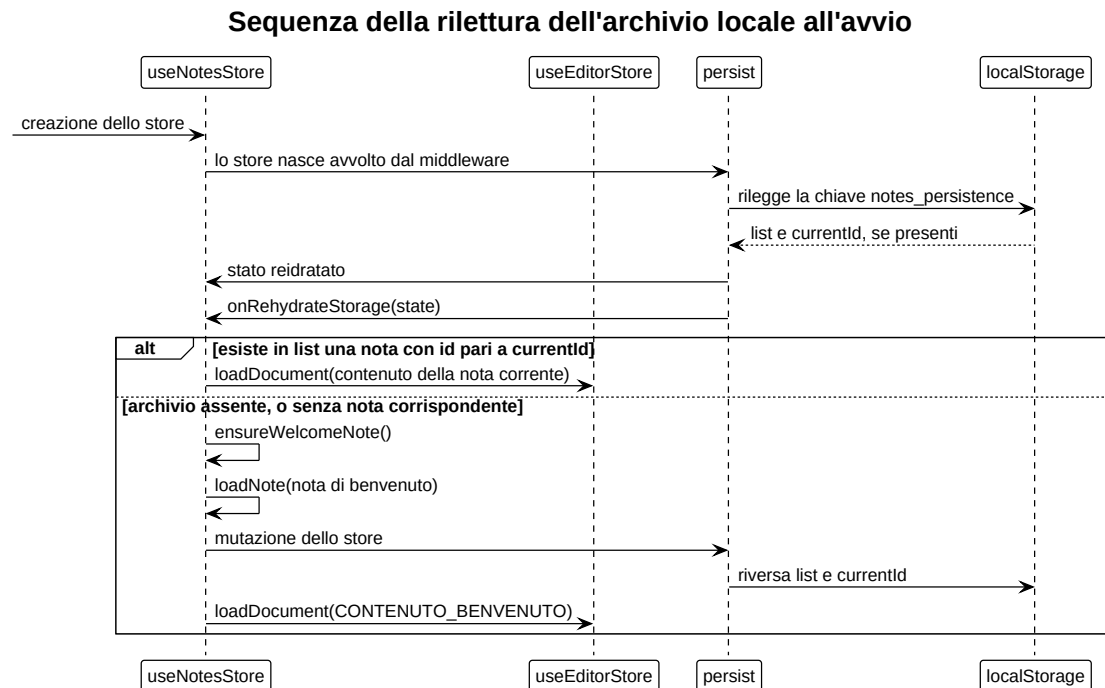
Figura 30: Diagramma UML 4.4.2-3 - Sequenza della rilettura dell'archivio locale all'avvio
