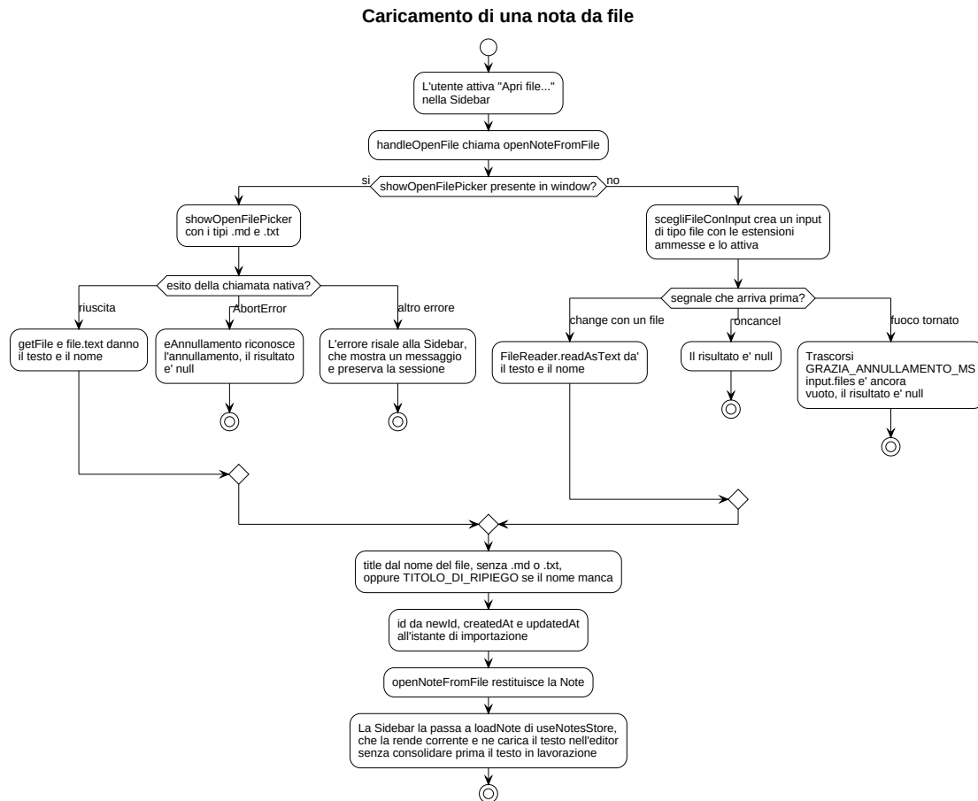
Figura 27: Diagramma UML 4.4.1-3 - Caricamento di una nota da file
