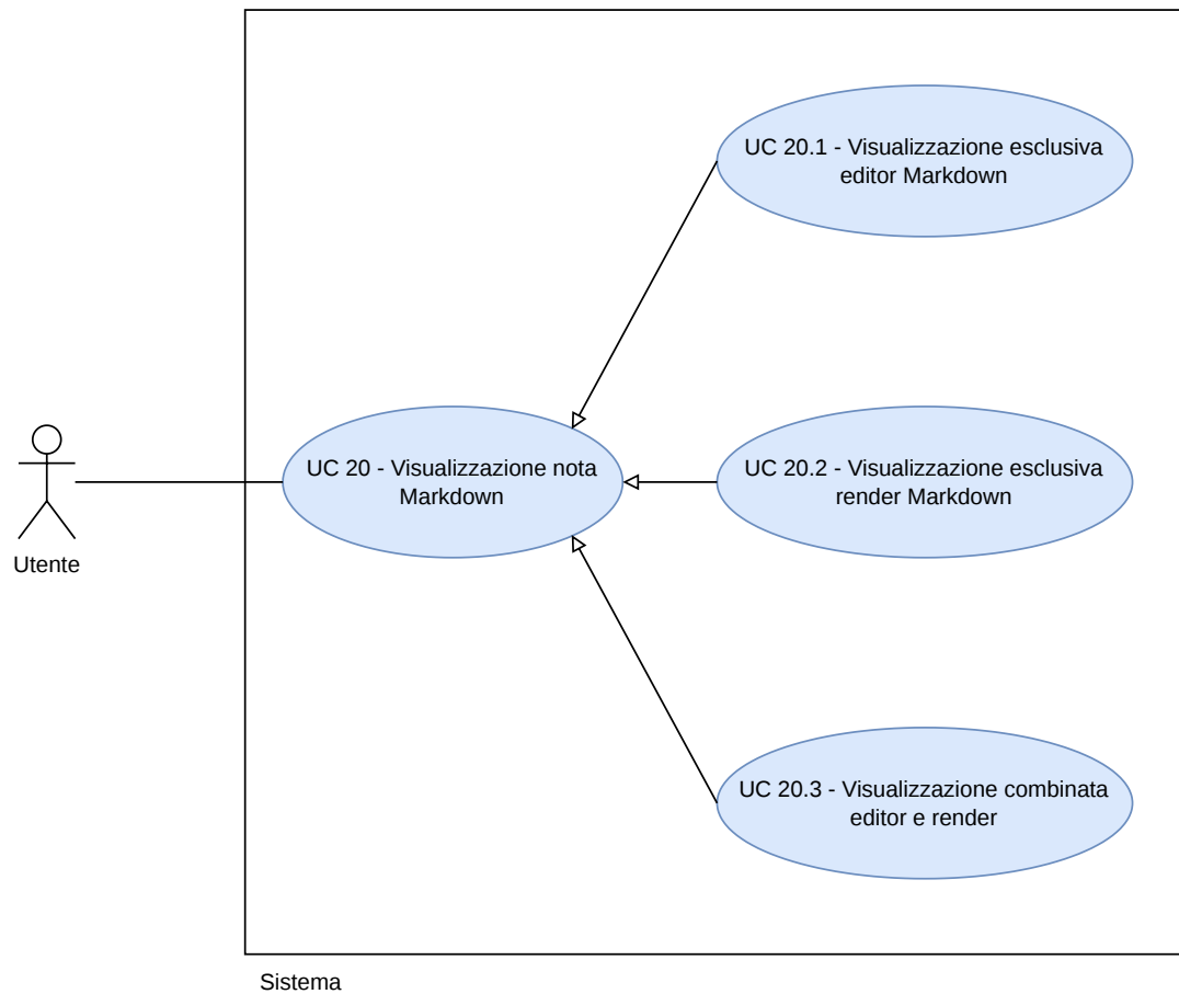
Figura 70: Diagramma UC20
