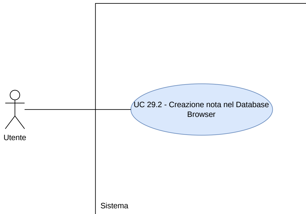
Figura 113: Diagramma UC29.2
