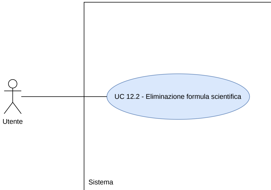
Figura 46: Diagramma UC12.2
