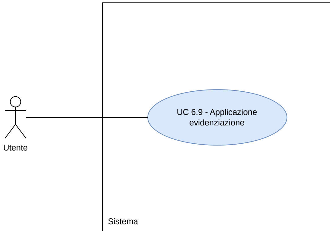
Figura 20: Diagramma UC6.9
