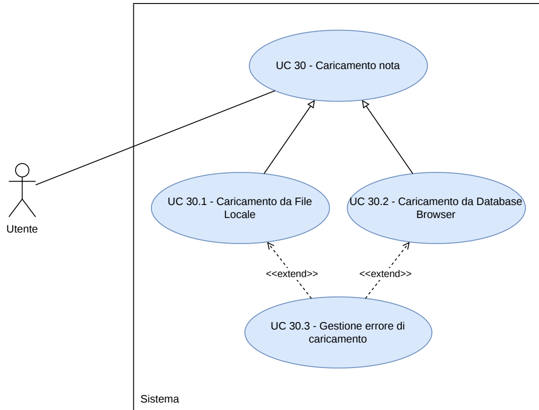
Figura 115: Diagramma UC30
