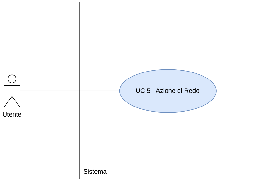
Figura 10: Diagramma UC5
