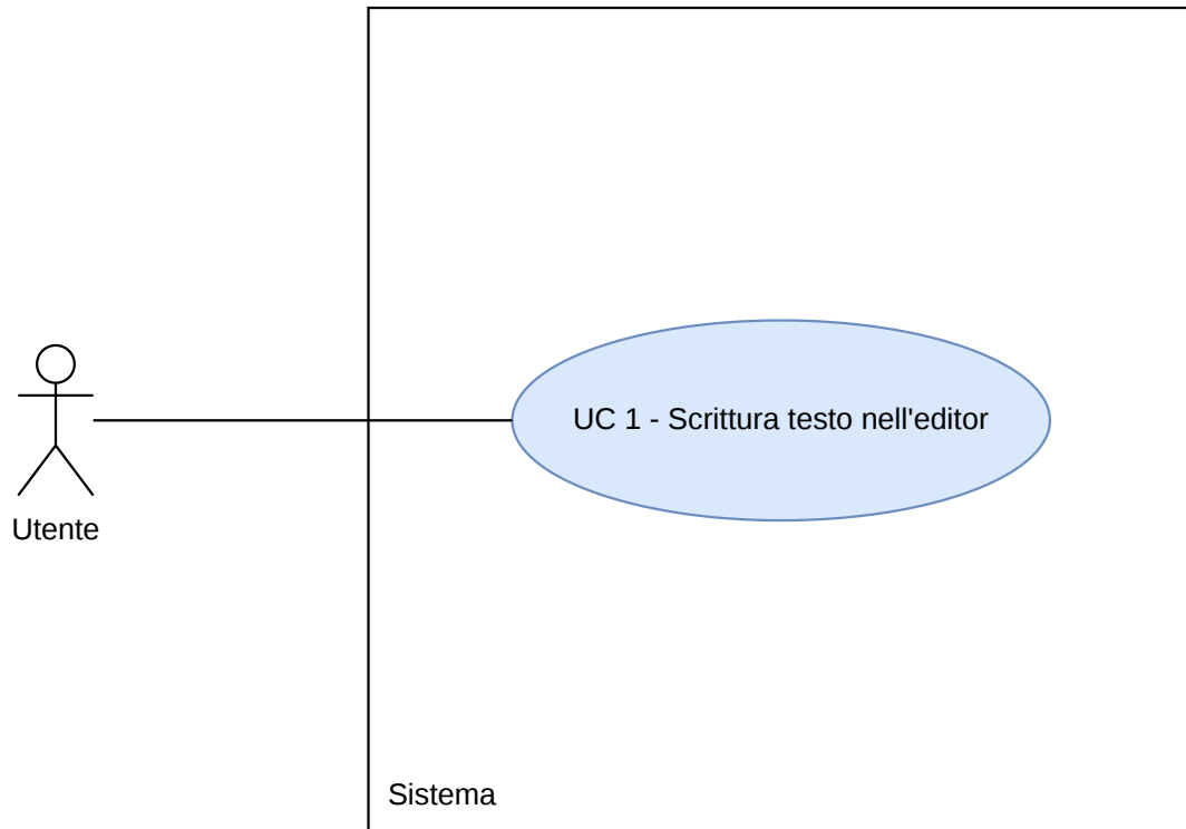
Figura 1: Diagramma UC1
