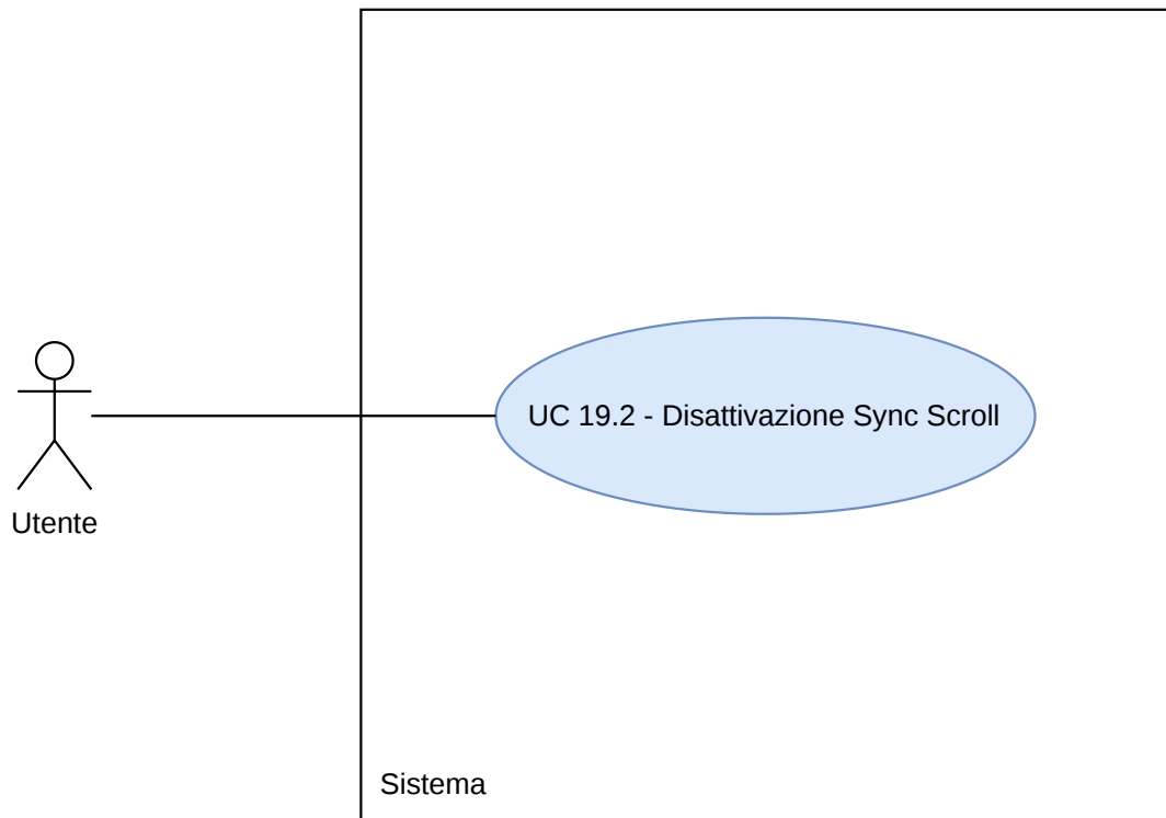
Figura 69: Diagramma UC19.2
