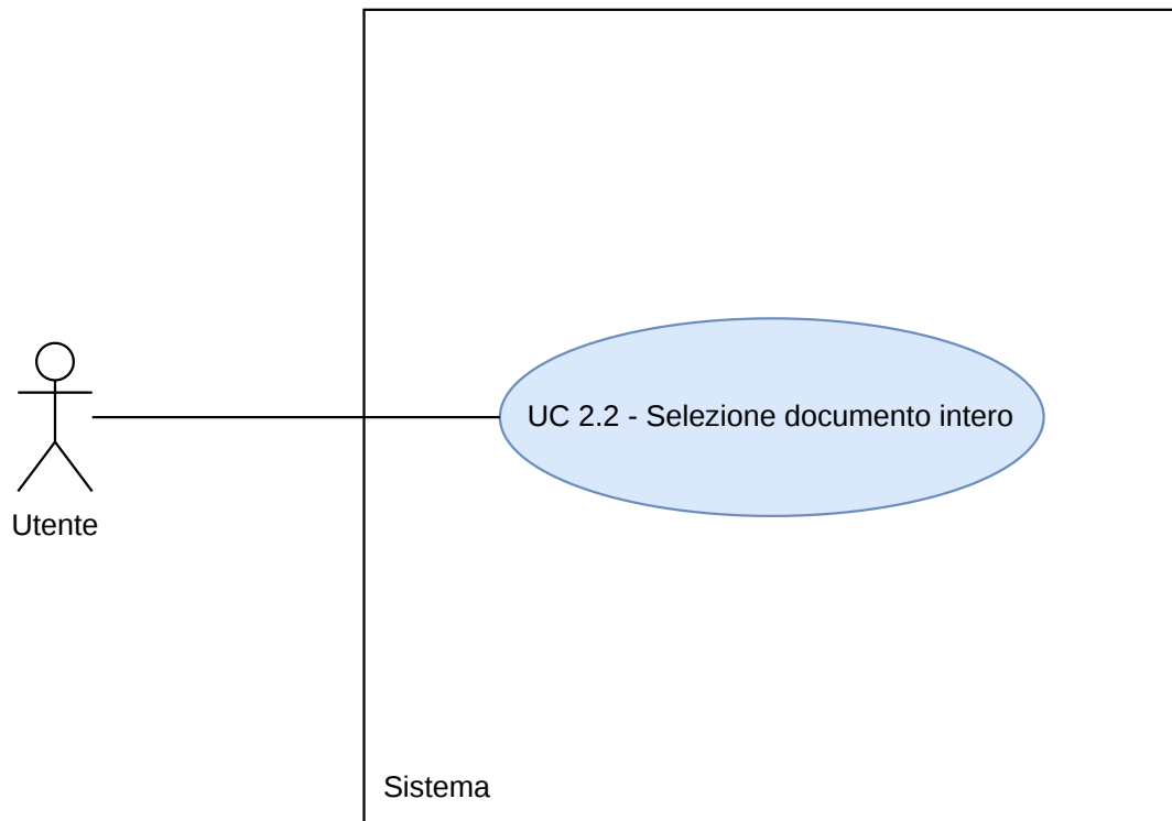
Figura 4: Diagramma UC2.2
