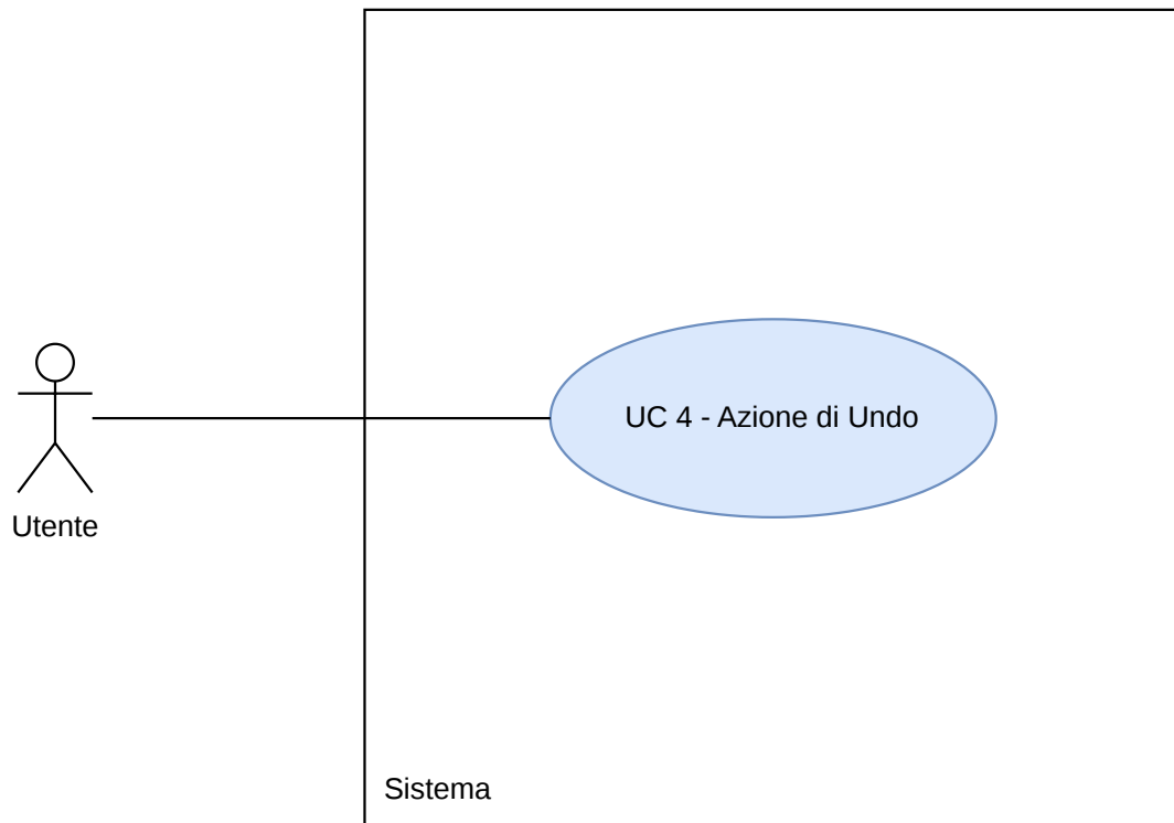
Figura 9: Diagramma UC4
