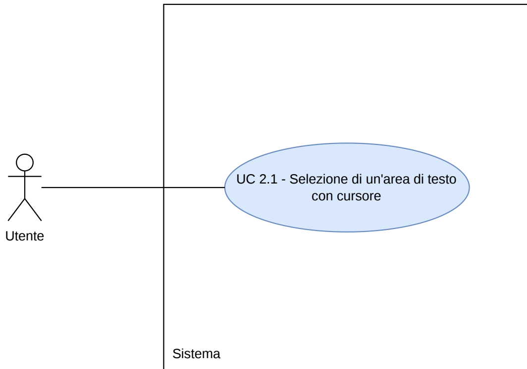
Figura 3: Diagramma UC2.1
