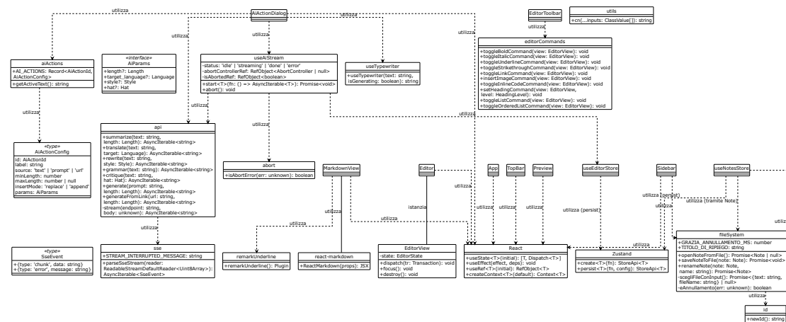
Figura 3: Diagramma UML 3.3-2 - Hooks, Librerie e Dipendenze Esterne
