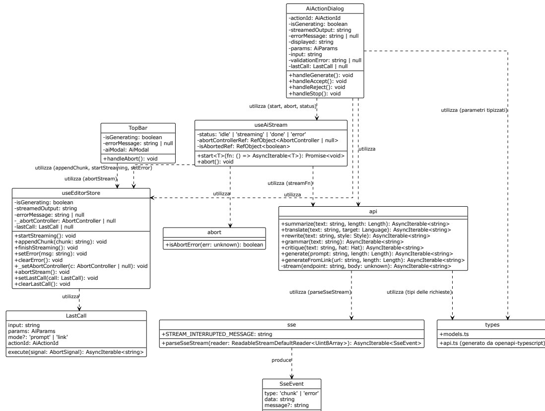
Figura 17: Diagramma UML 3.3.5 - Accesso al servizio applicativo
