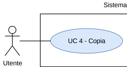
Figura 2: UC 4 - Copia
