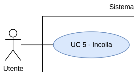
Figura 3: UC 5 - Incolla
