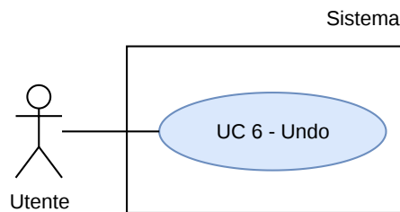
Figura 4: UC 6 - Undo
