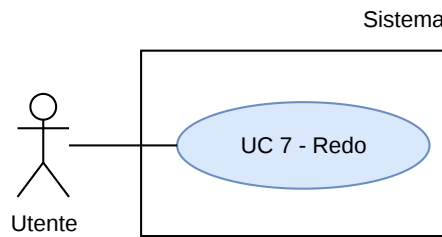
Figura 5: UC 7 - Redo
