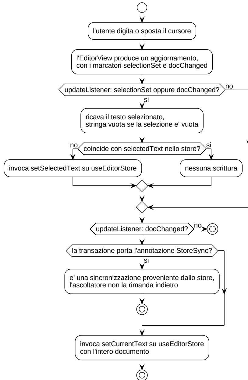
Figura 15: Diagramma UML 3.3.4-1 - Sincronizzazione editor → store
