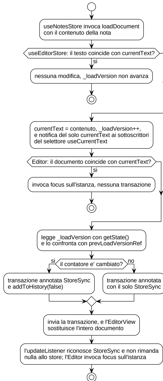
Figura 16: Diagramma UML 3.3.4-2 - Sincronizzazione store → editor
