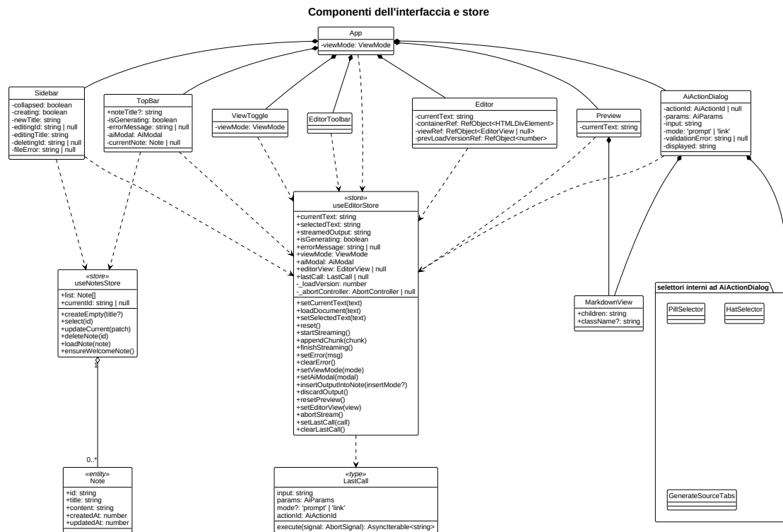
Figura 2: Diagramma UML 3.3-1 - Componenti UI e Store
