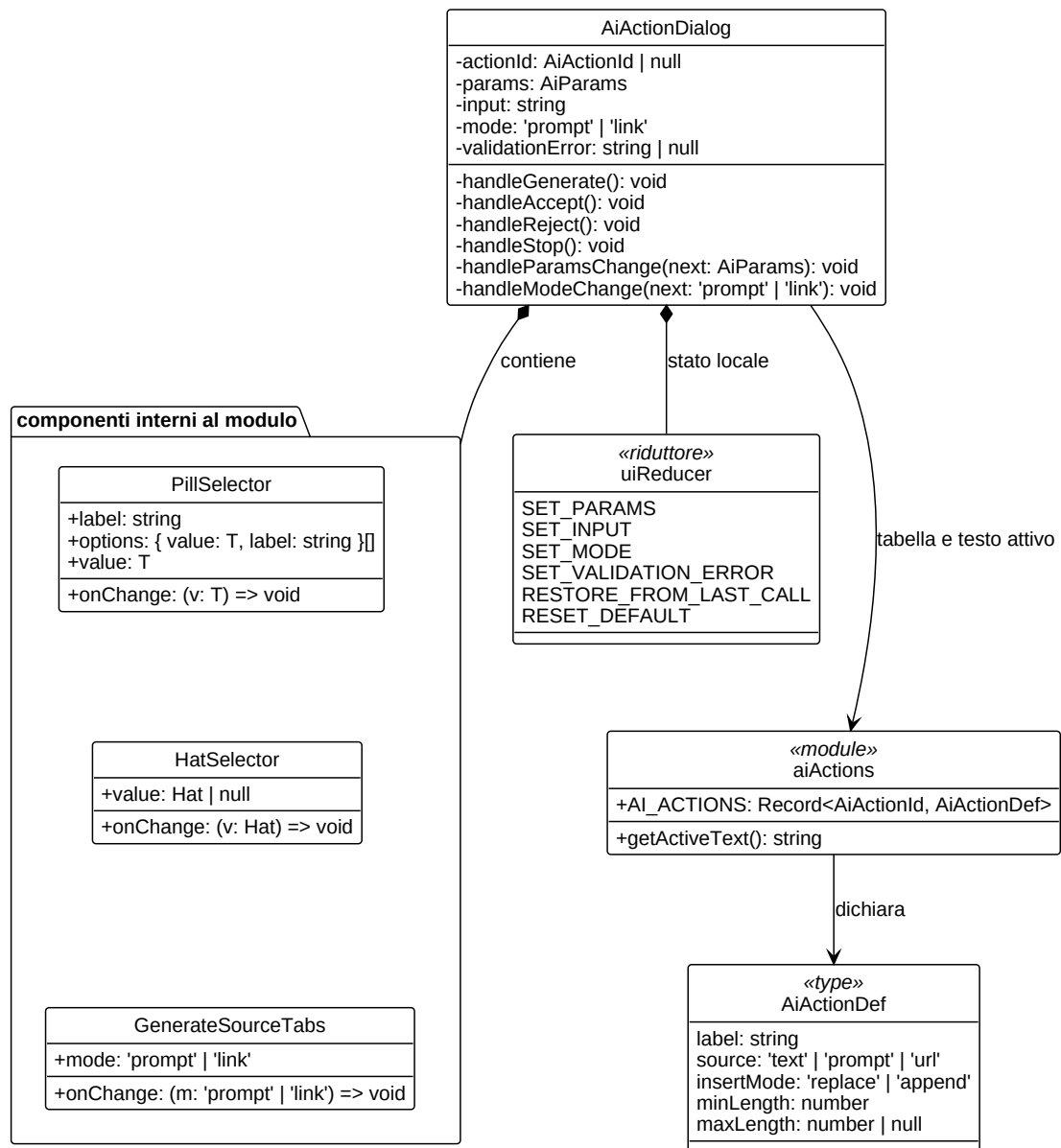
Figura 12: Diagramma UML 3.3.2-8 - AiActionDialog
