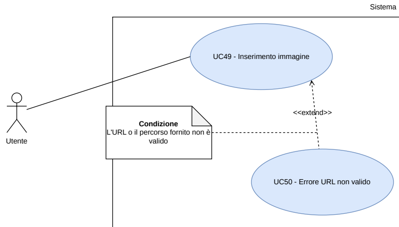
Figura 52: UC49 - Inserimento immagine
