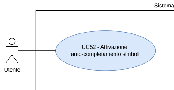
Figura 54: UC52 - Attivazione auto-completamento simboli
