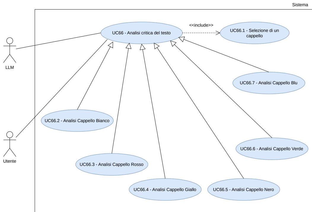
Figura 72: UC66.1, 66.2, 66.3, 66.4, 66.5, 66.6, 66.7 - Inclusione di UC66 e generalizzazioni
