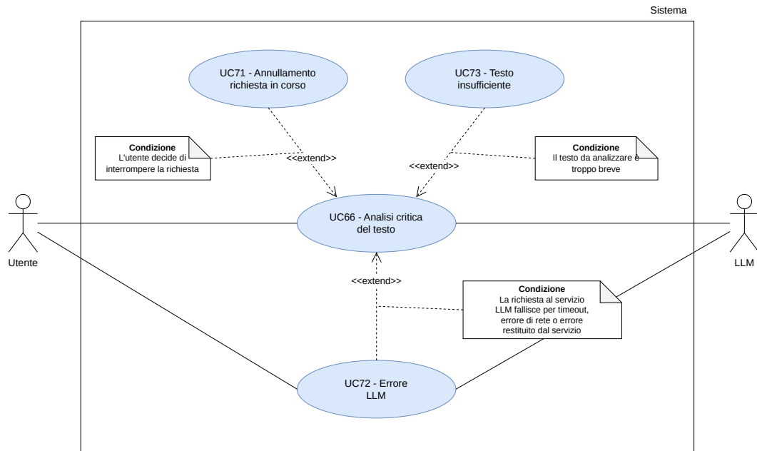
Figura 71: UC66 - Analisi Critica del testo
