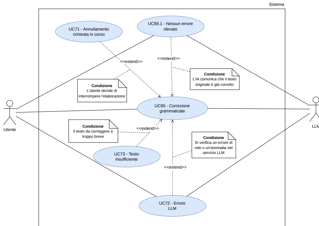
Figura 70: UC65 - Correzione Grammaticale
