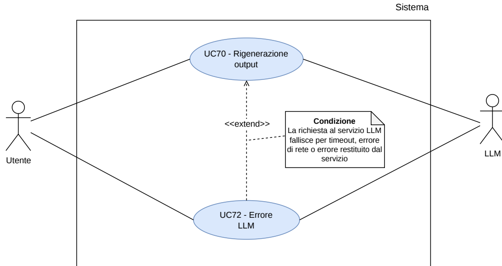
Figura 79: UC70 - Rigenerazione output
