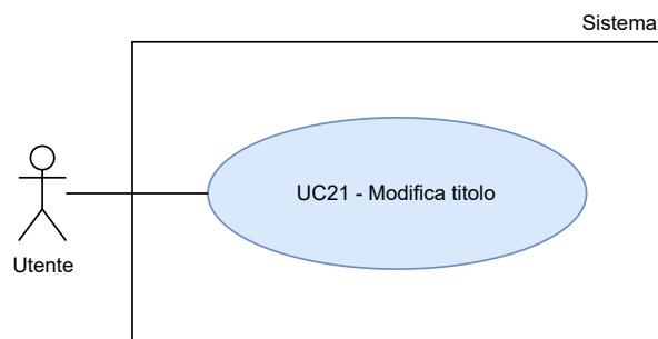
Figura 22: UC21 - Modifica titolo
