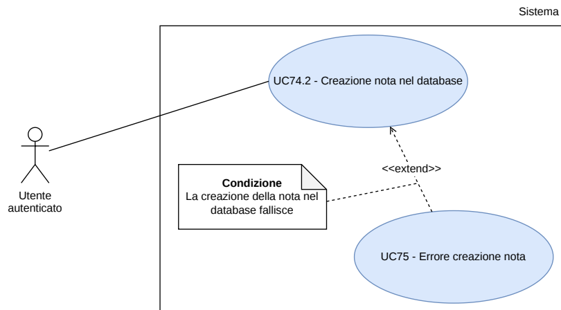
Figura 81: UC74.2 - Creazione nota nel database
