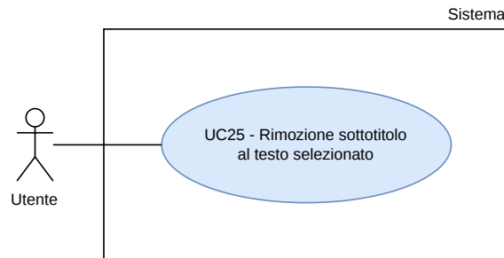
Figura 26: UC25 - Rimozione sottotitolo al testo selezionato
