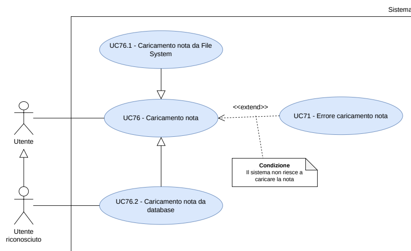
Figura 82: UC76 - Caricamento nota
