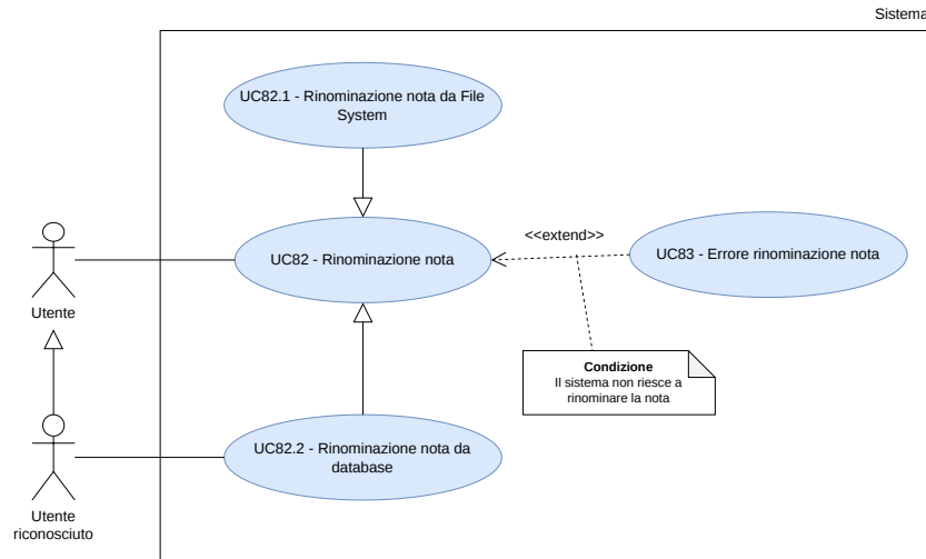
Figura 85: UC82 - Rinominazione nota
