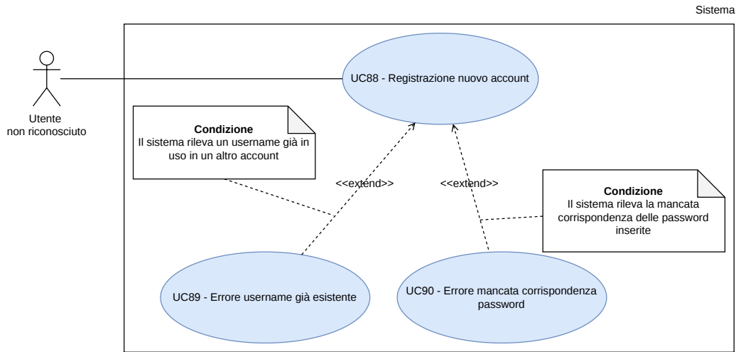
Figura 90: UC88 - Registrazione nuovo account
