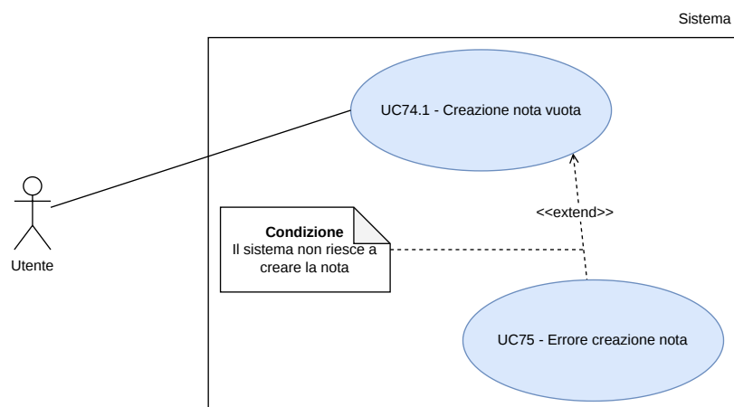
Figura 80: UC74.1 - Creazione nota vuota
