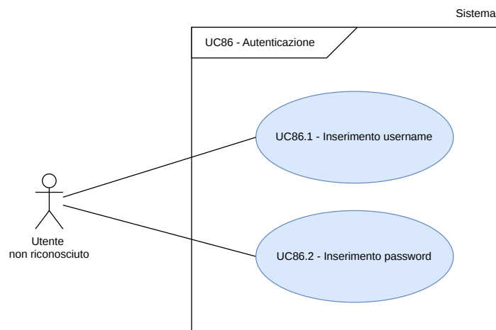
Figura 89: UC86.1, UC86.2 - Inclusioni di UC86
