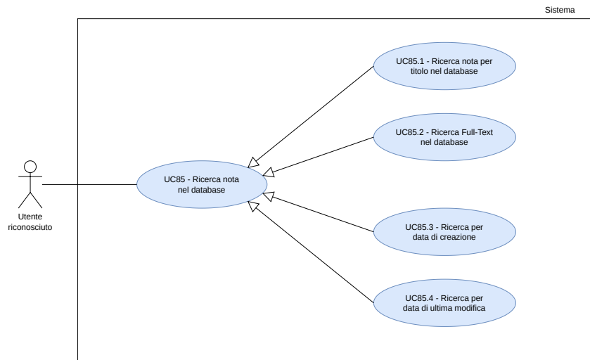
Figura 87: UC85 - Ricerca nota nel database
