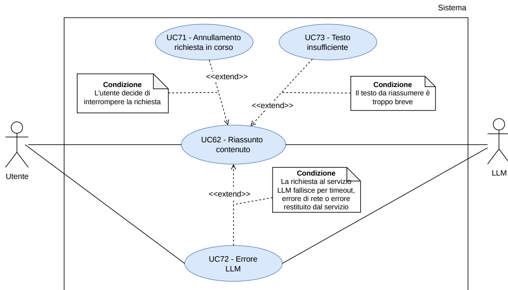
Figura 64: UC62 - Riassunto Contenuto
