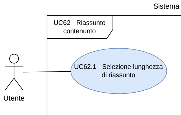
Figura 65: UC62.1 - Inclusione di UC62
