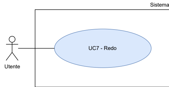
Figura 8: UC7 - Redo
