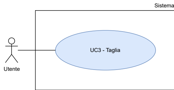
Figura 4: UC3 - Taglia
