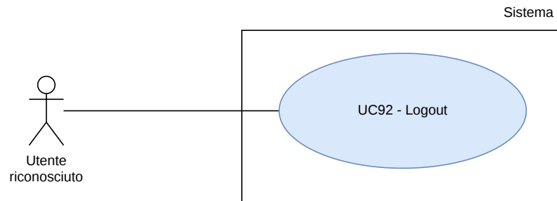
Figura 93: UC92 - Logout
