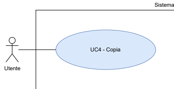
Figura 5: UC4 - Copia
