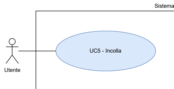
Figura 6: UC5 - Incolla
