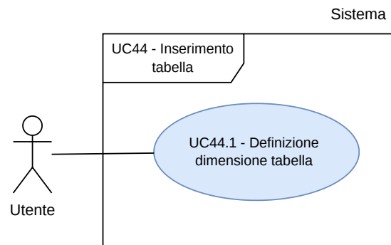
Figura 47: UC44.1 - Inclusione di UC44
