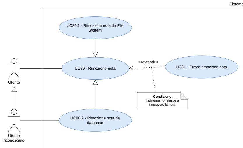
Figura 84: UC80 - Rimozione nota
