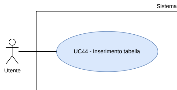
Figura 46: UC44 - Inserimento tabella
