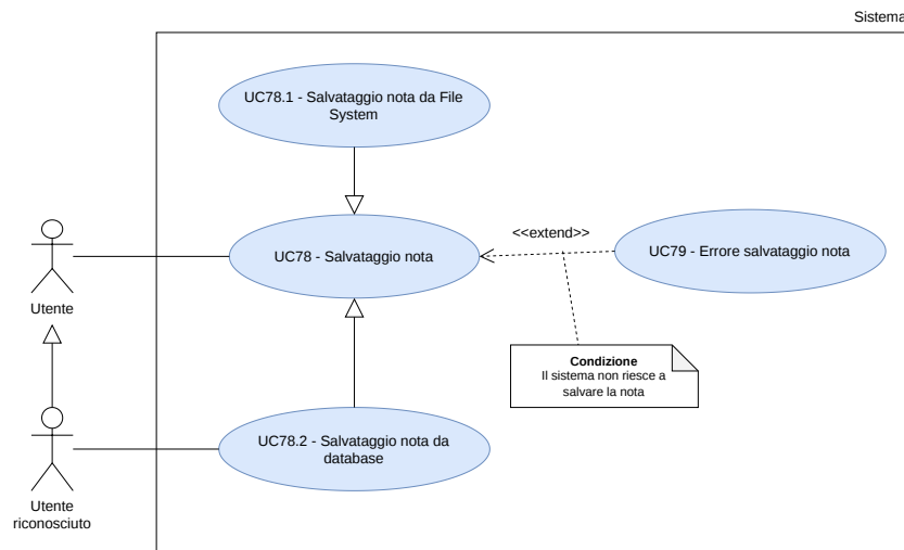
Figura 83: UC78 - Salvataggio nota
