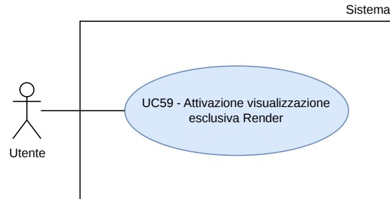
Figura 61: UC59 - Attivazione visualizzazione esclusiva Render
