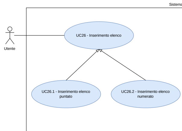
Figura 27: UC26 - Inserimento elenco
