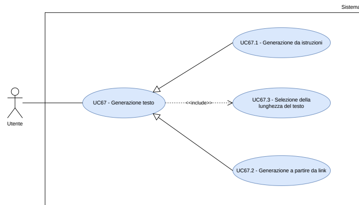
Figura 74: UC67 - Generalizzazione della generazione testo e inclusione UC67.3
