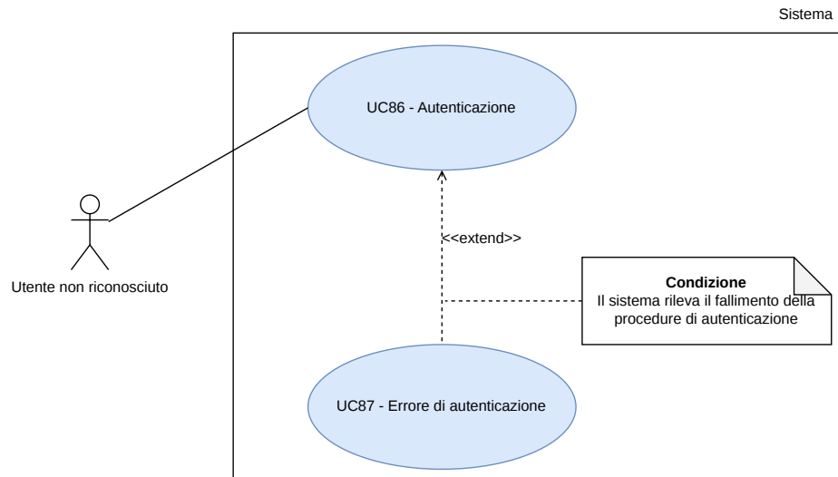
Figura 88: UC86 - Autenticazione
