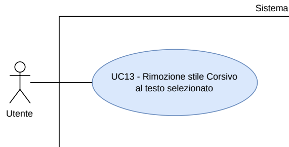
Figura 14: UC13 - Rimozione stile Corsivo al testo selezionato
