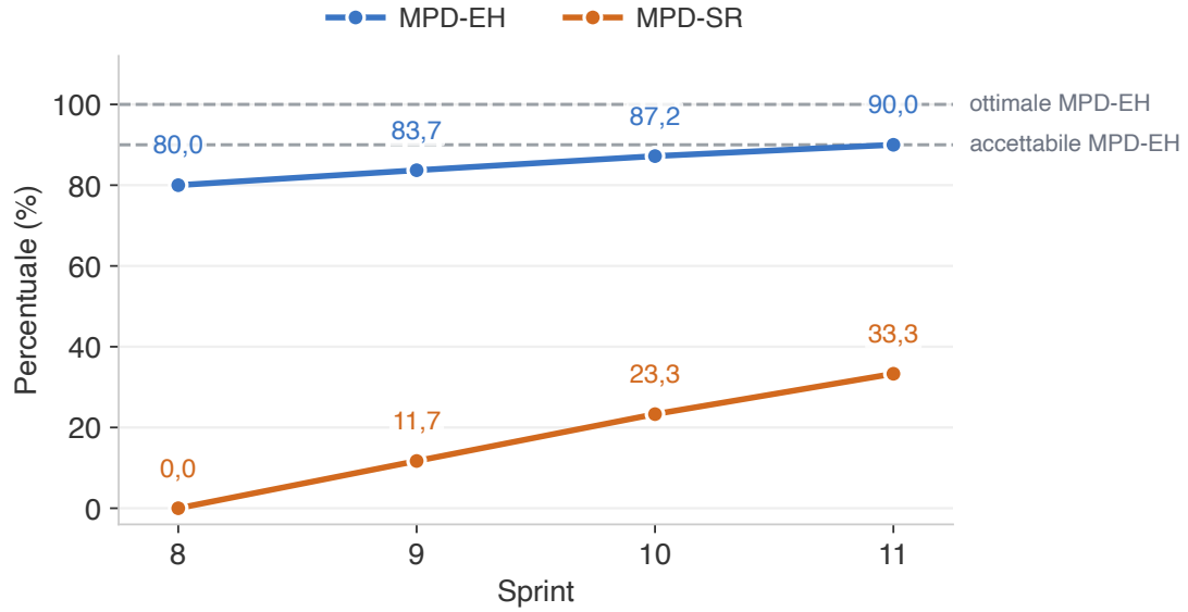
Figura 17: Valutazione Error Handling e Session Recovery
