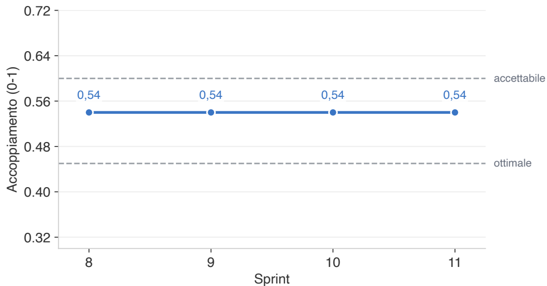
Figura 27: Valutazione Modularità
