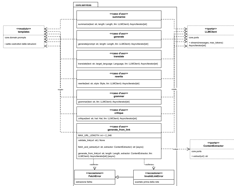
Figura 19: I sette casi d'uso e le dipendenze verso le porte
