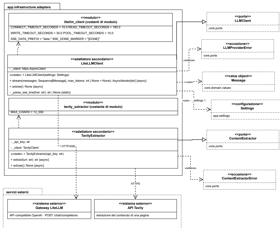
Figura 22: Adattatori secondari e servizi esterni
