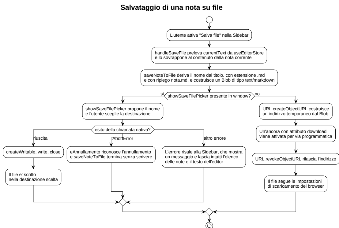
Figura 30: Diagramma UML 4.4.1-2 - Salvataggio di una nota su file
