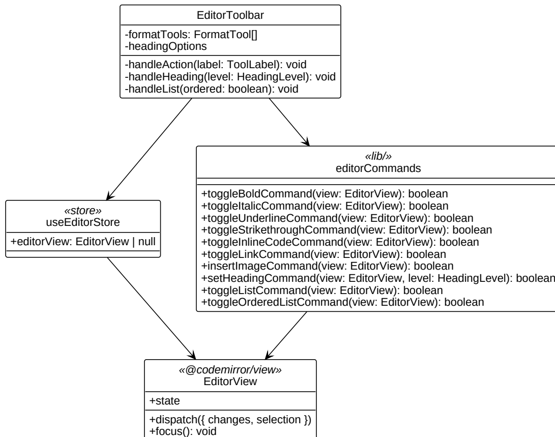
Figura 7: Diagramma UML 3.3.2-3 - EditorToolbar
