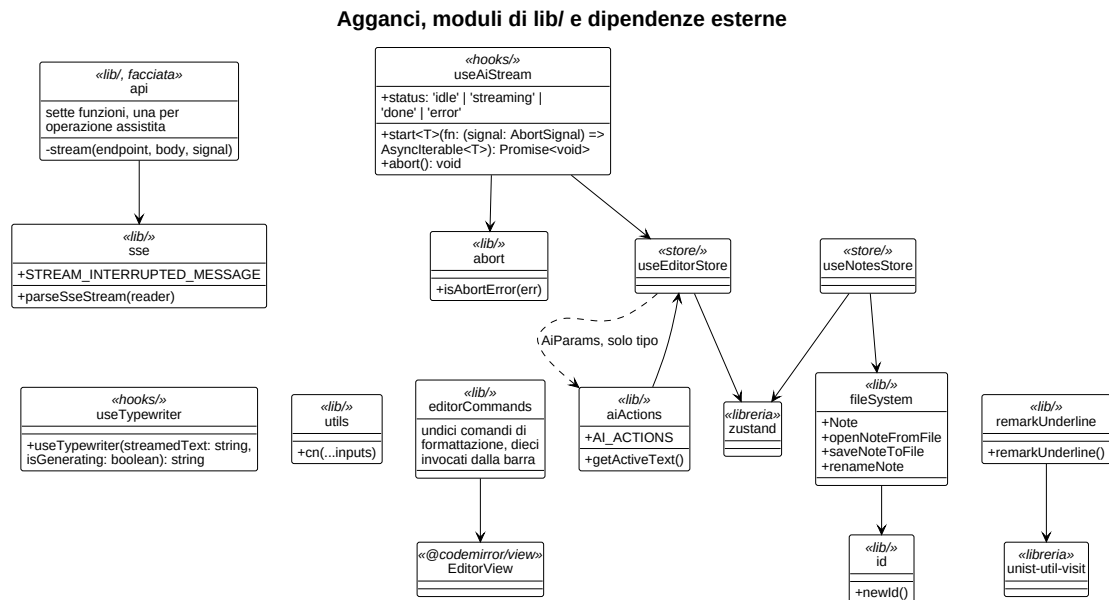
Figura 3: Diagramma UML 3.3-2 - Agganci, moduli di lib/ e dipendenze esterne
