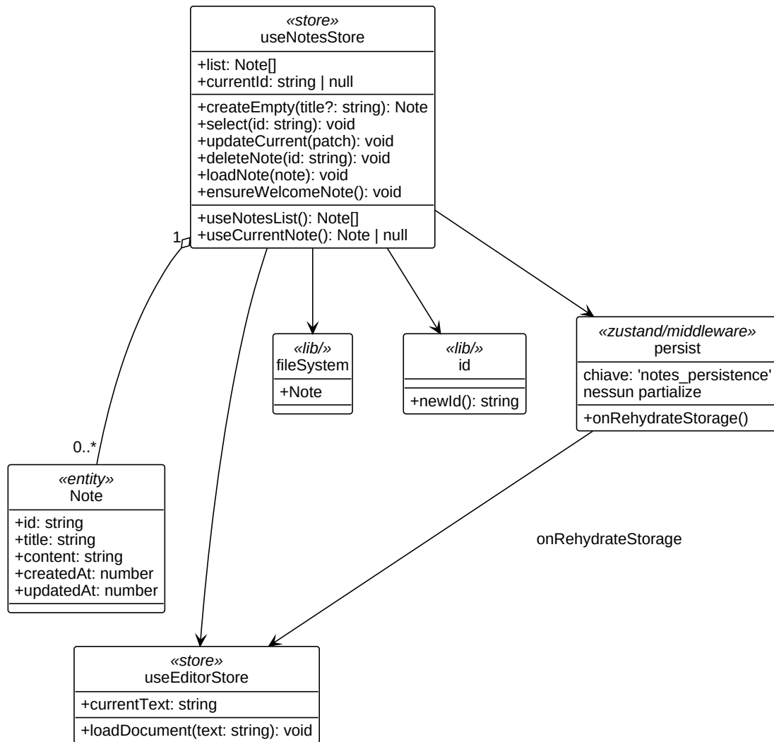
Figura 11: Diagramma UML 3.3.3-2 - useNotesStore
