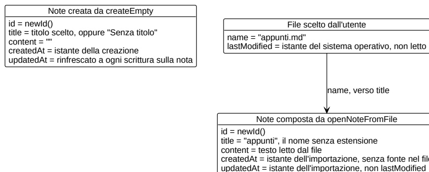
Figura 35: Diagramma UML 4.4.3 - Provenienza dei metadati per una nota creata nel prodotto e per una importata da file
