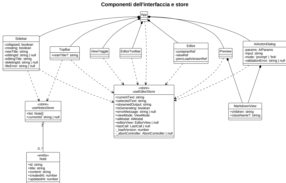
Figura 2: Diagramma UML 3.3-1 - Componenti dell'interfaccia e store
