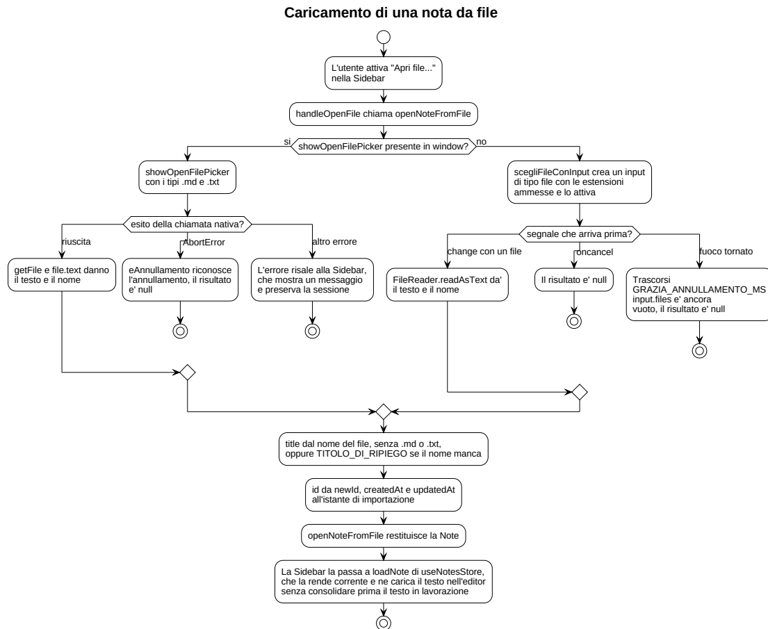
Figura 31: Diagramma UML 4.4.1-3 - Caricamento di una nota da file
