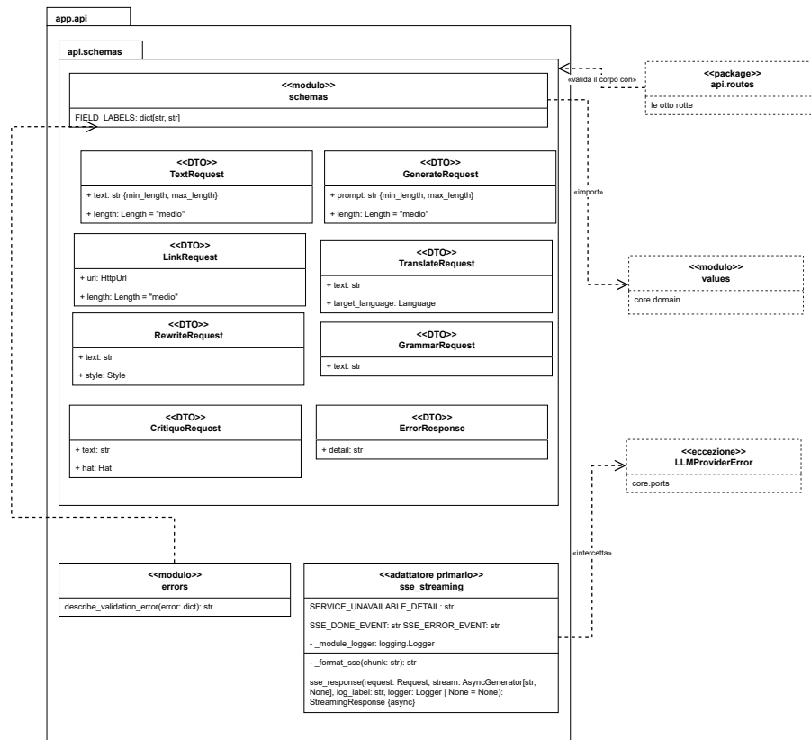
Figura 18: Schemi di validazione, traduzione degli errori e adattatore di trasporto
