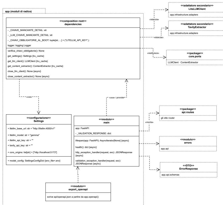
Figura 23: Composition root: provider, configurazione e costruzione dell'applicazione
