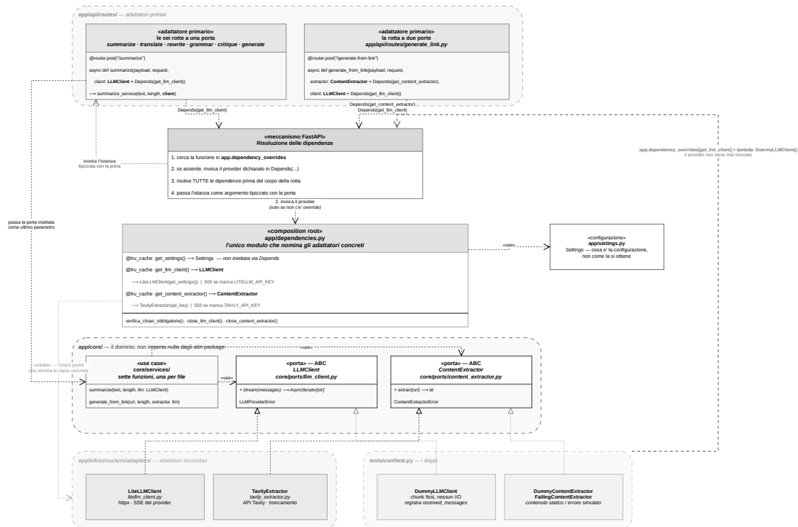
Figura 27: Diagramma della risoluzione della dipendenza e della sostituzione con un doppio
