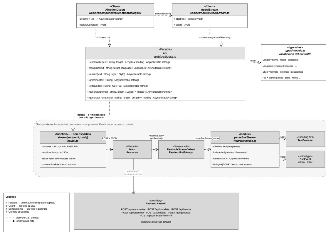
Figura 25: Diagramma della facciata di accesso al servizio applicativo
