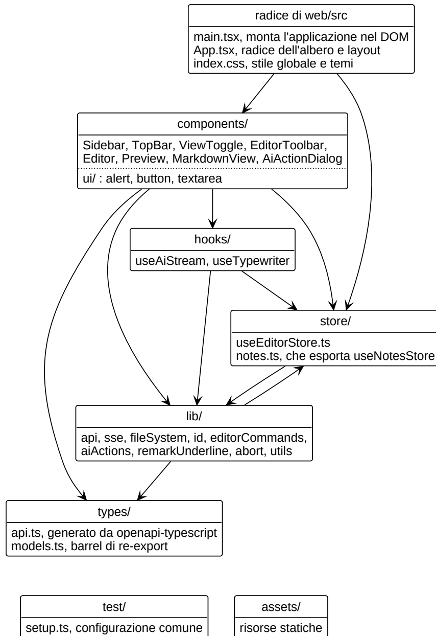
Figura 4: Diagramma UML 3.3.1 - Organizzazione per ruolo dei sorgenti in web/src
