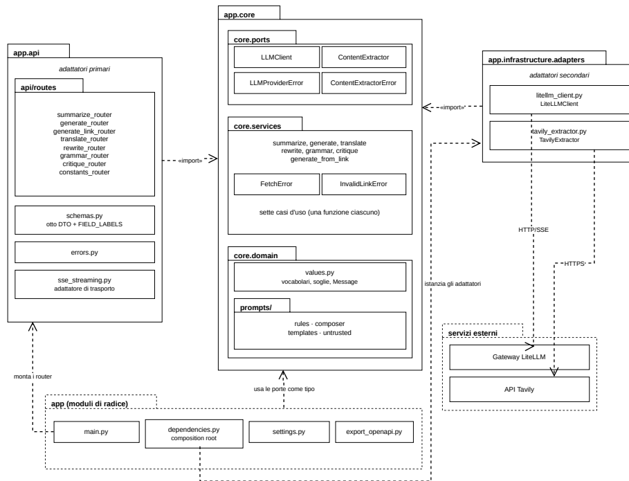
Figura 16: Architettura del servizio applicativo
