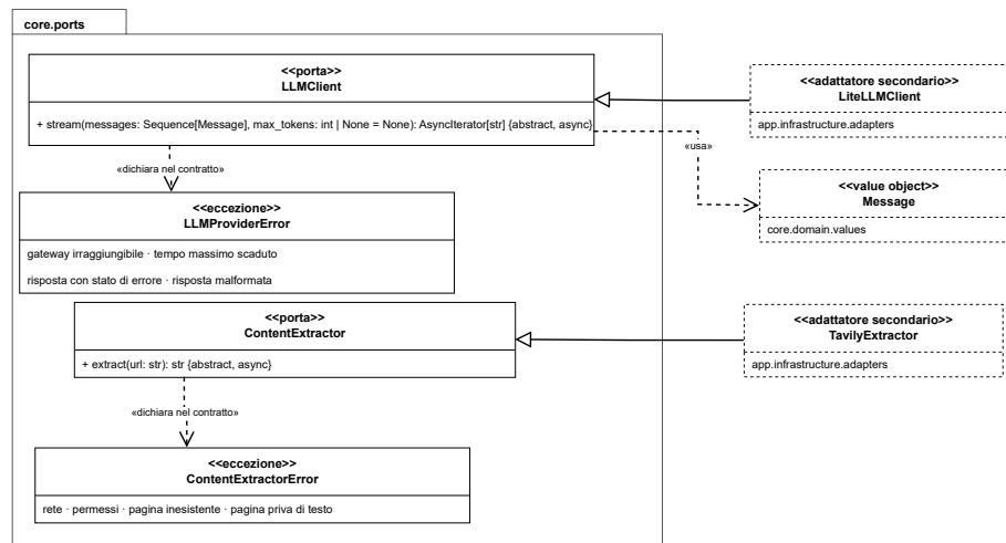
Figura 21: Le due porte e i rispettivi tipi di errore
