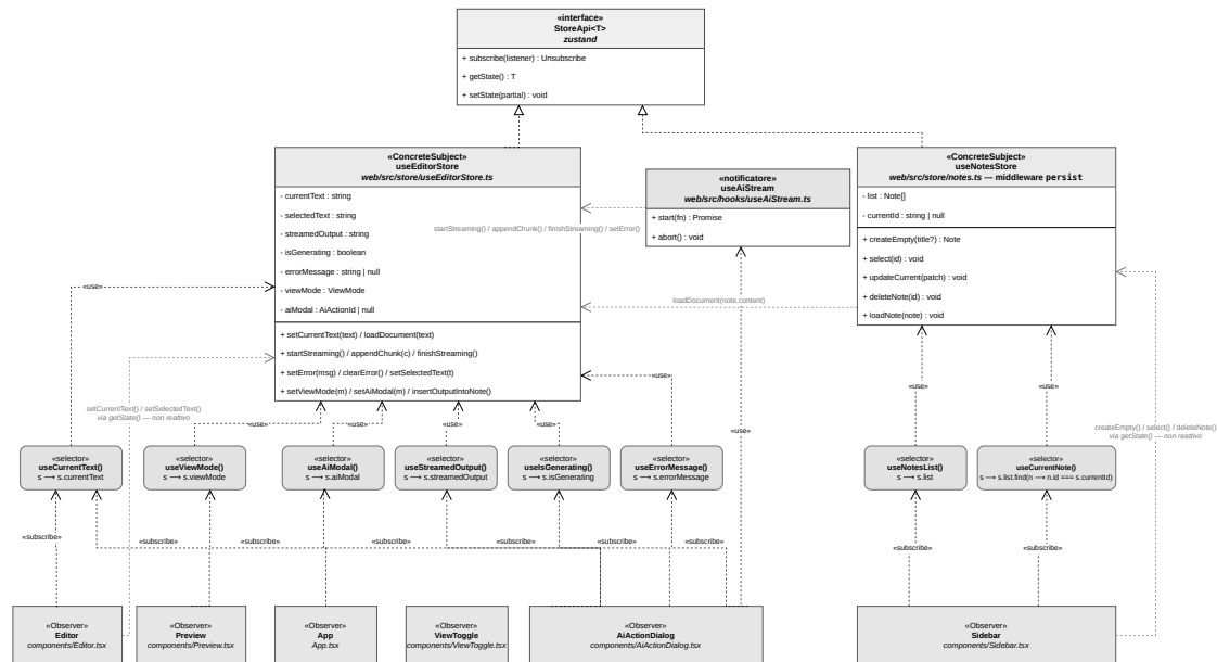
Figura 26: Diagramma soggetto-osservatori degli store e dei selettori
