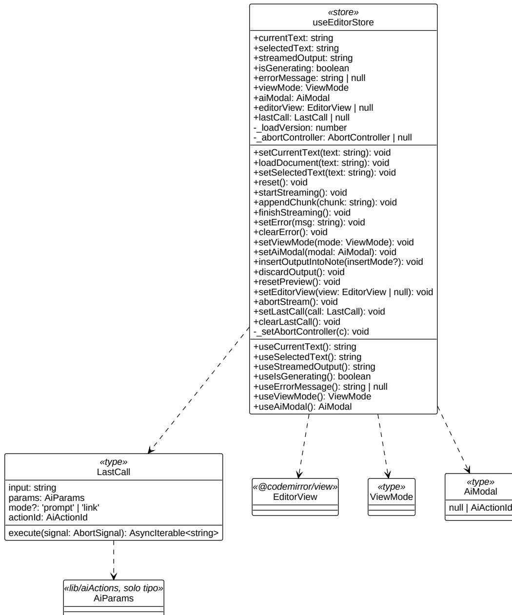
Figura 10: Diagramma UML 3.3.3-1 - useEditorStore
