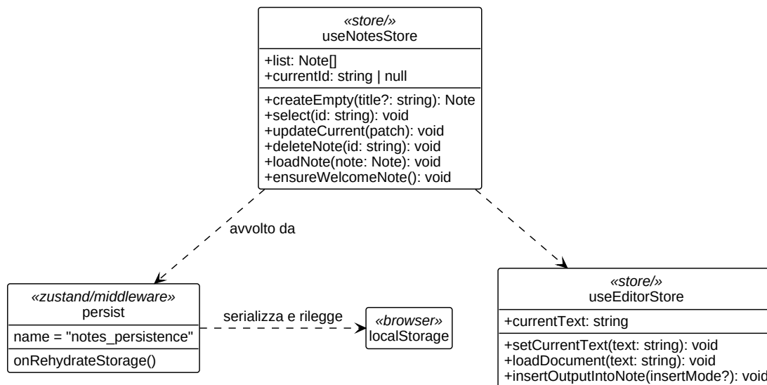
Figura 32: Diagramma UML 4.4.2-1 - La catena di persistenza dello store delle note
