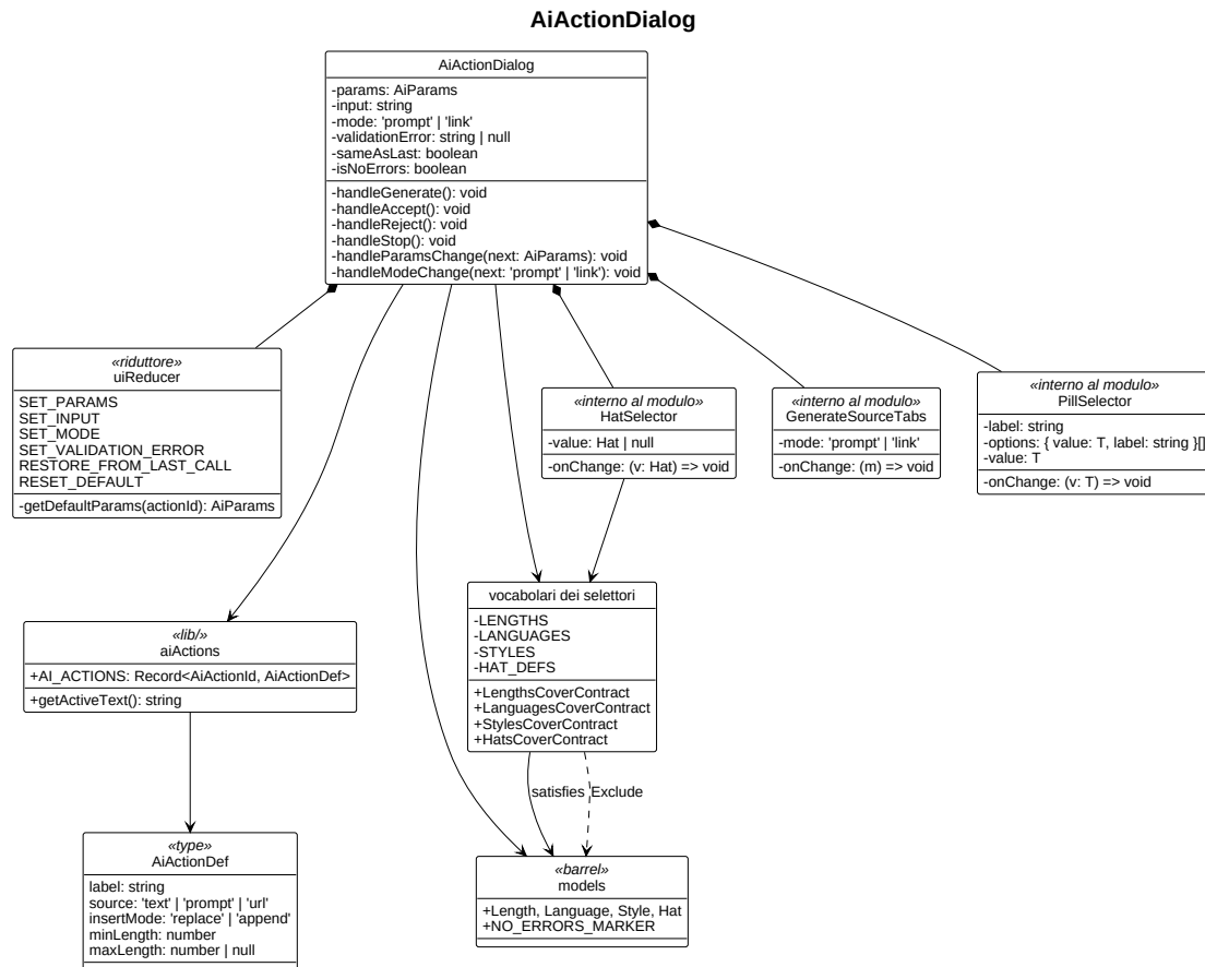
Figura 9: Diagramma UML 3.3.2-5 - AiActionDialog
