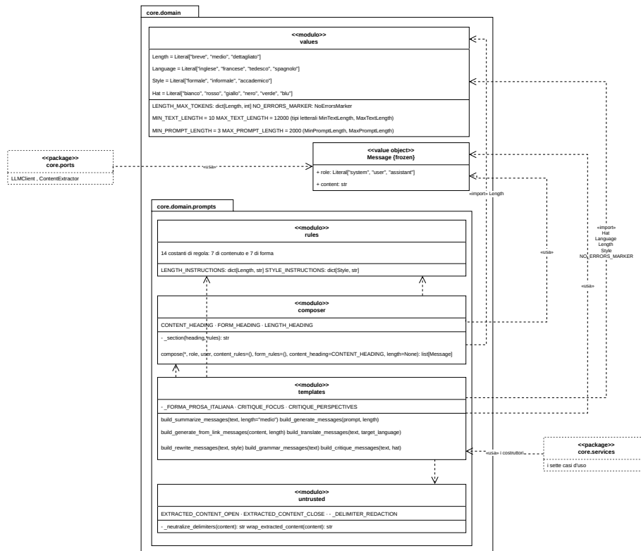
Figura 20: Valori del dominio e composizione delle istruzioni
