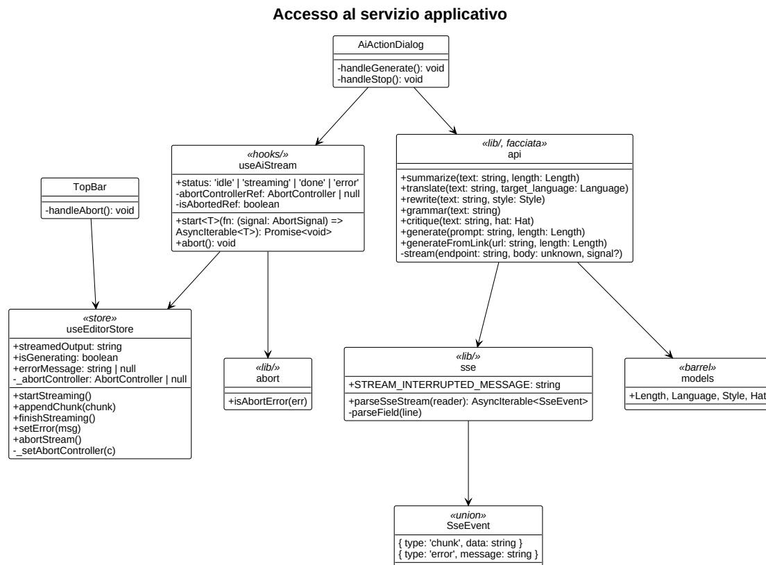
Figura 14: Diagramma UML 3.3.5 - Accesso al servizio applicativo
