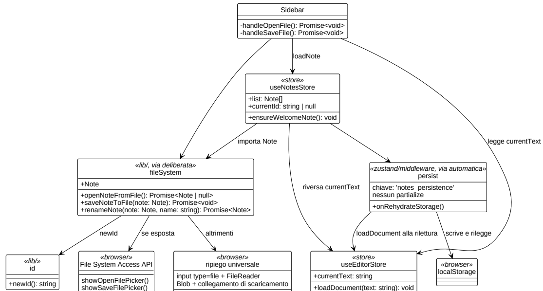
Figura 15: Diagramma UML 3.3.6 - I due meccanismi di persistenza lato client
