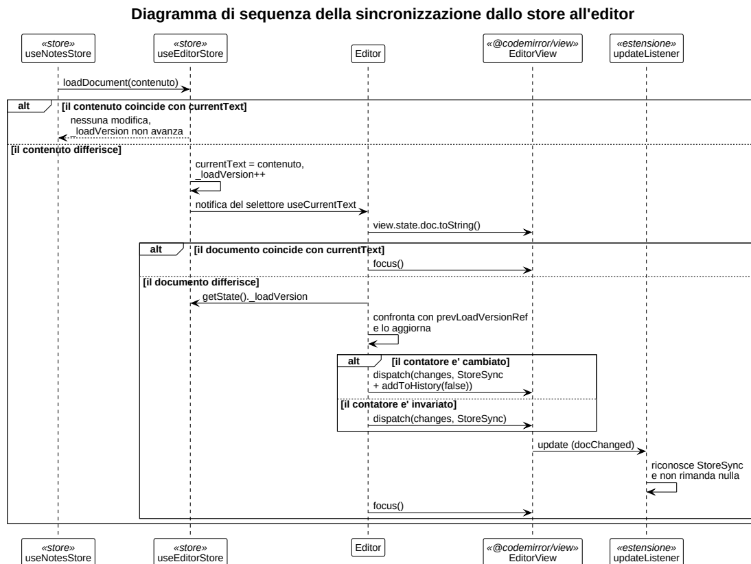
Figura 13: Diagramma UML 3.3.4-2 - Diagramma di sequenza della sincronizzazione dallo store all'editor
