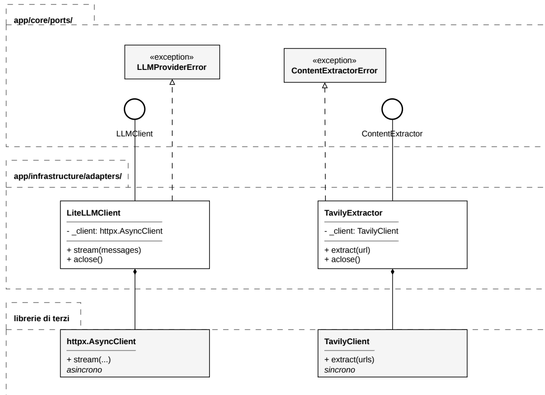
Figura 24: Diagramma delle classi dell'Object Adapter
