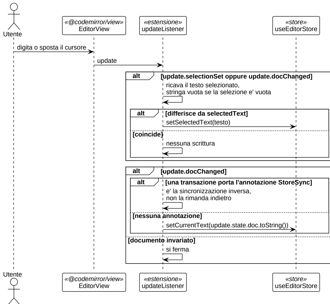
Figura 12: Diagramma UML 3.3.4-1 - Diagramma di sequenza della sincronizzazione dall'editor allo store
