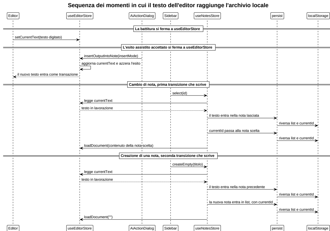
Figura 33: Diagramma UML 4.4.2-2 - Sequenza dei momenti in cui il testo dell'editor raggiunge l'archivio locale
