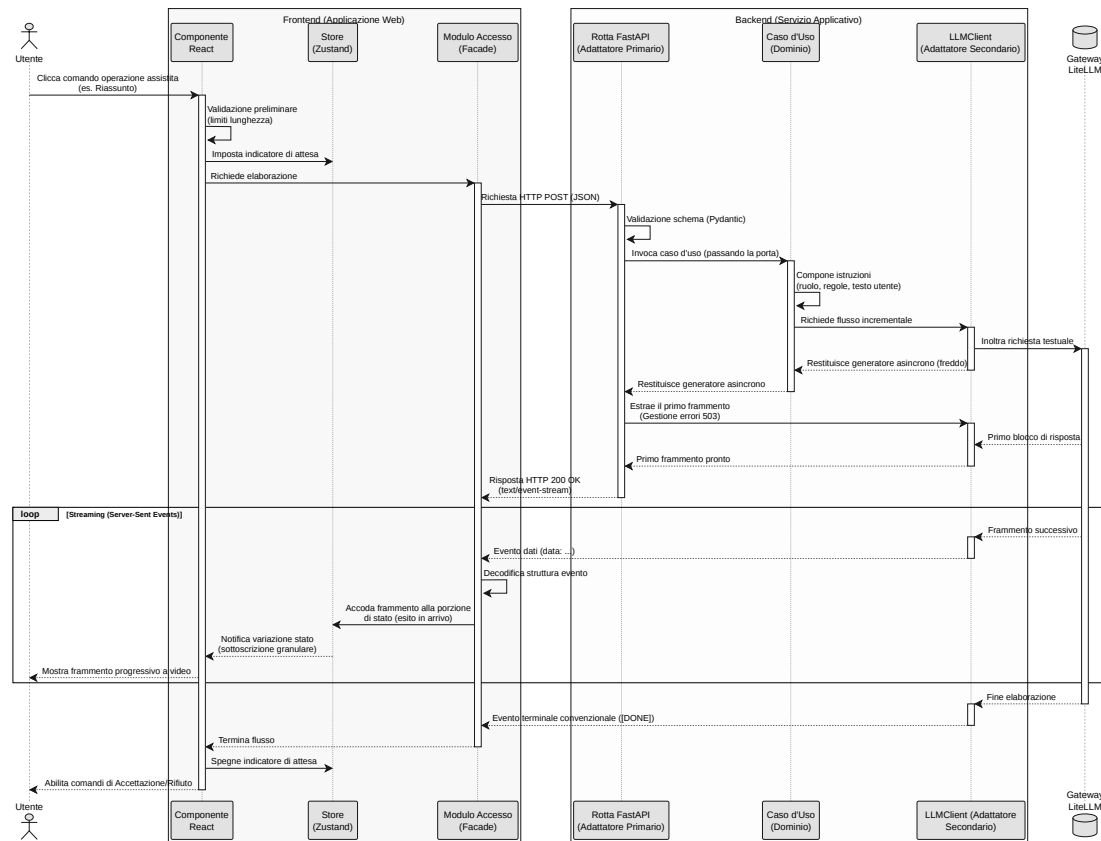
Figura 28: Diagramma di sequenza di un'operazione assistita con risposta in streaming
