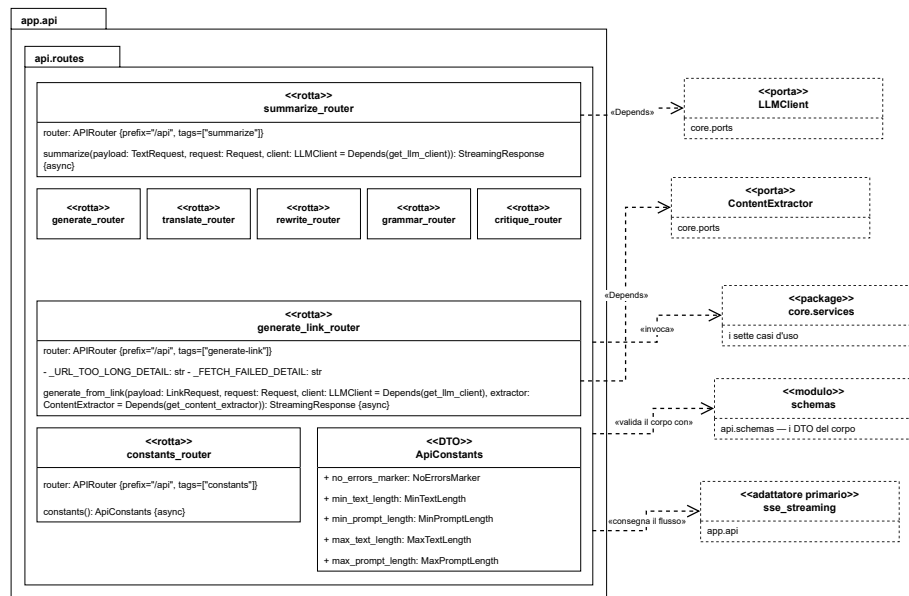
Figura 17: Le otto rotte e le loro dipendenze verso il nucleo
