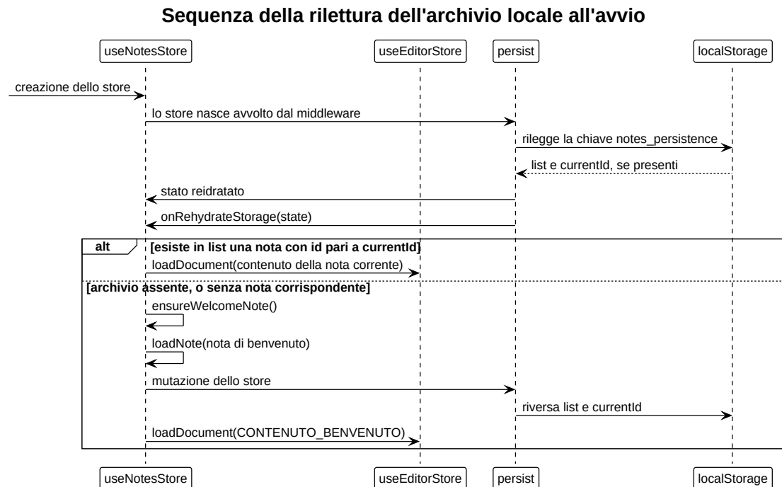
Figura 34: Diagramma UML 4.4.2-3 - Sequenza della rilettura dell'archivio locale all'avvio
