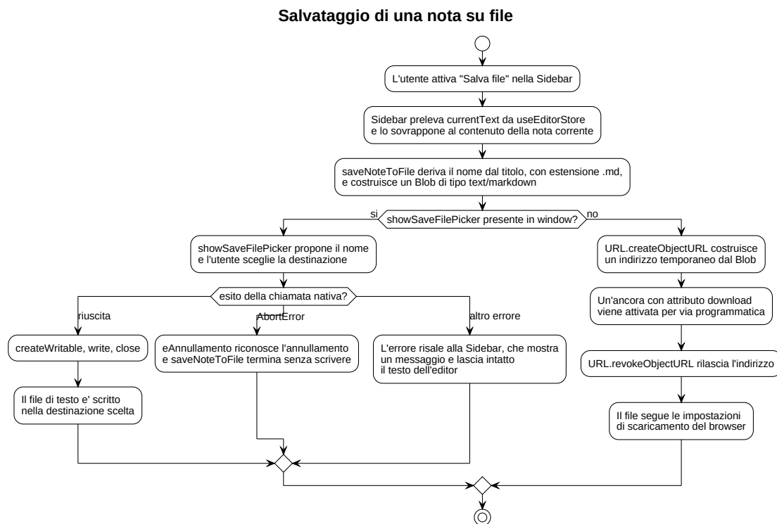
Figura 26: Diagramma UML 4.4.1-2 - Salvataggio di una nota su file
