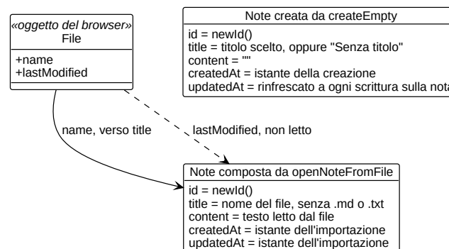
Figura 31: Diagramma UML 4.4.3 - Provenienza dei metadati per una nota creata nel prodotto e per una importata da file
