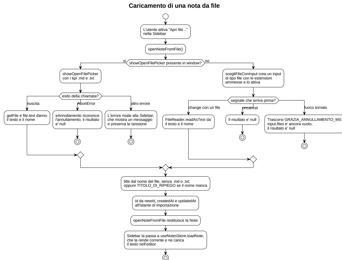
Figura 27: Diagramma UML 4.4.1-3 - Caricamento di una nota da file
