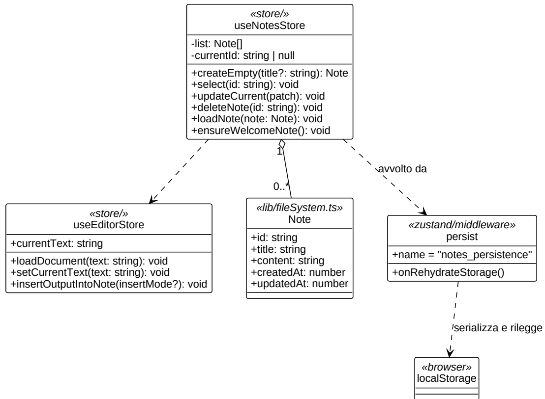
Figura 28: Diagramma UML 4.4.2-1 - La catena di persistenza dello store delle note
