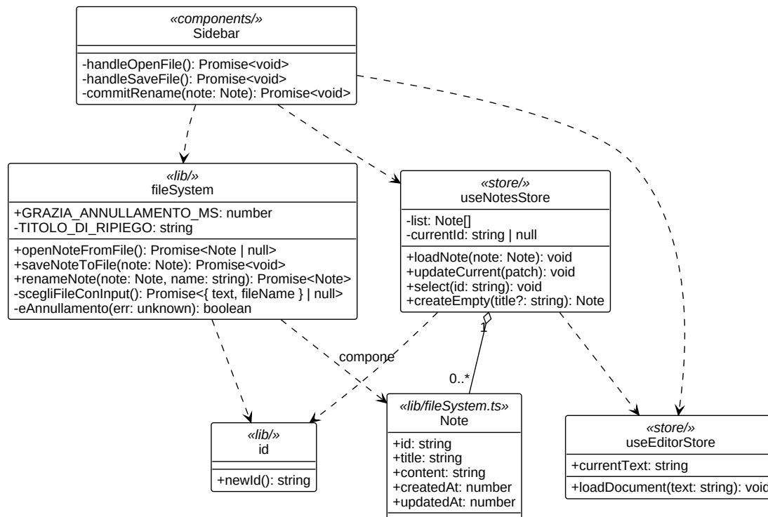
Figura 25: Diagramma UML 4.4.1-1 - Il modulo lib/fileSystem.ts e le sue dipendenze
