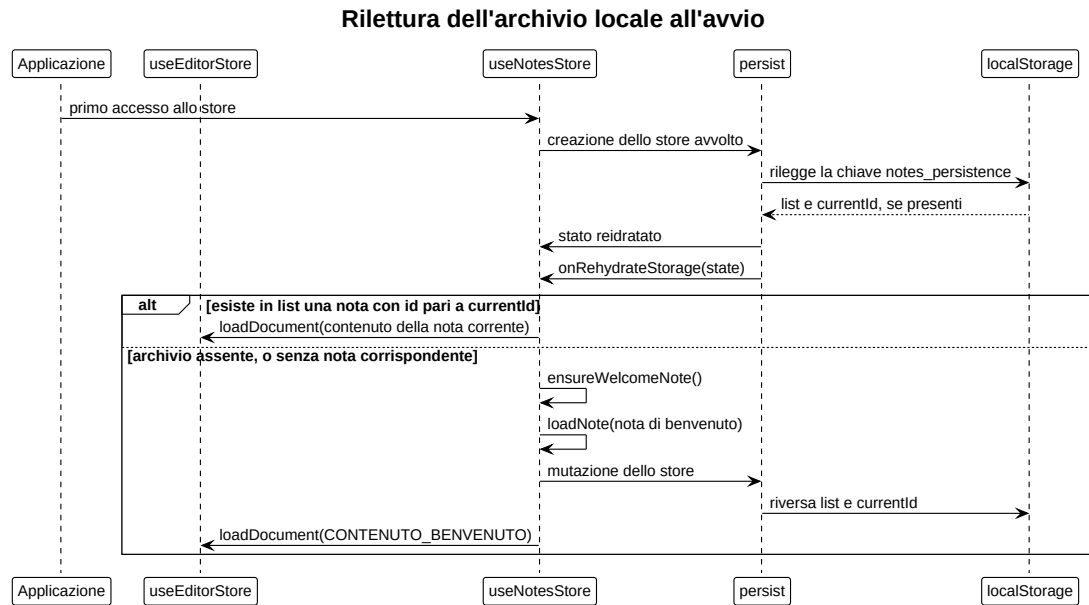
Figura 30: Diagramma UML 4.4.2-3 - Rilettura dell'archivio locale all'avvio
