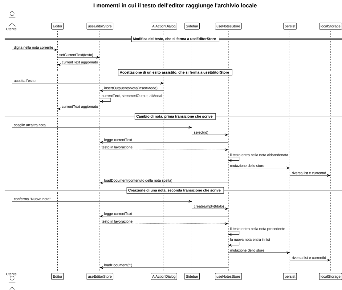
Figura 29: Diagramma UML 4.4.2-2 - I momenti in cui il testo dell'editor raggiunge l'archivio locale
