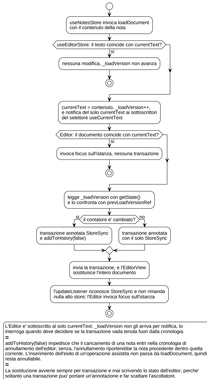
Figura 16: Diagramma UML 3.3.4-2 - Sincronizzazione store → editor
