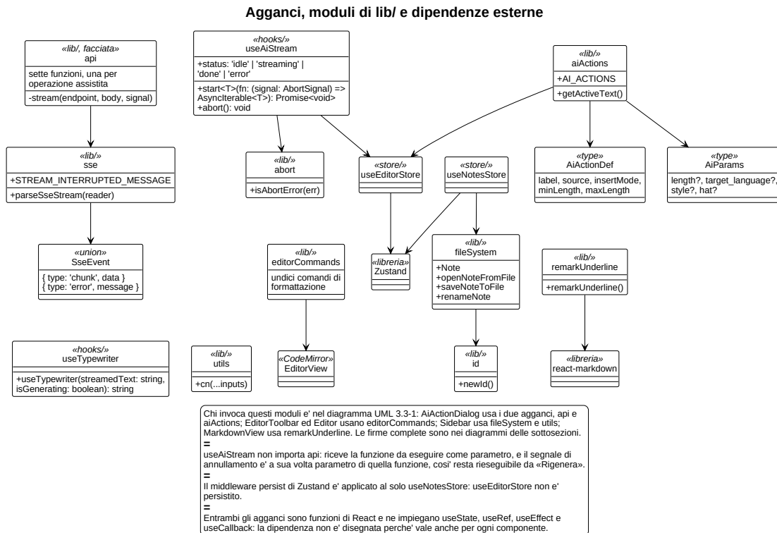
Figura 3: Diagramma UML 3.3-2 - Hooks, Librerie e Dipendenze Esterne
