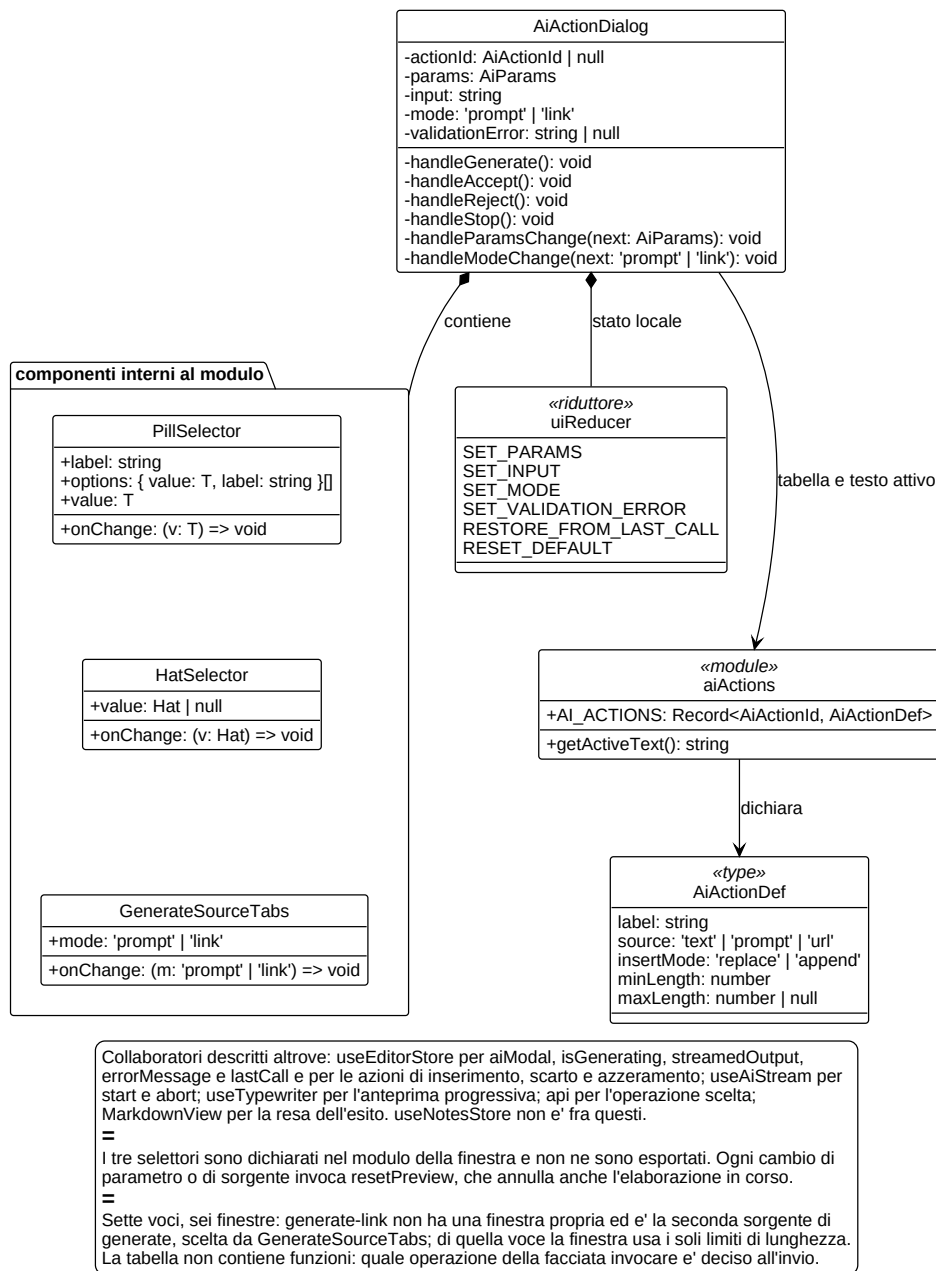
Figura 12: Diagramma UML 3.3.2-8 - AiActionDialog
