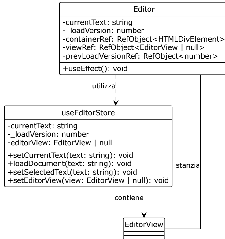
Figura 8: figura: Diagramma UML 3.3.2-5 - Editor
