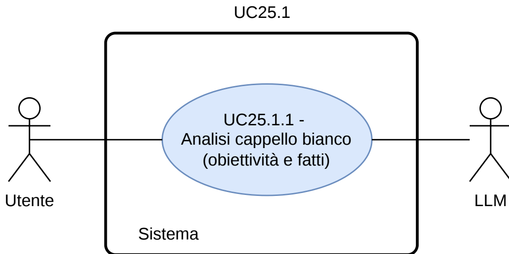
Figura 89: Diagramma UC25.1.1
