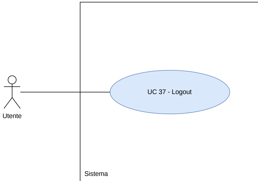
Figura 142: Diagramma UC37
