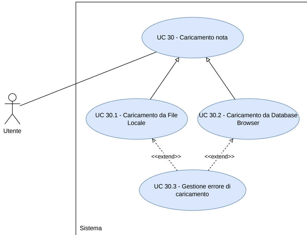
Figura 116: Diagramma UC30
