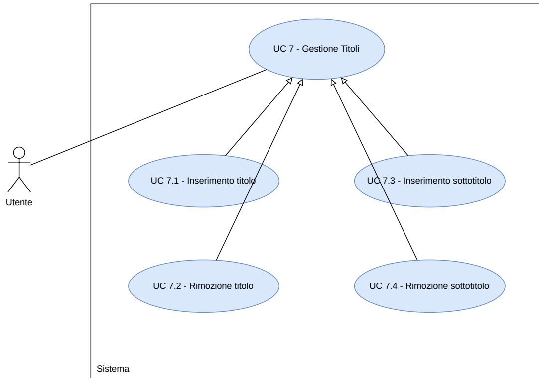
Figura 23: Diagramma UC7
