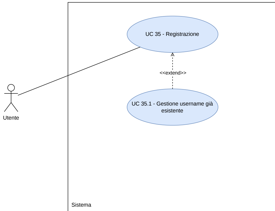
Figura 139: Diagramma UC35
