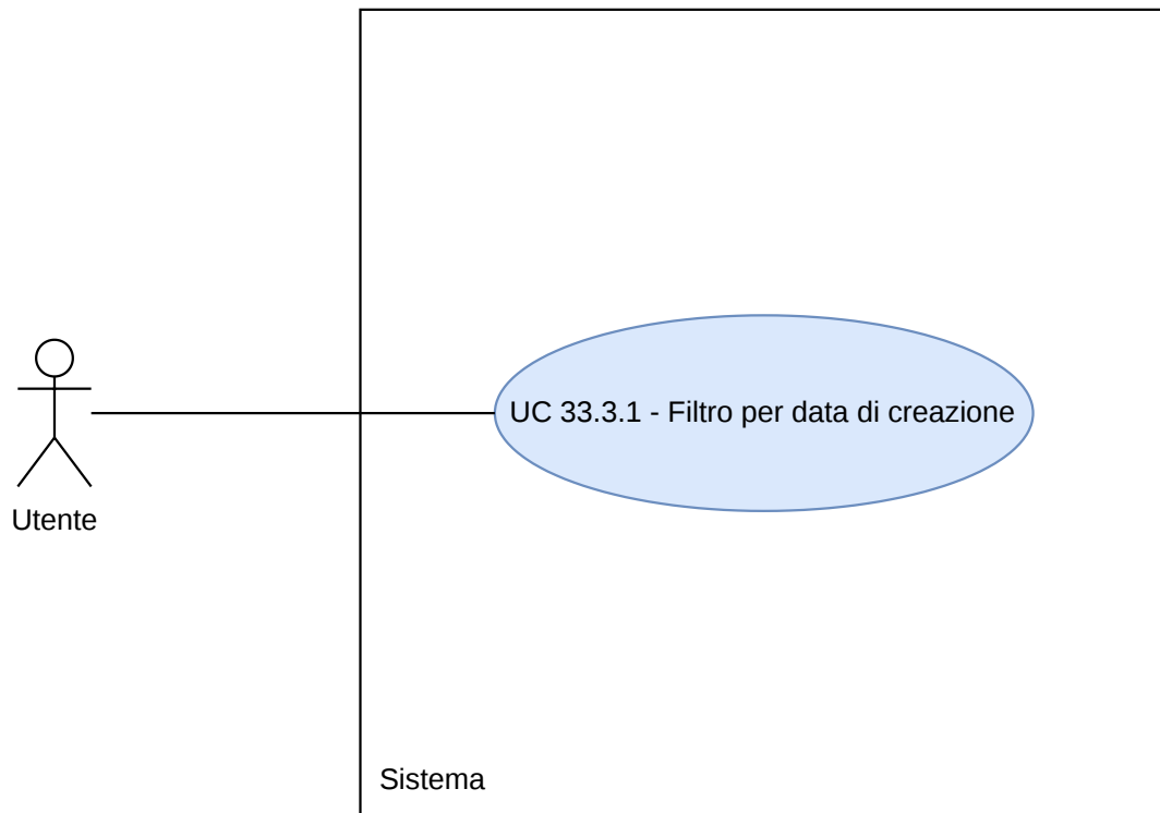
Figura 134: Diagramma UC33.3.1
