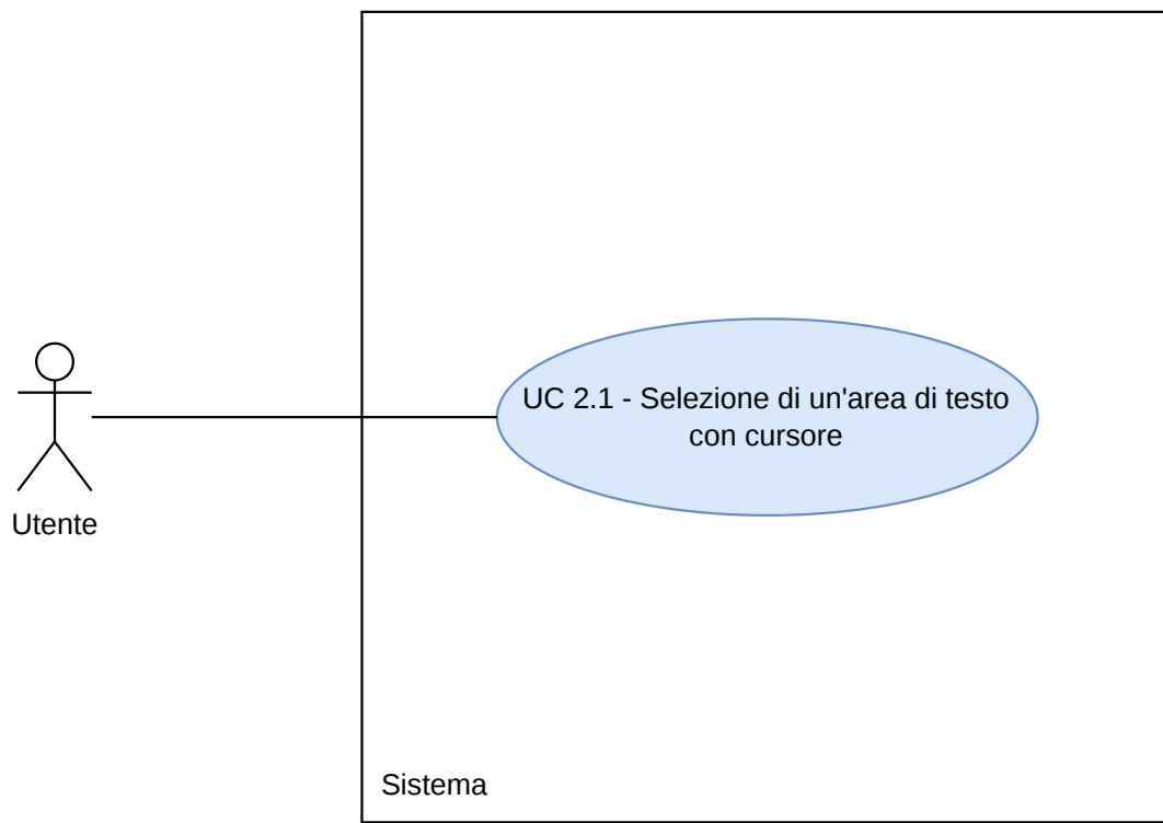
Figura 4: Diagramma UC2.1
