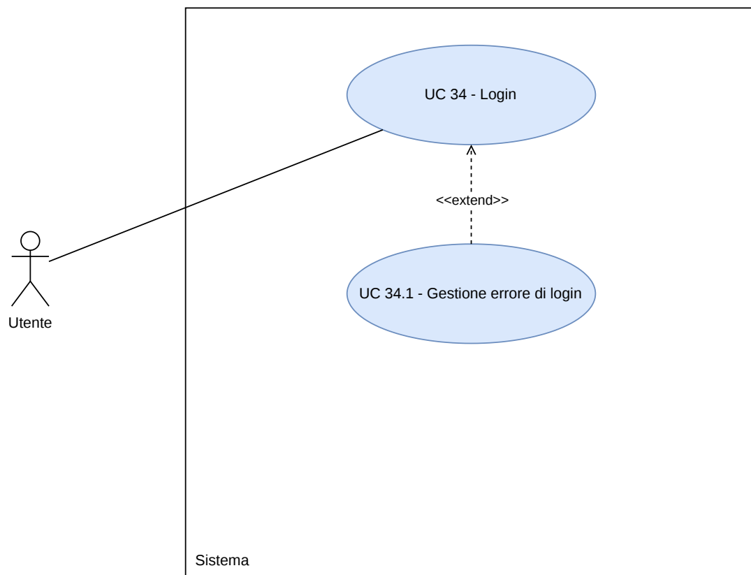
Figura 137: Diagramma UC34
