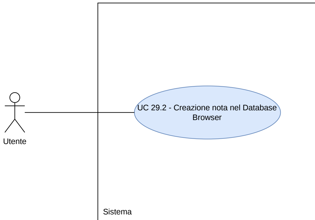
Figura 114: Diagramma UC29.2
