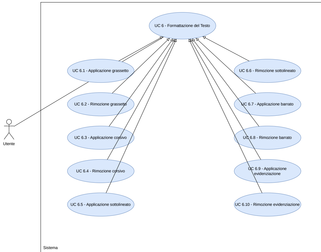
Figura 12: Diagramma UC6
