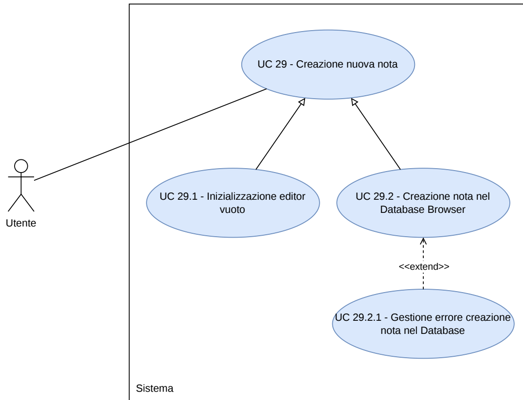
Figura 112: Diagramma UC29
