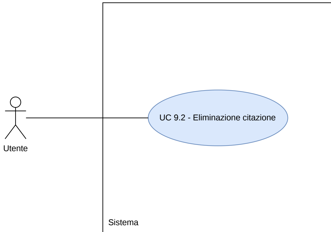
Figura 33: Diagramma UC9.2
