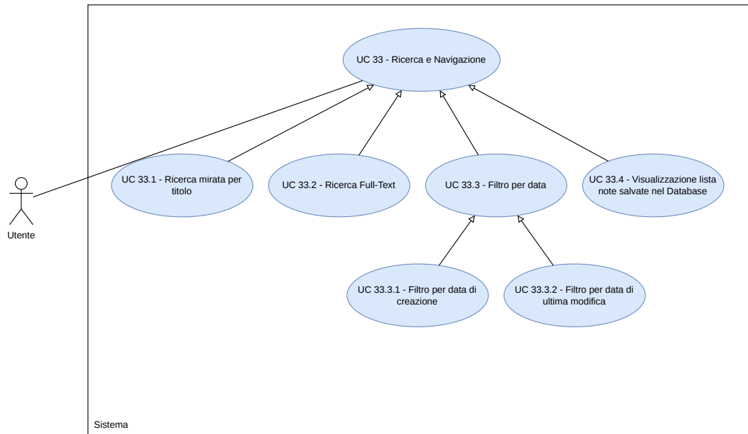
Figura 130: Diagramma UC33
