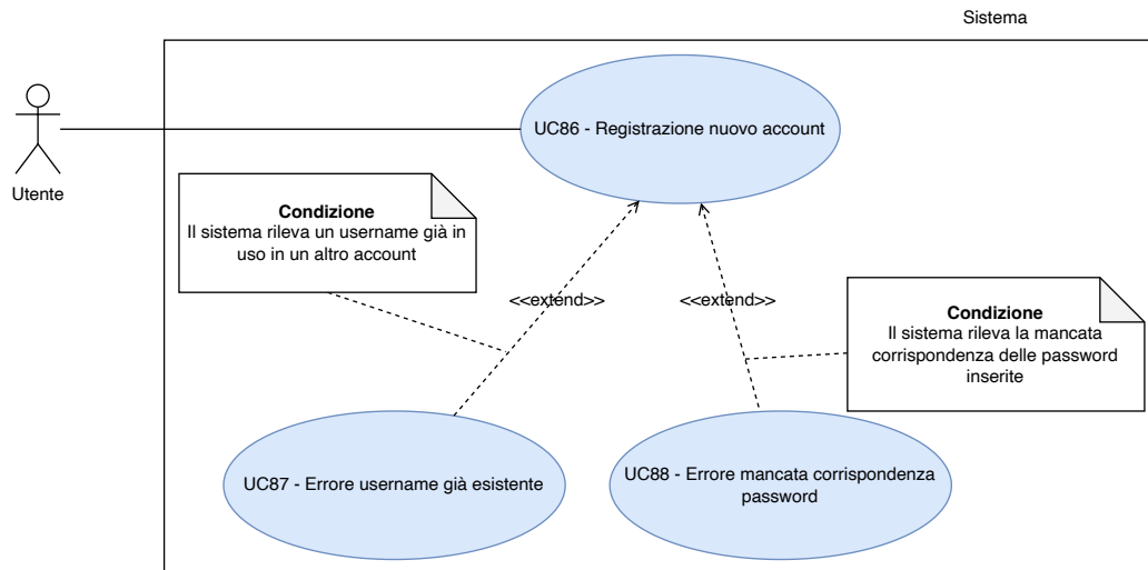
Figura 86: UC 86 -Registrazione nuovo account
