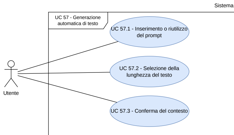
Figura 64: UC 57.1, UC 57.2, UC 57.3 - Inclusioni di UC 57
