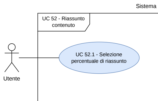
Figura 55: Inclusione del Caso d'Uso n.52: UC 52.1
