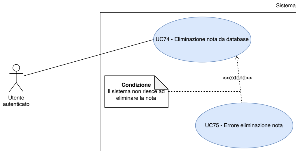
Figura 76: UC 74 - Eliminazione nota da database
