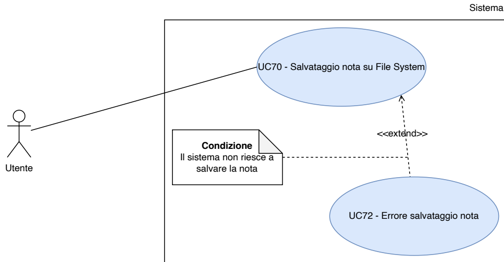
Figura 73: UC 70 - Salvataggio nota su File System
