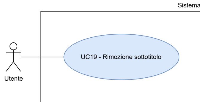
Figura 20: UC19 - Rimozione sottotitolo
