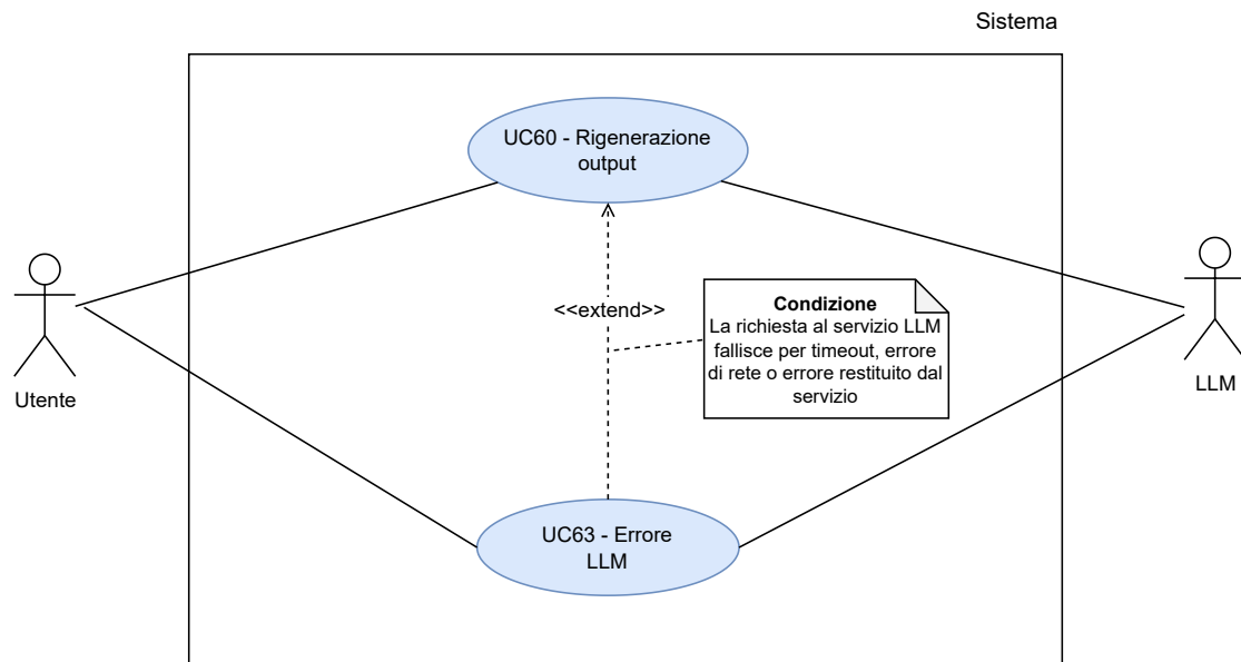
Figura 67: UC60 - Rigenerazione output
