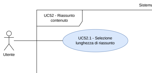
Figura 56: UC52.1 - Inclusione di UC52
