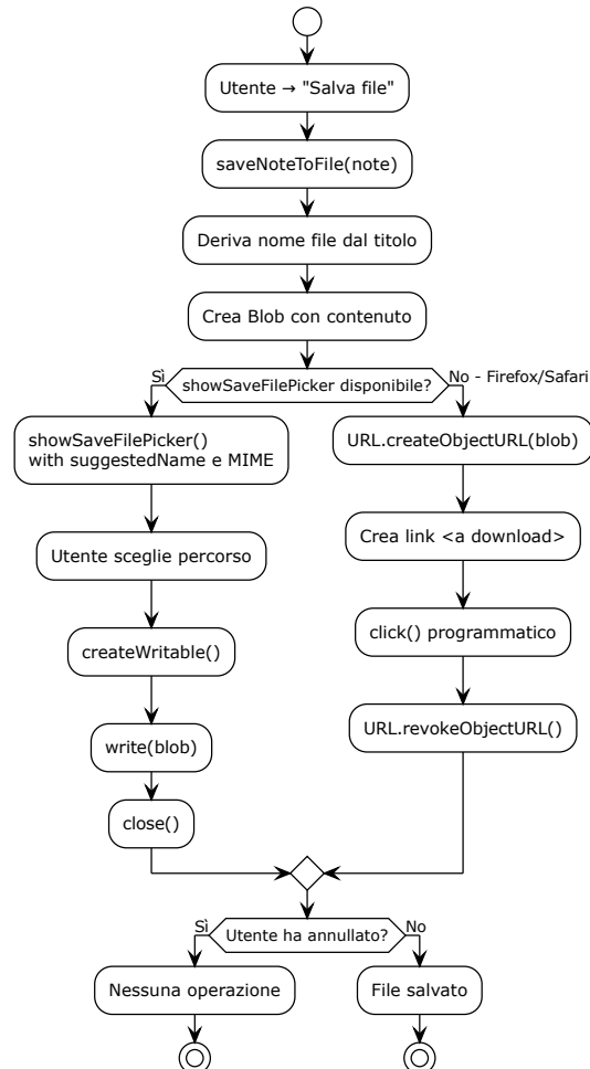
Figura 25: Diagramma UML 4.4.1-1 - fileSystem
