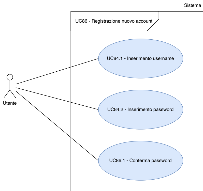
Figura 88: UC 84.1, UC 84.2, UC 86.1 - Inclusioni di UC 86
