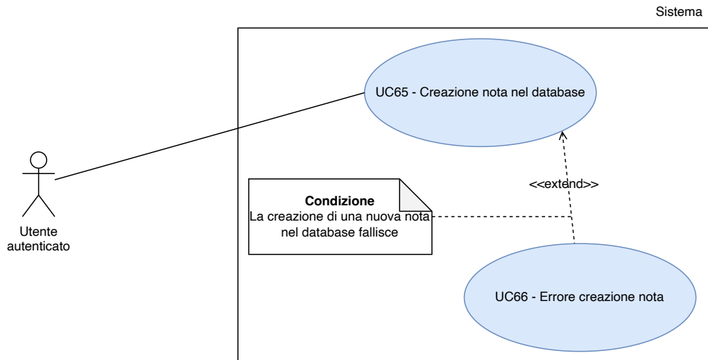
Figura 71: UC 65 - Creazione nota nel database
