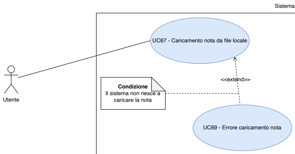
Figura 72: UC 67 - Caricamento nota da file locale
