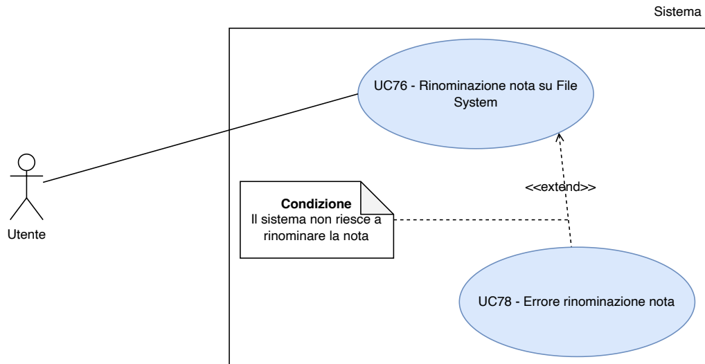
Figura 78: UC 76 - Rinominazione nota su File System
