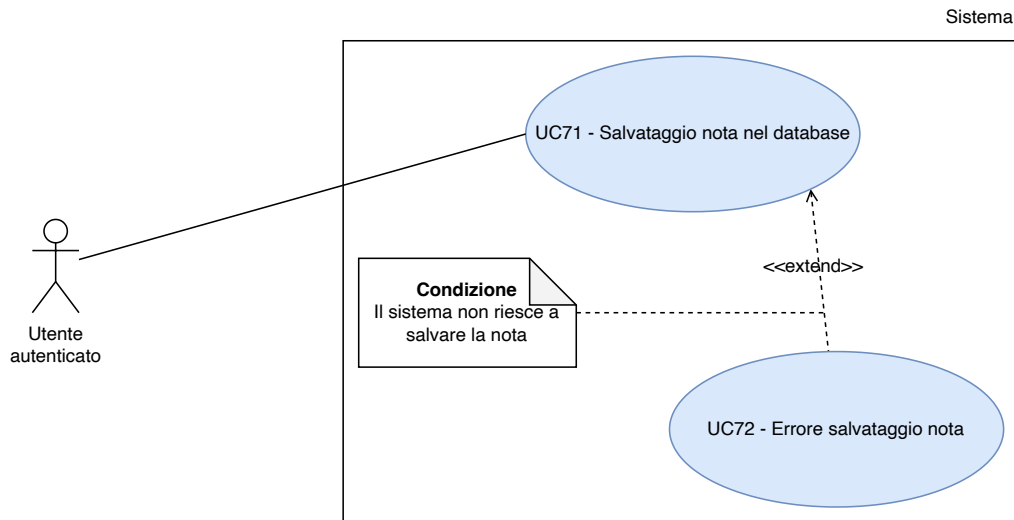
Figura 75: UC 71 - Salvataggio nota nel database
