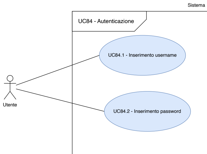
Figura 86: UC 84.1, UC 84.2 - Inclusioni di UC 84
