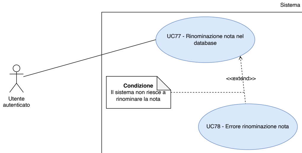
Figura 79: UC 77 - Rinominazione nota nel database
