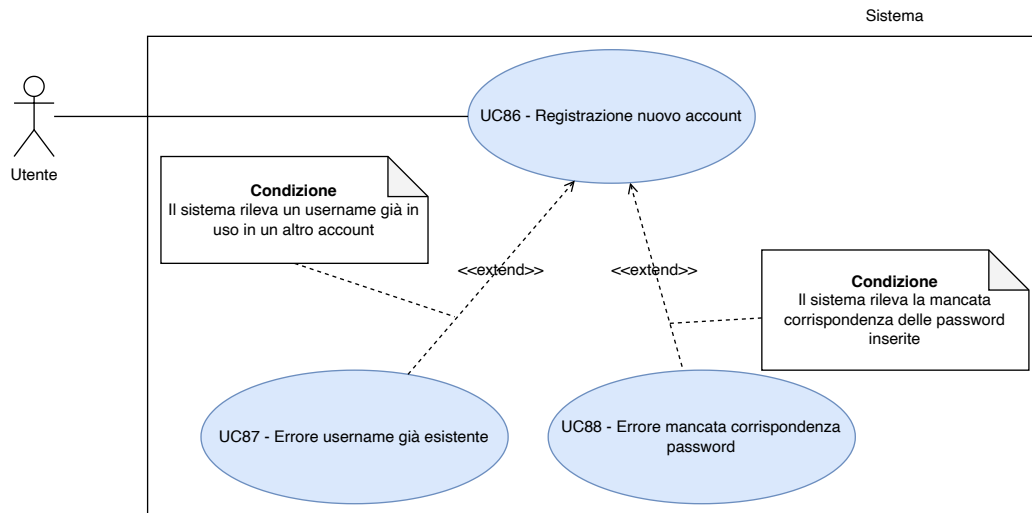
Figura 87: UC 86 -Registrazione nuovo account
