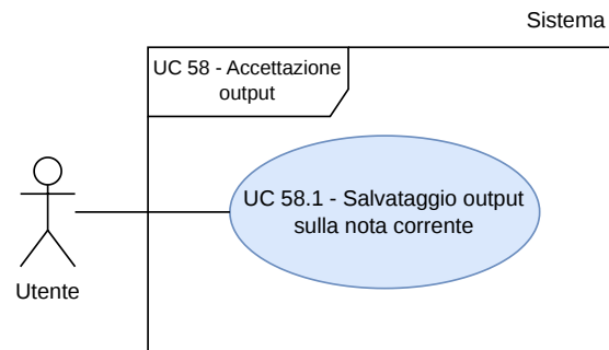
Figura 67: UC 58.1 - Inclusione di UC 58
