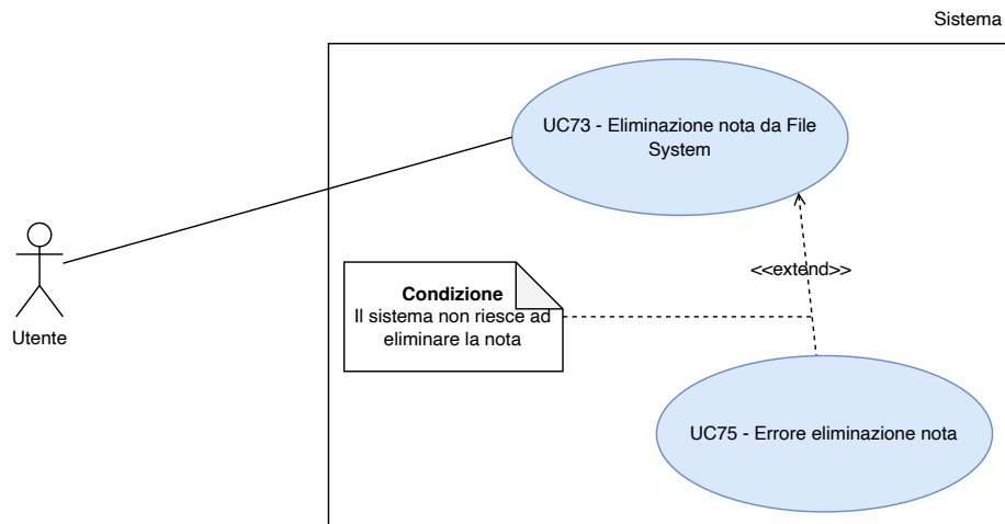
Figura 76: UC 73 - Eliminazione nota da File System
