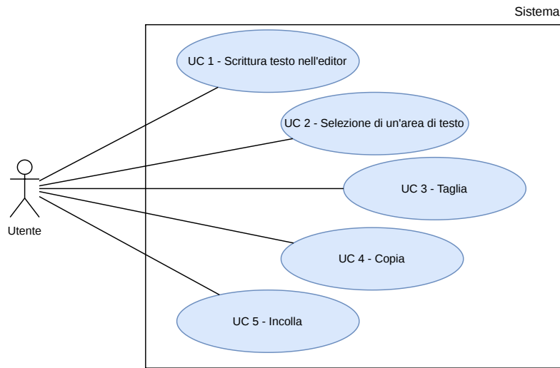
Figura 2: UC 1-5 - Scrittura, selezione del testo, taglia, copia e incolla
