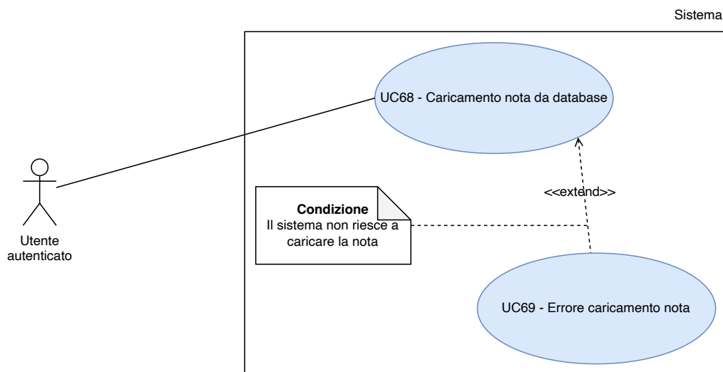
Figura 24: UC 68 - Caricamento nota da database
