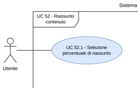
Figura 15: Inclusione del Caso d'Uso n.52: UC 52.1
