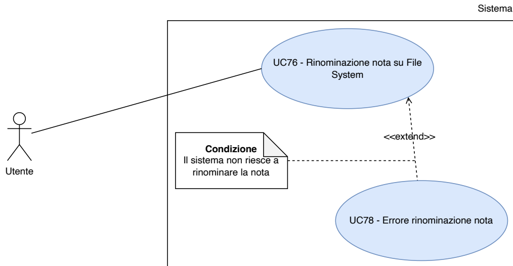
Figura 29: UC 76 - Rinominazione nota su File System
