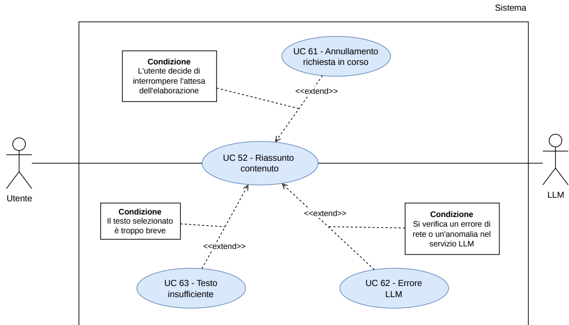
Figura 14: UC 52 - Riassunto Contenuto
