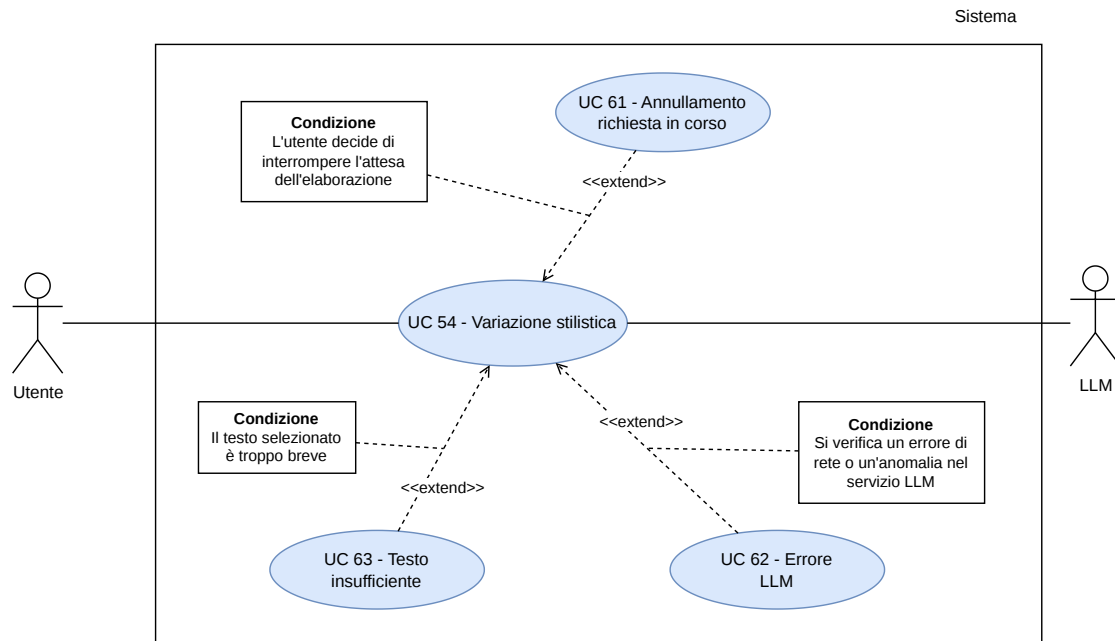
Figura 18: UC 54 - Variazione Stilistica
