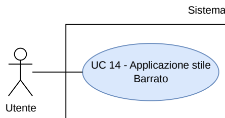
Figura 13: UC 14 - Applicazione stile Barrato
