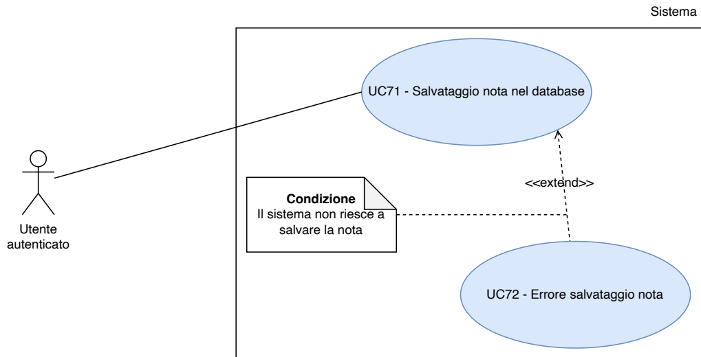
Figura 26: UC 71 - Salvataggio nota nel database
