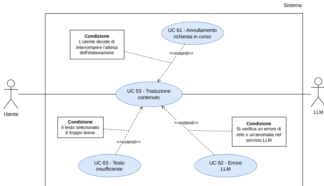
Figura 16: UC 53 - Traduzione Contenuto
