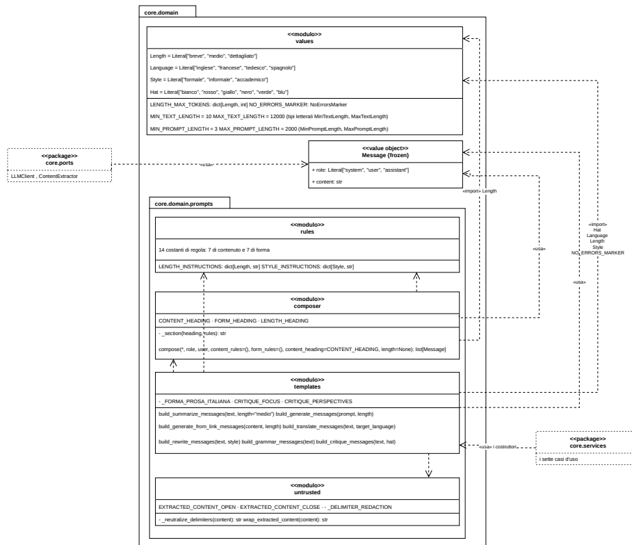
Figura 23: Valori del dominio e composizione delle istruzioni
