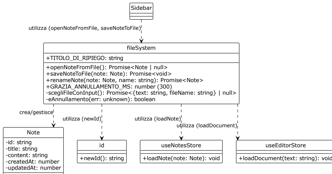
Figura 38: Diagramma UML 4.4.3 - nota creata nel prodotto vs nota importata da disco
