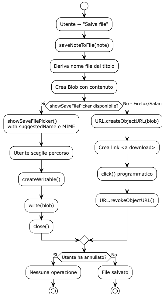
Figura 32: Diagramma UML 4.4.1-1 - fileSystem
