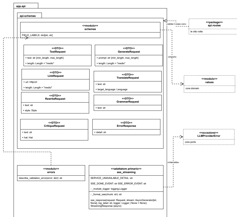
Figura 21: Schemi di validazione, traduzione degli errori e adattatore di trasporto
