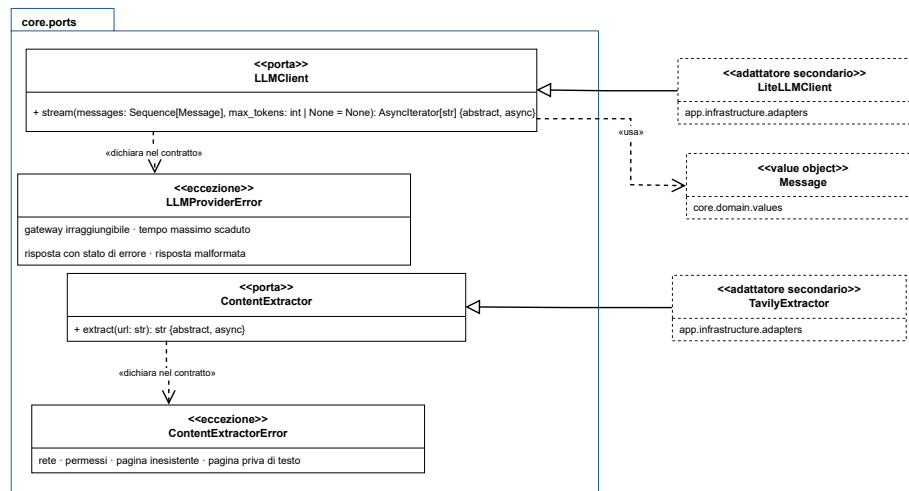
Figura 24: Le due porte e i rispettivi tipi di errore
