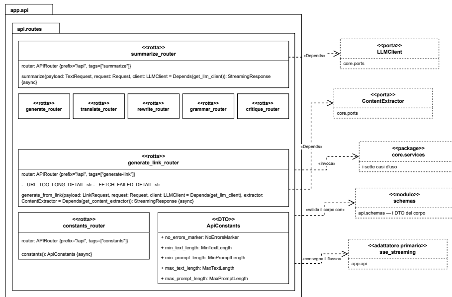
Figura 20: Le otto rotte e le loro dipendenze verso il nucleo
