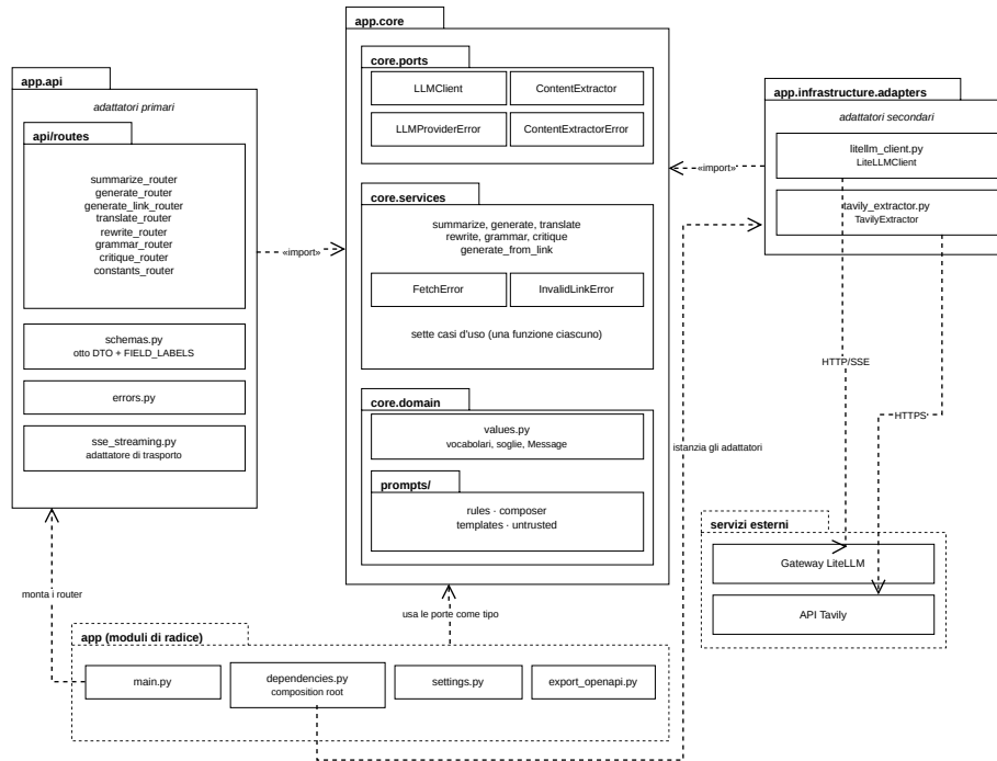
Figura 19: Architettura del servizio applicativo
