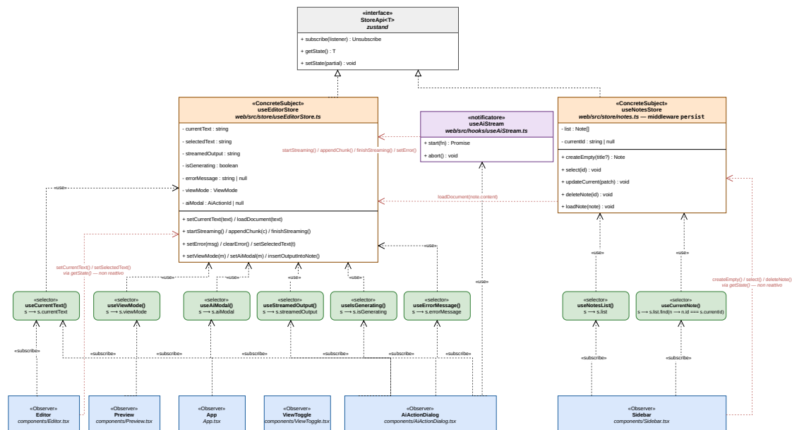
Figura 29: Diagramma soggetto-osservatori degli store e dei selettori
