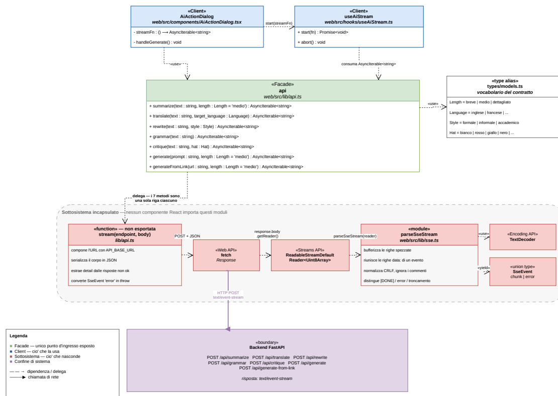
Figura 28: Diagramma della facciata di accesso al servizio applicativo
