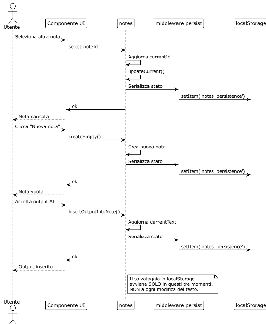
Figura 35: Diagramma UML 4.4.2-1 - salvataggio automatico in localStorage
