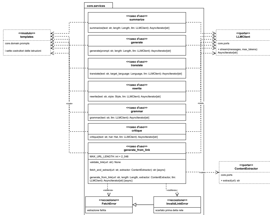
Figura 22: I sette casi d'uso e le dipendenze verso le porte
