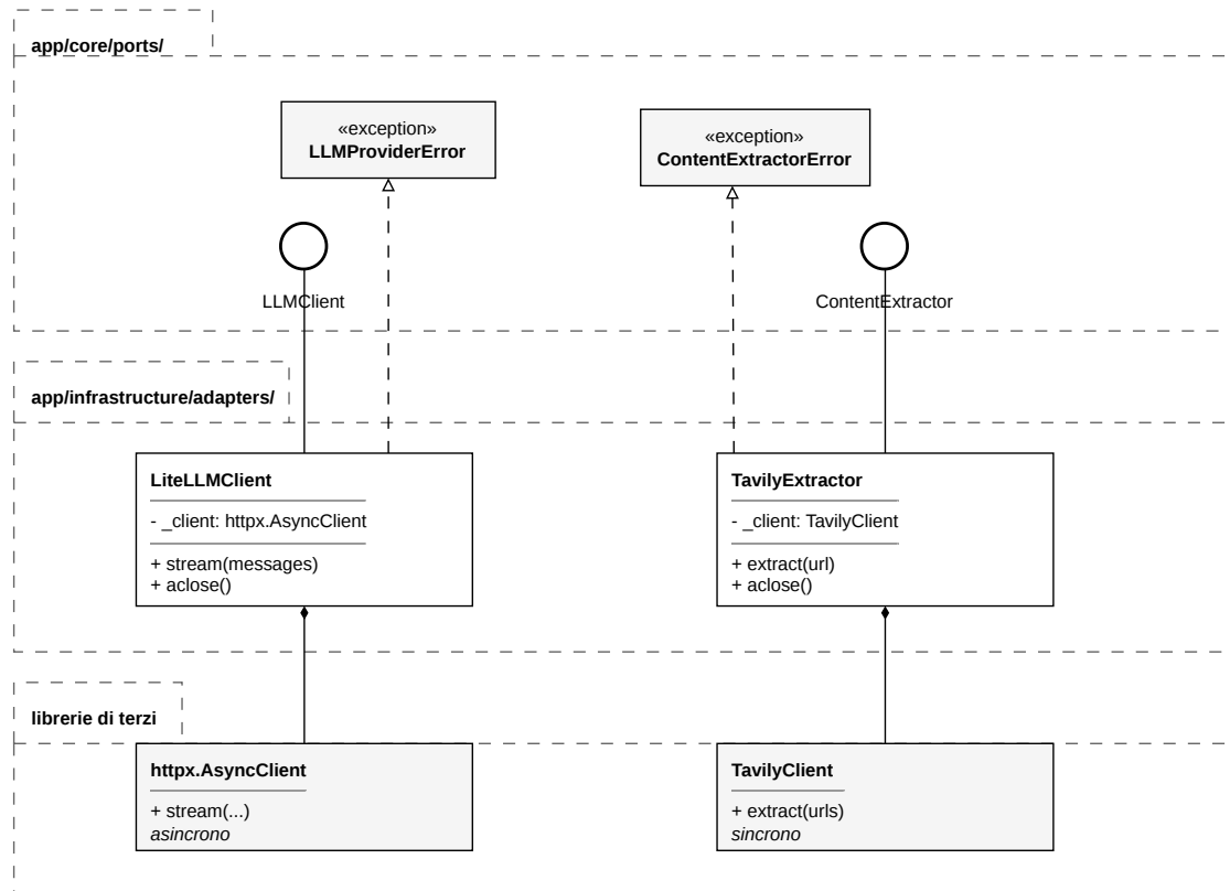
Figura 27: Diagramma delle classi dell'Object Adapter
