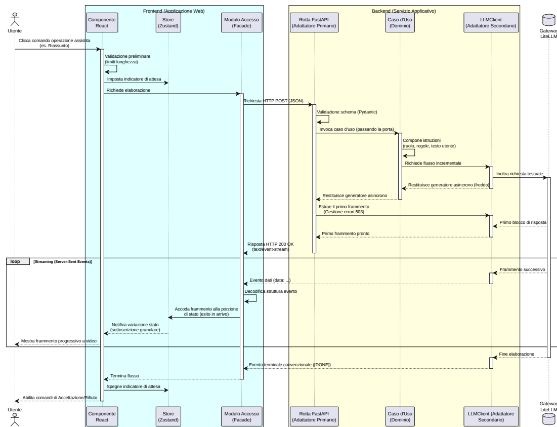
Figura 31: Diagramma di sequenza di un'operazione assistita con risposta in streaming
