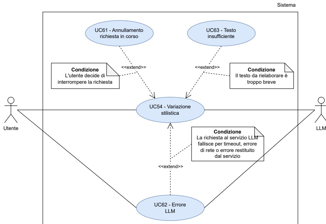
Figura 58: UC54 - Variazione Stilistica
