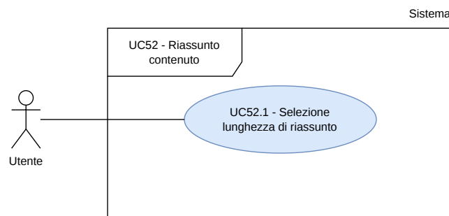
Figura 55: UC52.1 - Inclusione di UC52
