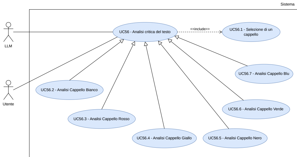
Figura 62: UC56.1, 56.2, 56.3, 56.4, 56.5, 56.6, 56.7 - Inclusione di UC56 e generalizzazioni
