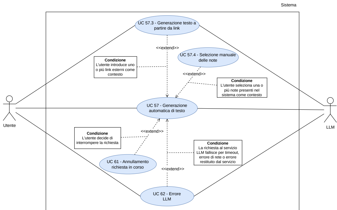
Figura 63: UC57 - Generazione automatica di testo
