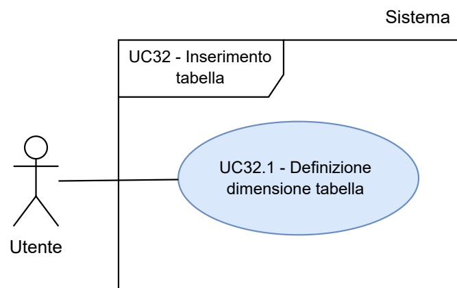
Figura 35: UC32.1 - Inclusione di UC32
