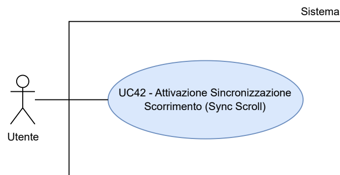
Figura 44: UC42 - Attivazione Sincronizzazione Scorrimento (Sync Scroll)
