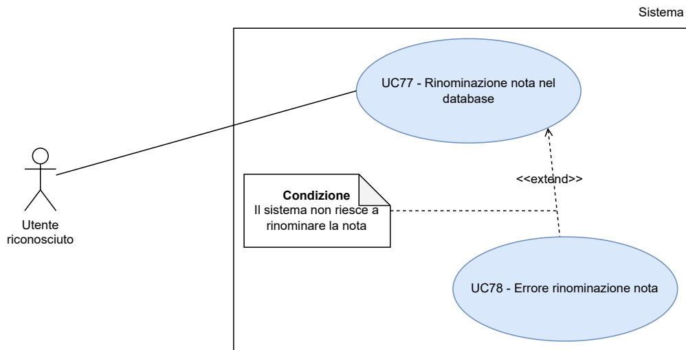
Figura 77: UC77 - Rinominazione nota nel database
