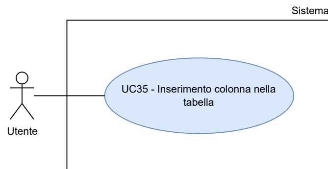
Figura 38: UC35 - Inserimento colonna nella tabella
