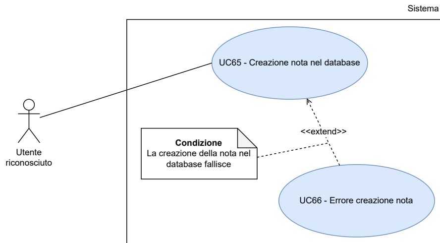
Figura 69: UC65 - Creazione nota nel database
