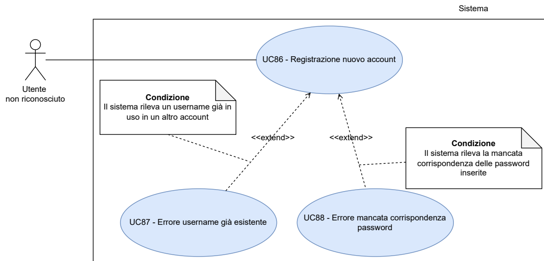
Figura 85: UC86 - Registrazione nuovo account
