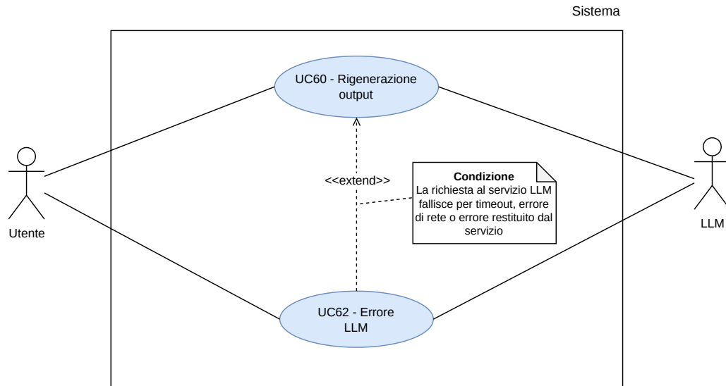
Figura 67: UC60 - Rigenerazione output
