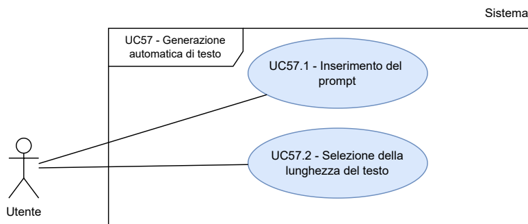
Figura 64: UC57.1, UC57.2 - Inclusioni di UC57
