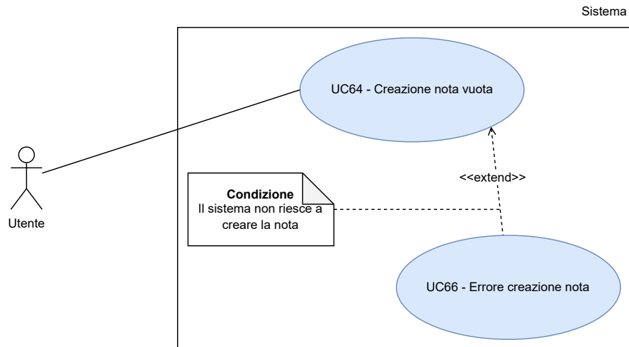
Figura 68: UC64 - Creazione nota vuota
