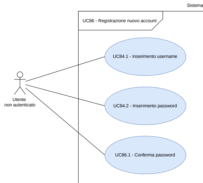
Figura 86: UC84.1, UC84.2, UC86.1 - Inclusioni di UC86
