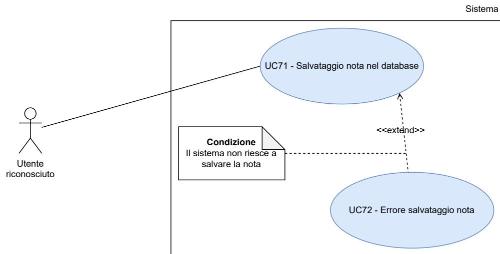
Figura 73: UC71 - Salvataggio nota nel database
