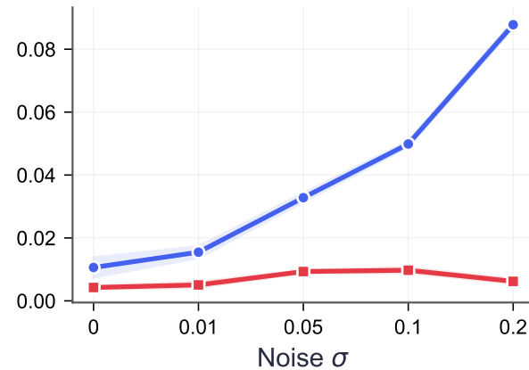
Linear 5D
