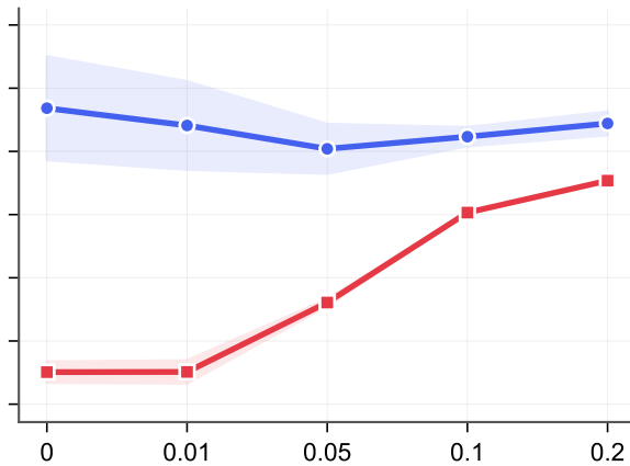
Linear 5D
