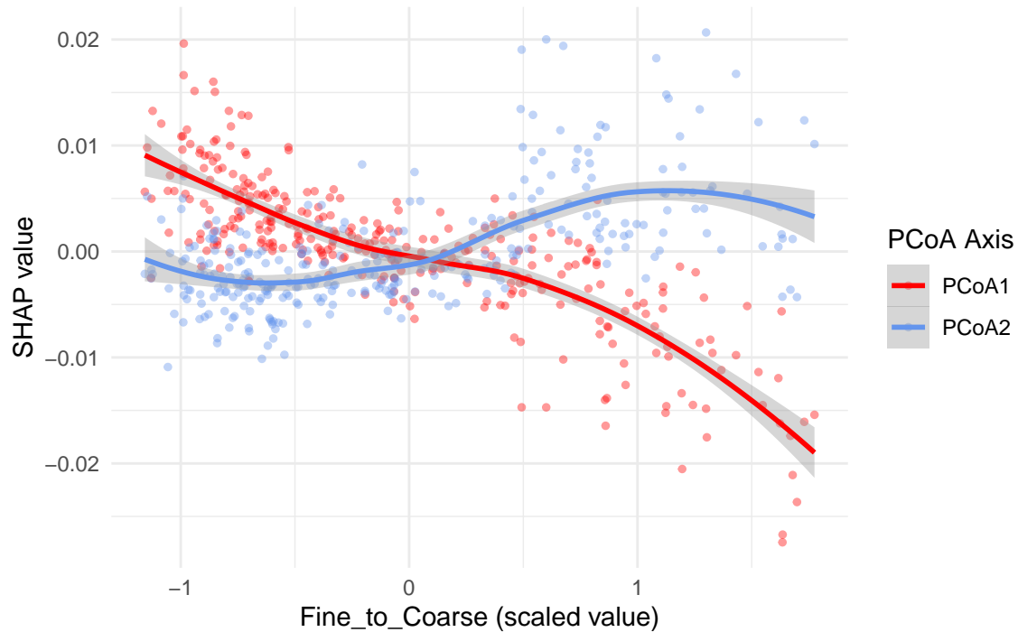
SHAP Values vs Scaled Fine_to_Coarse
