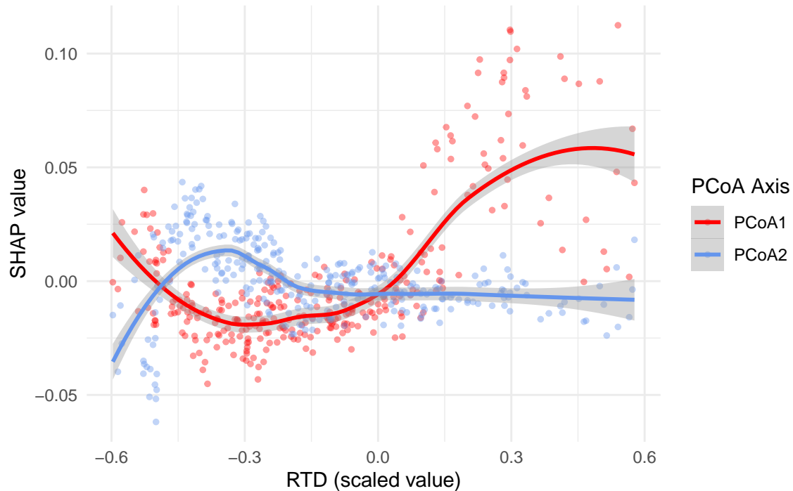
SHAP Values vs Scaled RTD (Fungi)
