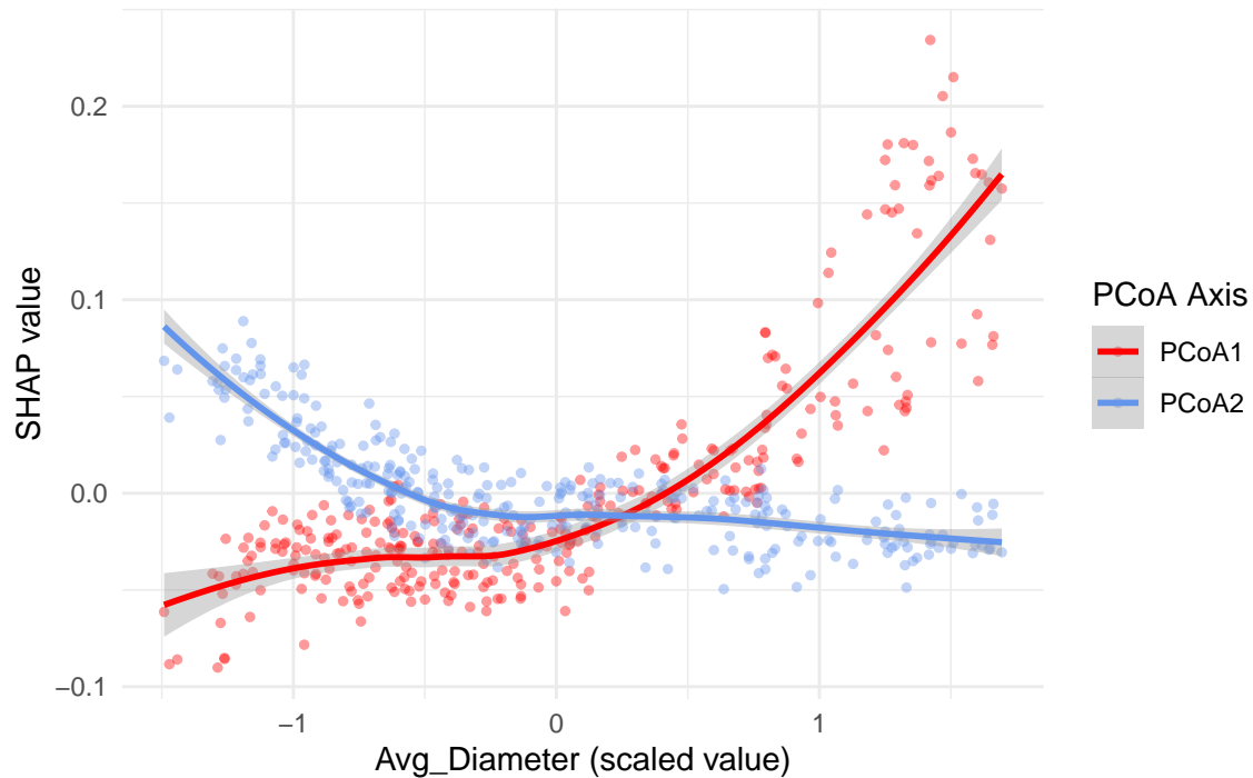
SHAP Values vs Scaled Avg_Diameter (Fungi)
