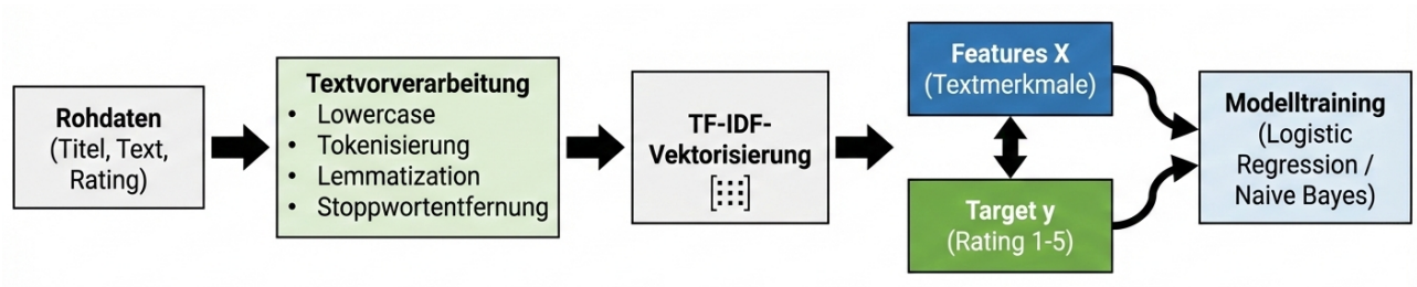
Abbildung 4.: Vorverarbeitungsprozess. Quelle: Gemini, Nano Banana Pro
