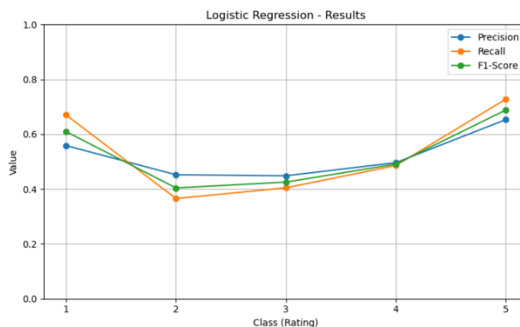
Abbildung 5.: Classification Report, Logistische Regression
