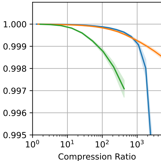
SSIM
