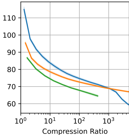
PSNR (dB)
