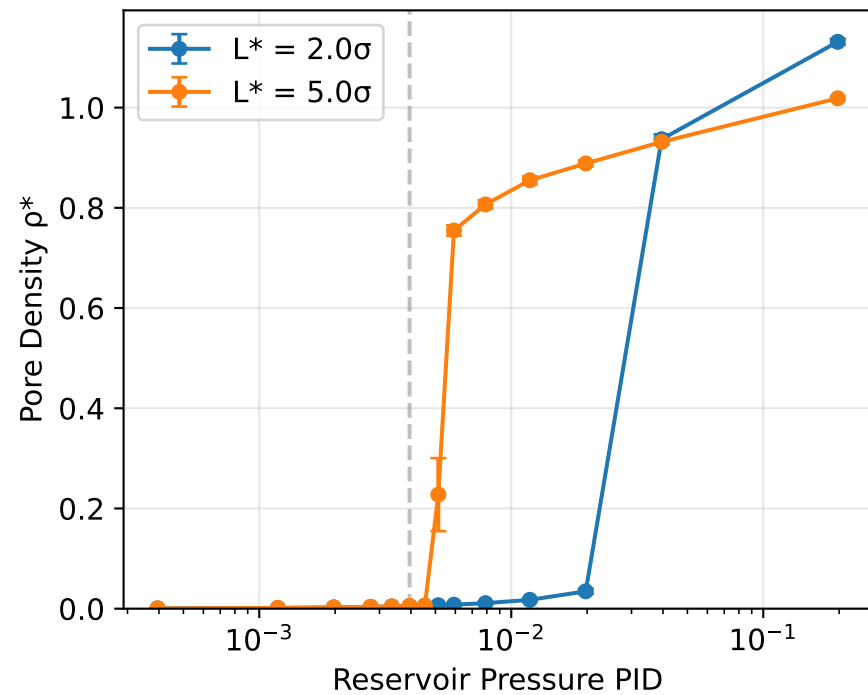
T^* = 0.8 (Subcritical)
