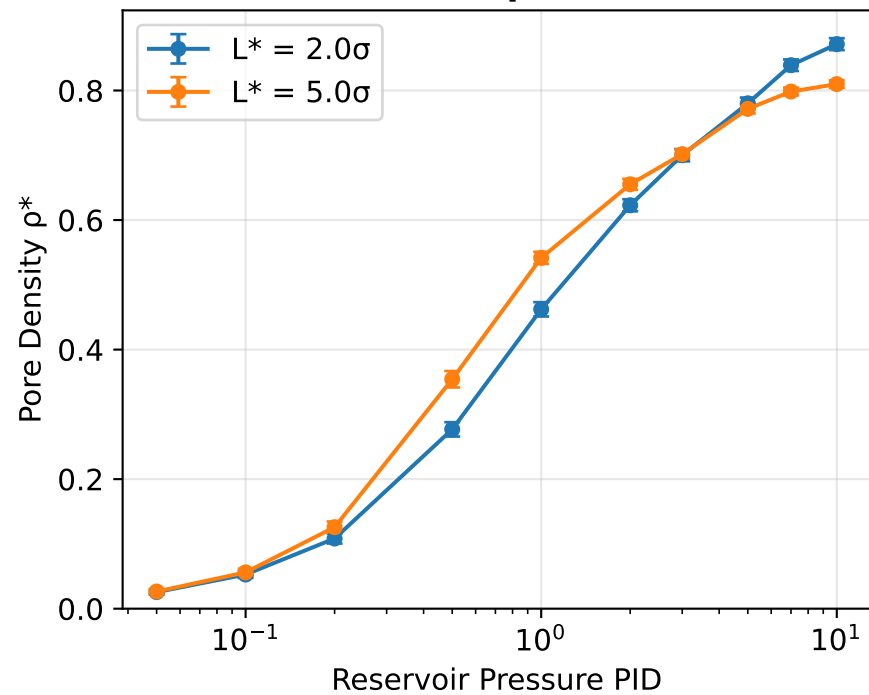
T^* = 2.0 (Supercritical)
