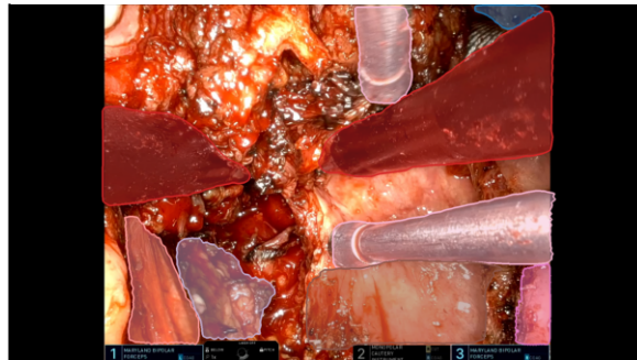
Mask R-CNN
