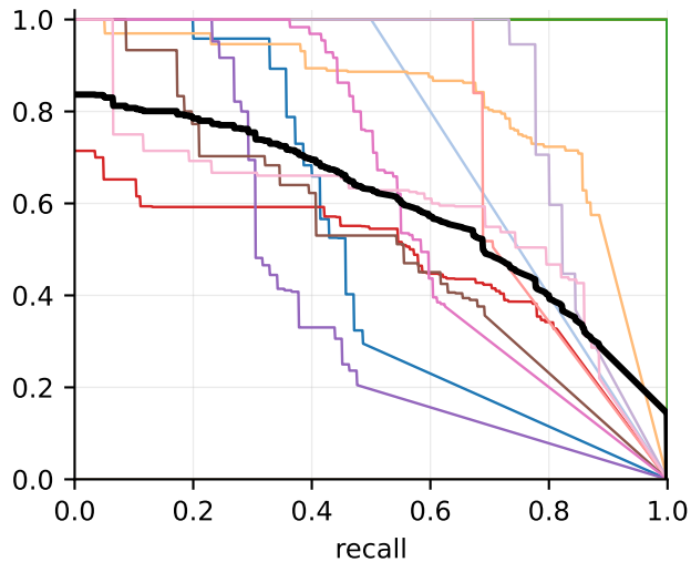
YOLO11n-seg mAP@0.5 = 0.543
