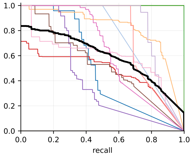
YOLO11n-seg mAP@0.5 = 0.543
