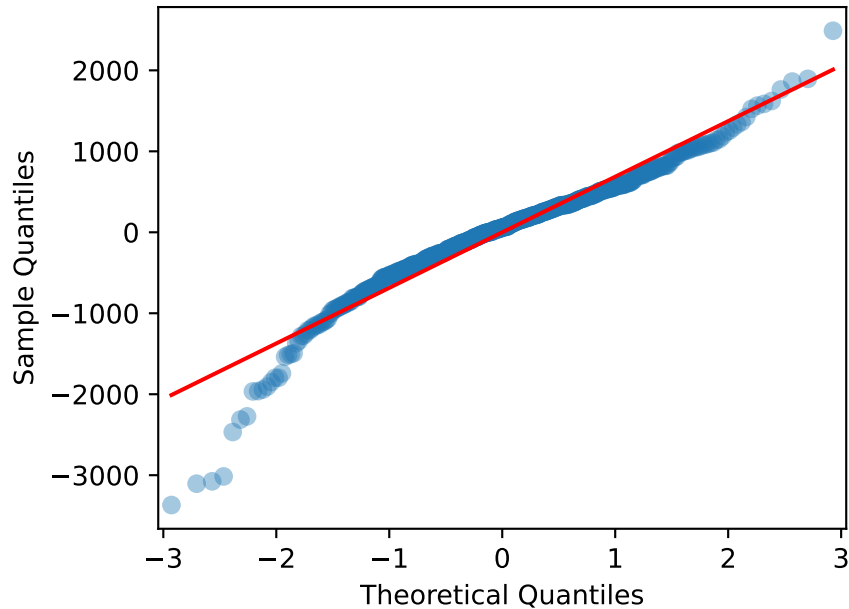
Normal Q-Q
